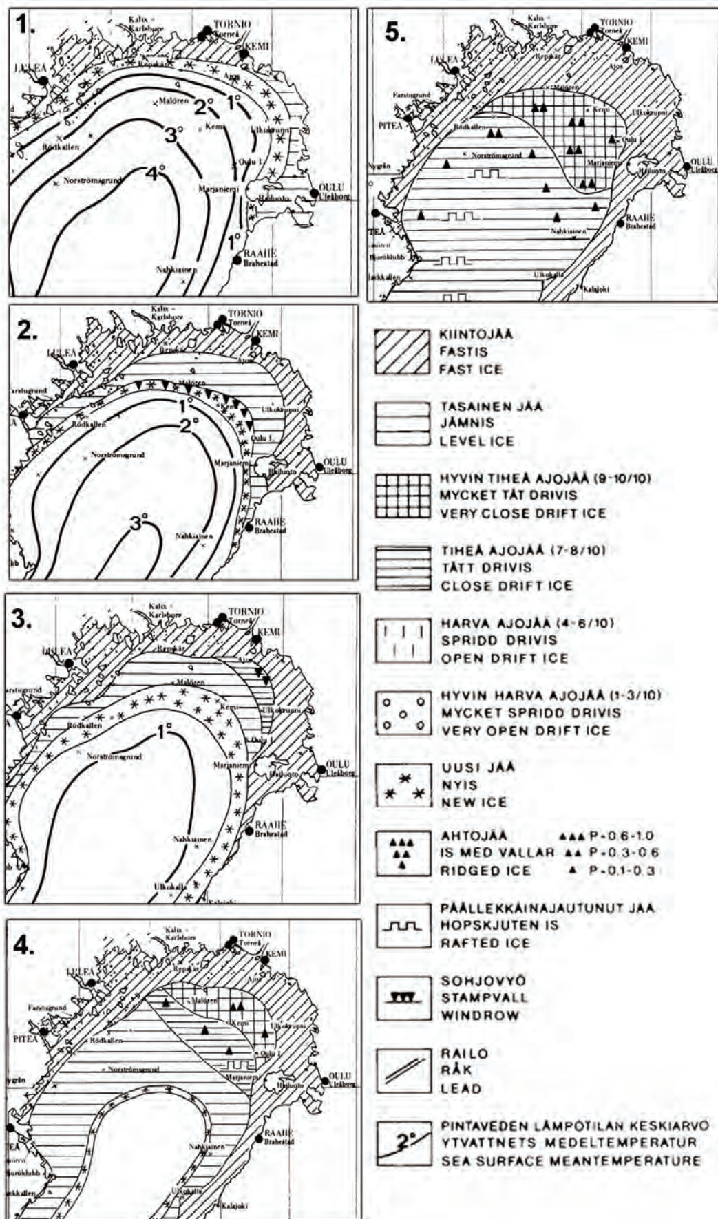
Kuva 17. Alkutilan jäävaiheet 1–5 Perämerellä (Leppäranta ym., 1988).
