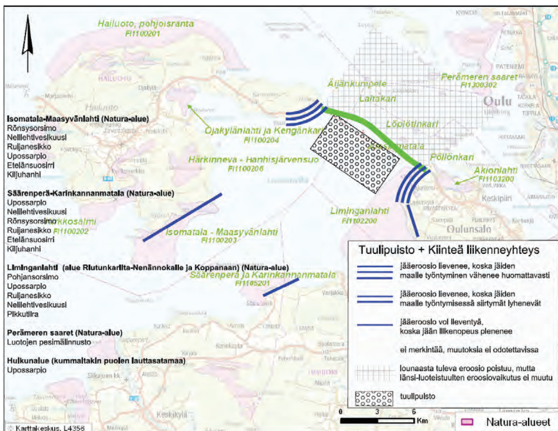
Kuva 20. Yhteenvedo jääeroosion muutoksista tuulipuiston ja kiinteän liikenneyhteyden toteutuksessa sekä muutosten kannalta merkittävimmät lajit.
