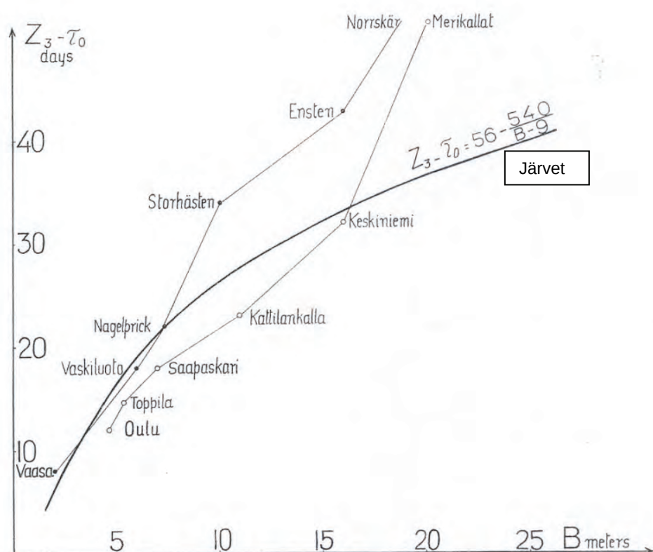
Kuva 6. Jäätymisen riippuvuus syvyydestä Oulun välillä (Oulu – Merikallat), vertaus myös Vaasan välillä (Vaasa – Norrskär) ja järviin. Pystyakselilla on aika (vrk) siitä kun ilman lämpötila on asettunut 0^{\circ}\text{C} alapuolelle, vaaka-akselilla syvyys (m).
