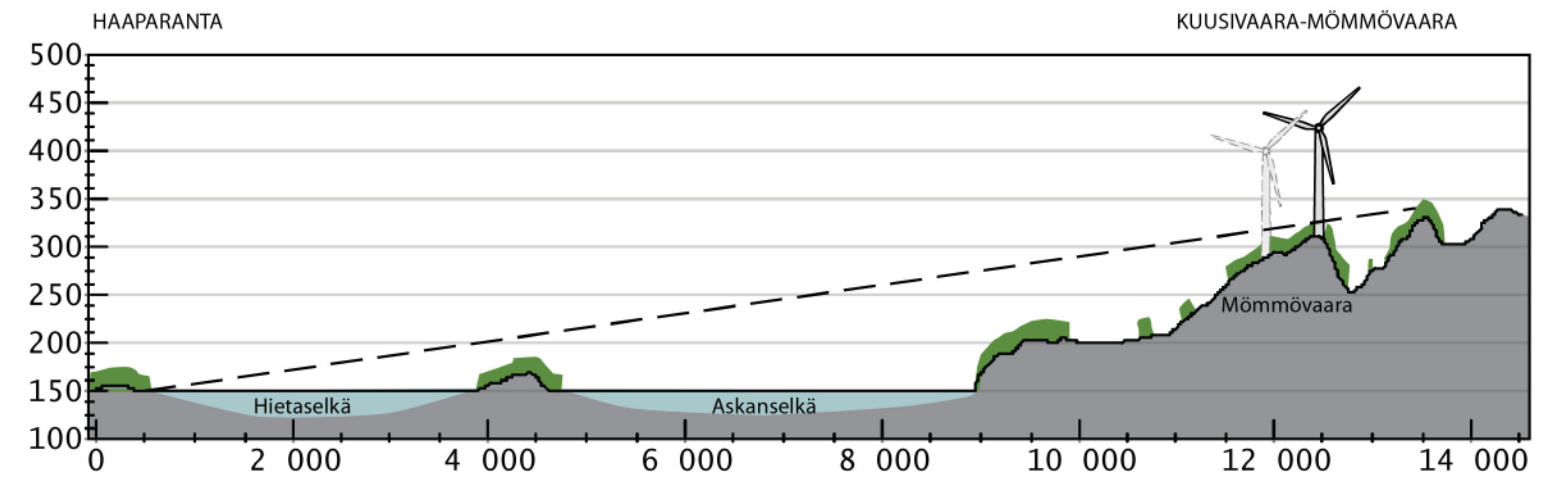
Kuva 100. Maastopoikkileikkaus Haaparannasta Kuusivaara-Mömmövaaralle. Tuulivoimalat näkyvät tarkastelupisteeseen Hietaselän ja Askanselän yli.
