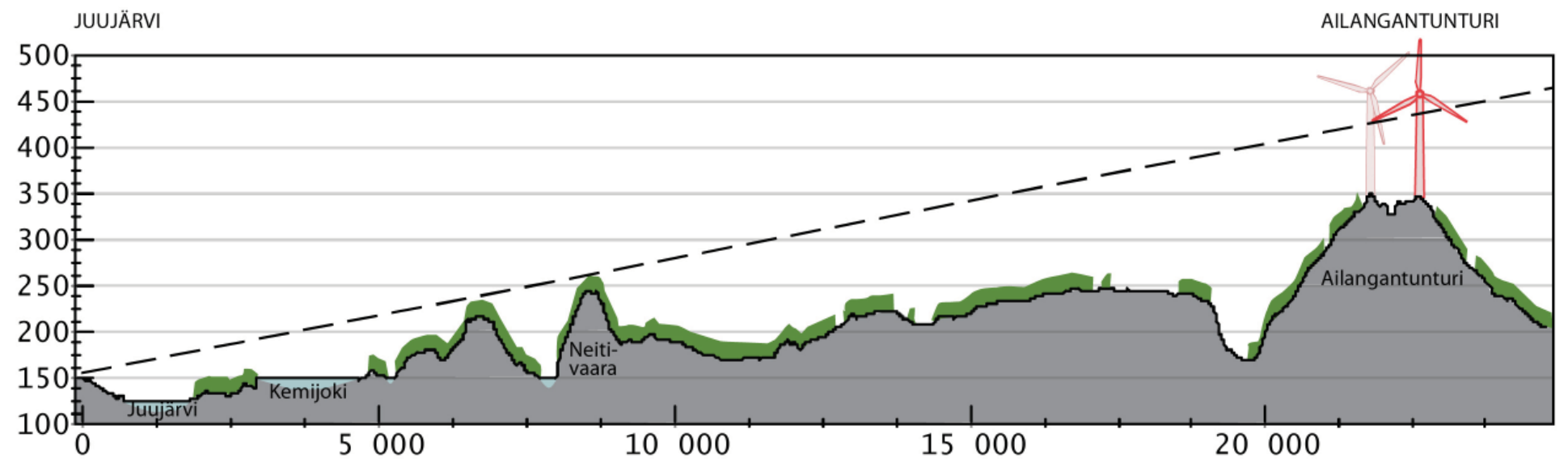
Kuva 122. Maastopoikkileikkaus Juujärven kylältä Ailangantunturin hankealueelle. Tuulivoimalat näkyvät esteettä, mutta etäisyyden ollessa noin 21-23 kilometriä, ne eivät enää hallitse maisemakuvaakaan vaan uppoavat pitkälti taustaan. Roottorin lapoja ei näy, mutta tornit erottuvat selkeällä säällä.
