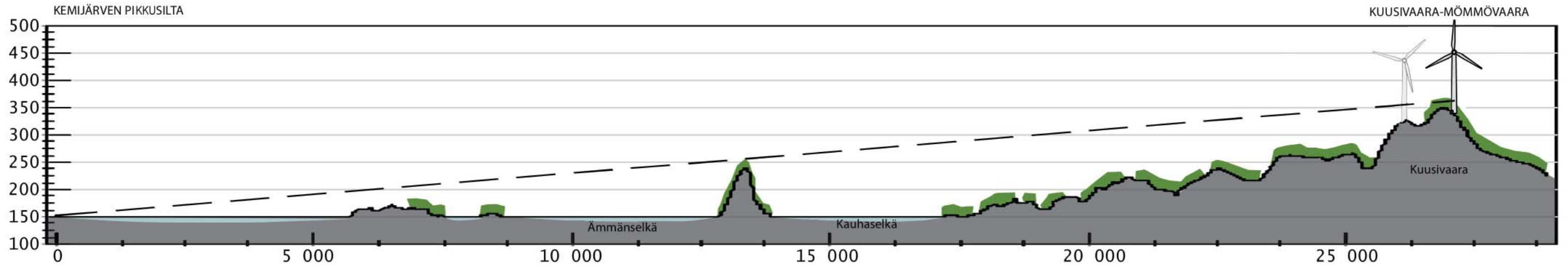
Kuva 107. Maastopoikkileikkaus Kemijärven pitkäsillalta
