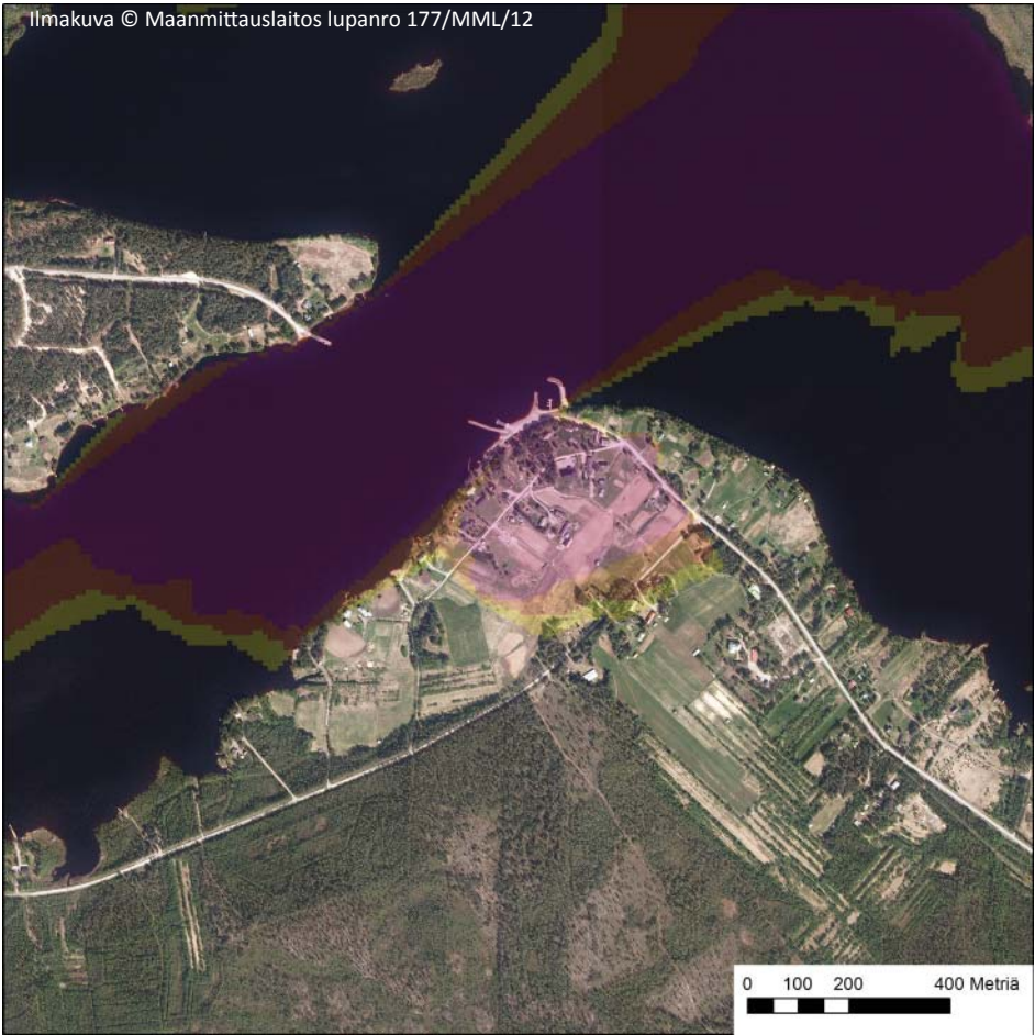
Tuulivoimalasta näkyy lapojen lisäksi osa tornia silmänkorkeudella (1,65 m)
