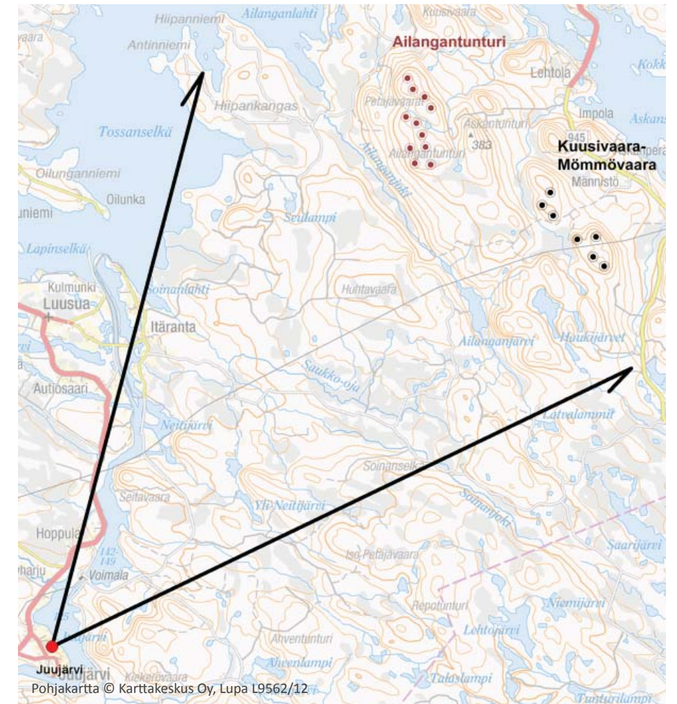
Kuva 123. Seuraavan sivun (sivu 74) havainnekuvien kuvanottopiste ja kuvasektori.
