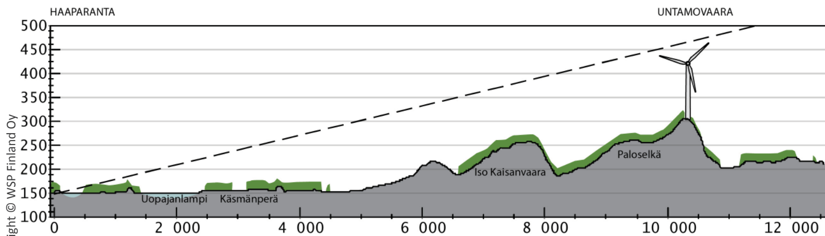
Kuva 98. Maastopoikkileikkaus Haaparannasta Untamovaaralle. Tuulivoimalat eivät näy tarkastelupisteeseen, koska metsä estää näkyvyyden. Näkymä-alueanalyysin mukaan kylällä, sekä Räisälässä että Haaparannassa on aluieta, joihin näkyy Untamovaaran voimaloita.
