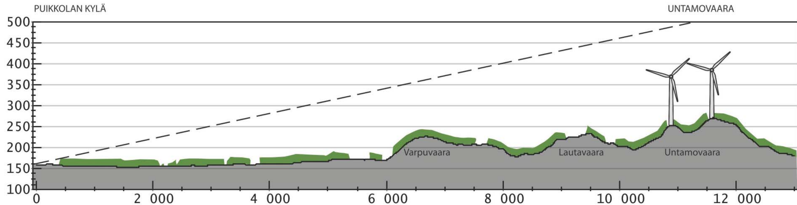
Kuva 68. Maastopoikkileikkaus Puikkolan kylältä Untamovaaralle. Metsä estää tuulivoimaloiden näkymisen tarkastelupisteeseen.
