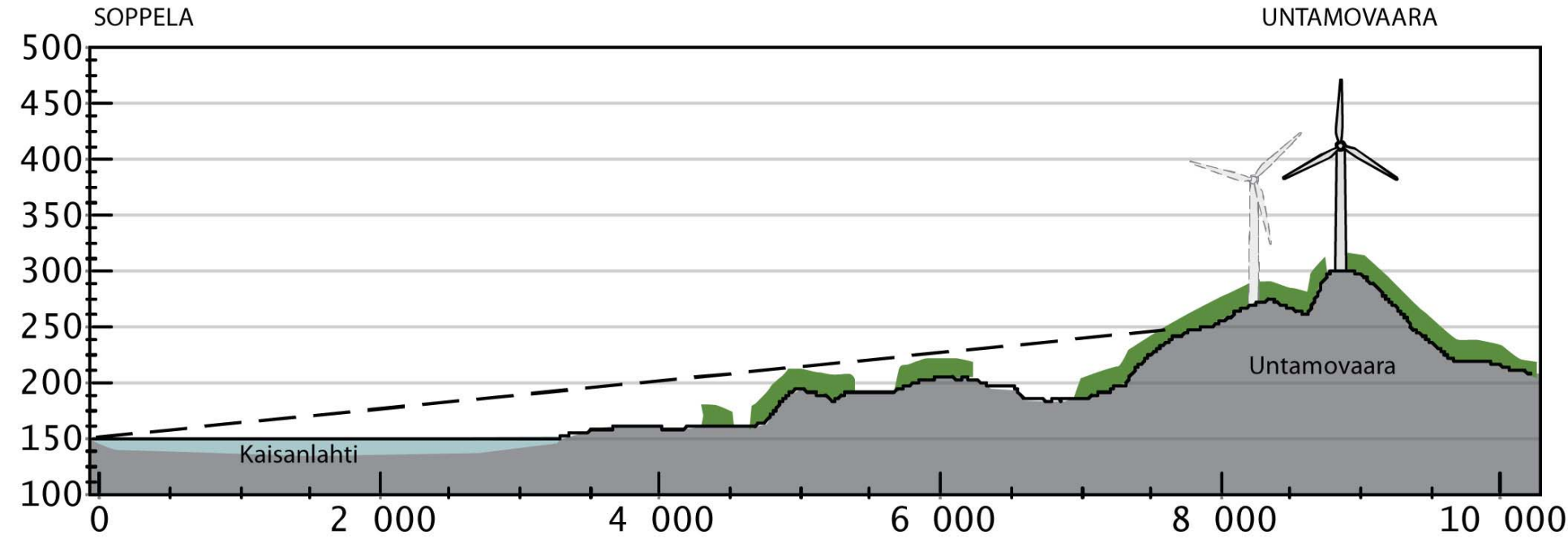
Kuva 74. Maastopoikkileikkaus Soppelan pengertieltä Untamovaaralle. Tuulivoimalat näkyvät esteettä tarkastelupisteeseen ja järvelle.
