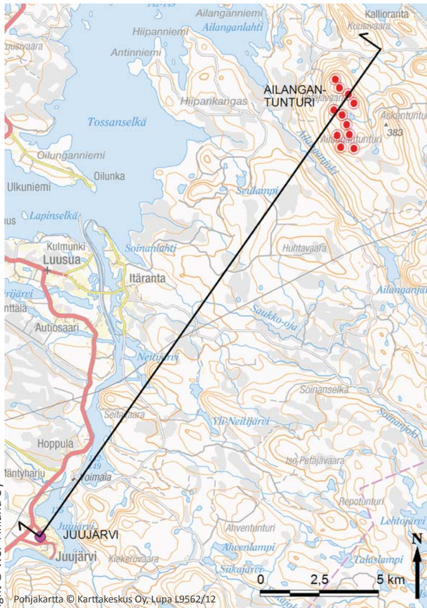
Kuva 121. Viereisen (kuva 122) maastopoikkileikkauksen leikkauskohta.
