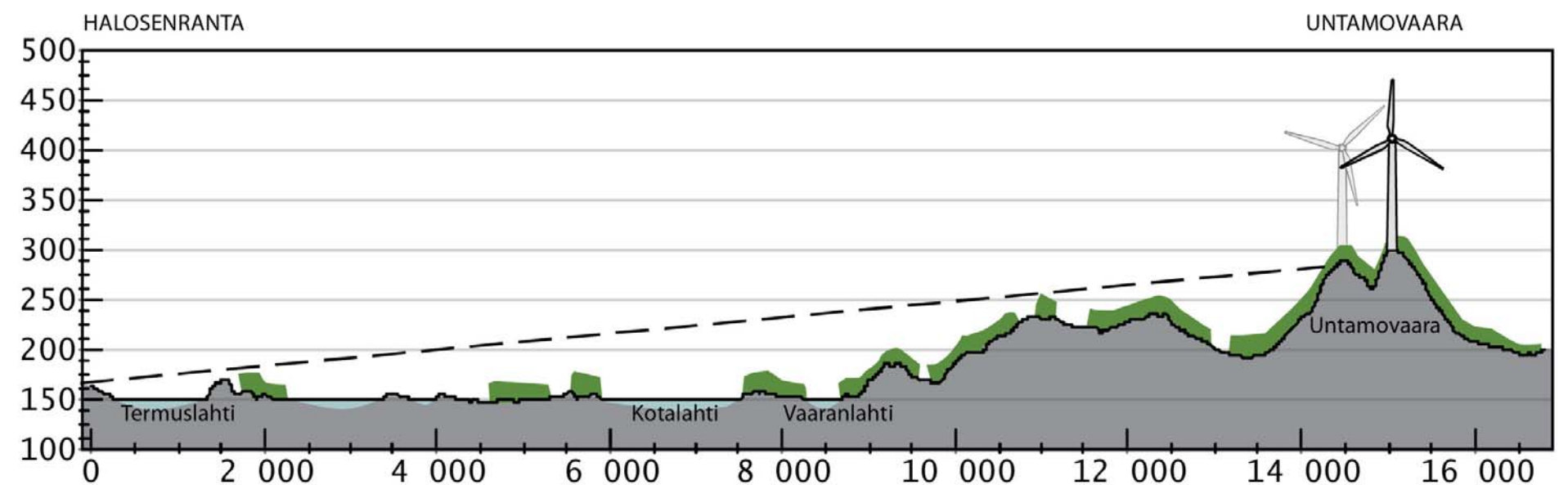
Kuva 114. Maastopoikkileikkaus Halosenrannan kylältä Untamovaaran hankealueelle. Tuulivoimalat näkyvät esteettä, mutta etäisyyden ollessa noin 14–16 kilometriä, ne eivät enää hallitse maisemakuvaa vaan uppoavat pitkälti taustaan. Roottorin lapoja ei näy, mutta tornit erottuvat selkeällä säällä.
