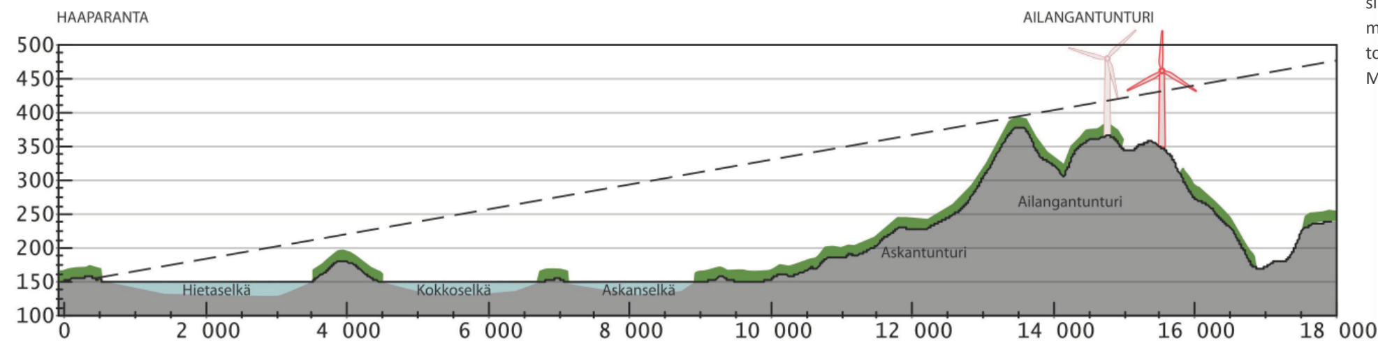
Kuva 102. Maastopoikkileikkaus Haaparannasta Ailangantunturille. Ailangantunturin tuulivoimalat näkyvät sekä Räisälään että Haaparantaan.
