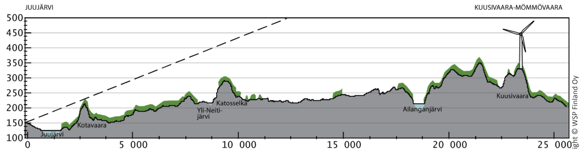
Kuva 120. Maastopoikkileikkaus Juujärven kylältä Untamovaaran hankealueelle. Tuulivoimalat eivät näy tarkastelupisteeseen. Näkyvyyden estävät maastonmuodot ja kasvillisuus. Toisaalta, koska etäisyyttä hankealueelle on 22-24 kilometriä, tuulivoimalat uppoavat maisemaan. Vain tornit näkyvät ihanteellisissa olosuhteissa.
