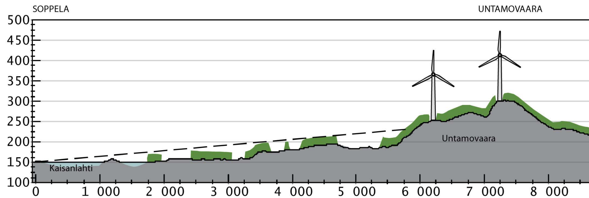
Kuva 81. Maastopoikkileikkaus Soppelan kylältä Untamovaaralle. Tuulivoimalat näkyvät esteettä tarkastelupisteeseen ja järvelle.
