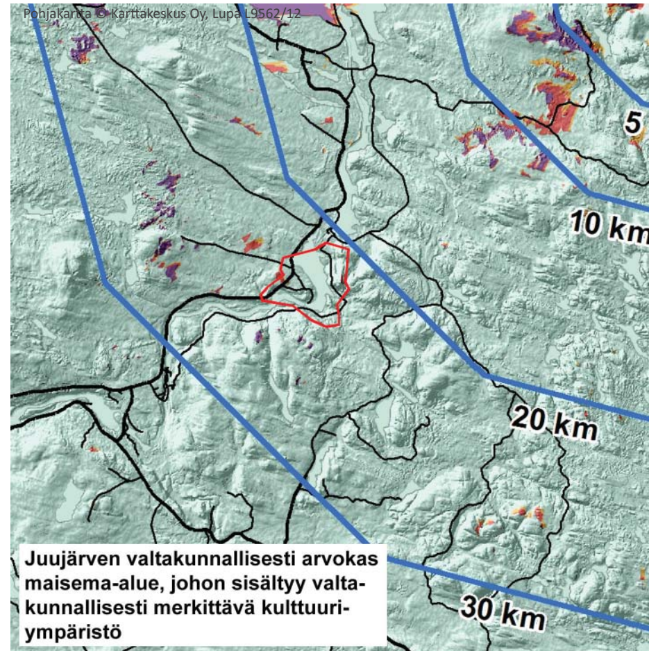
Kuva 118. Suurennos näkymäalueanalyysistä, VE 3. Maisema-alueen, joka on rajattu kuvassa punaisella, länsireunassa on pieni alue, johon näkyy 1-4 Kuusivaara-Mömmövaaran voimalaa.
