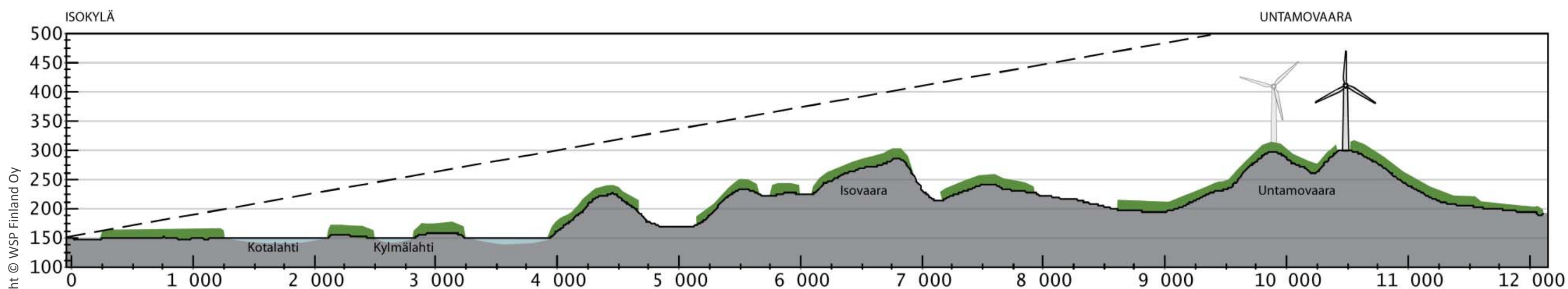
Kuva 90. Maastopoikkileikkaus Isokylän kohdalta Untamovaaralle. Tuulivoimalat eivät näy tarkastelupisteeseen, koska metsä estää näkyvyyden.
