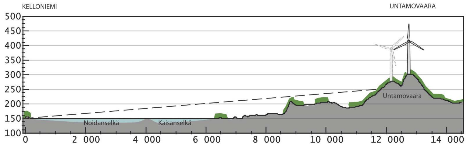
Kuva 117. Maastopoikkileikkaus Kelloniemestä Untamovaaran hankealueelle. Tuulivoimalat näkyvät rannan tarkastelupisteeseen esteettä, mutta etäisyyden ollessa noin 12-13 kilometriä ne eivät enää hallitse maisemakuvaa vaan uppoavat pitkälti taustaan. Roottorin lavat saattavat erottua suotuisissa sää- ja valo-olosuhteissa.
