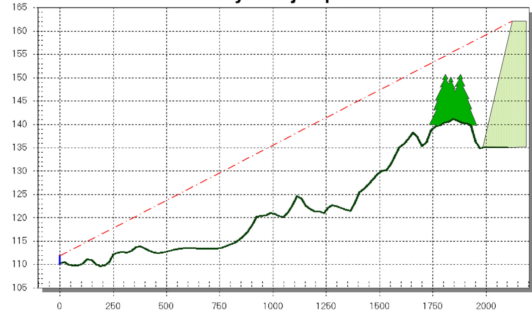
Näkymälinja Np6
