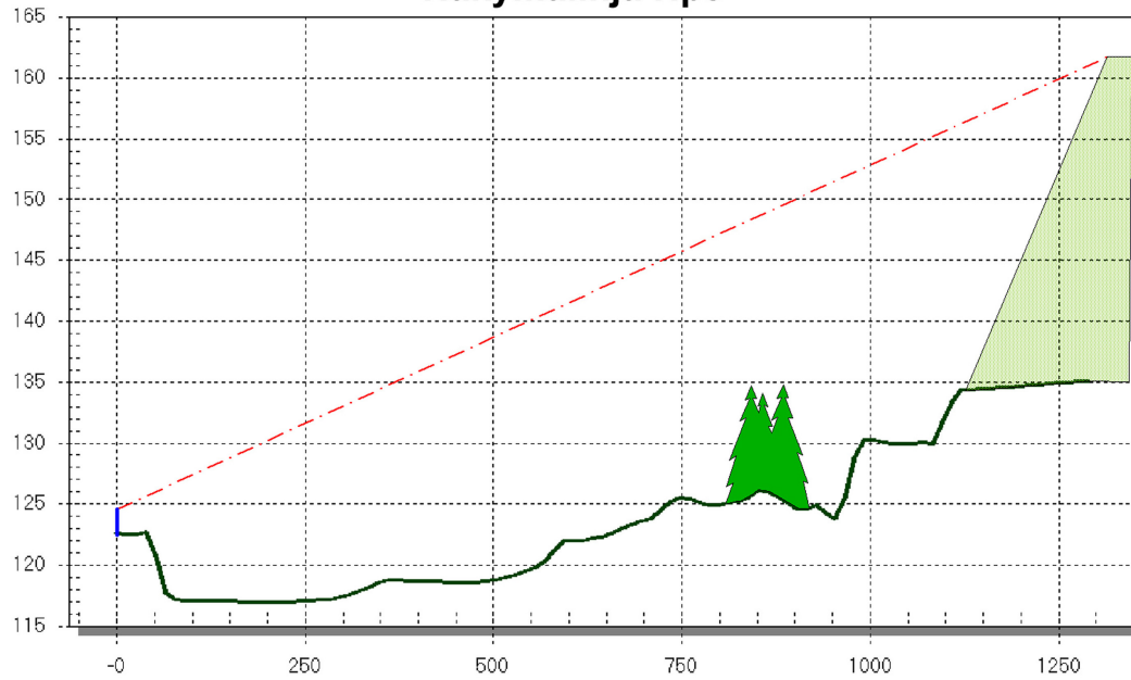
Näkymälinja Np7
