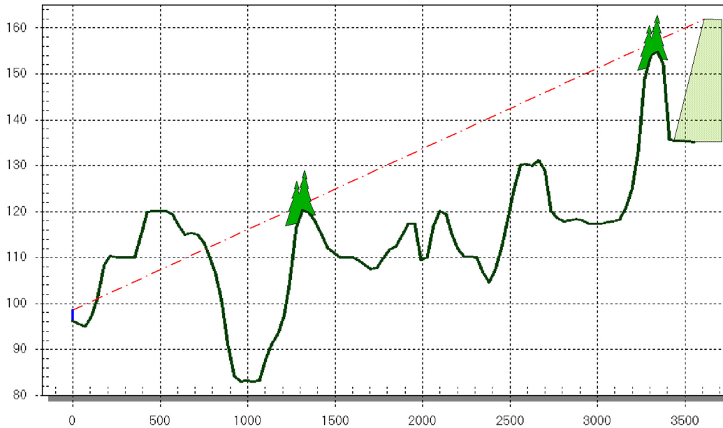
Näkymälinja Np7
