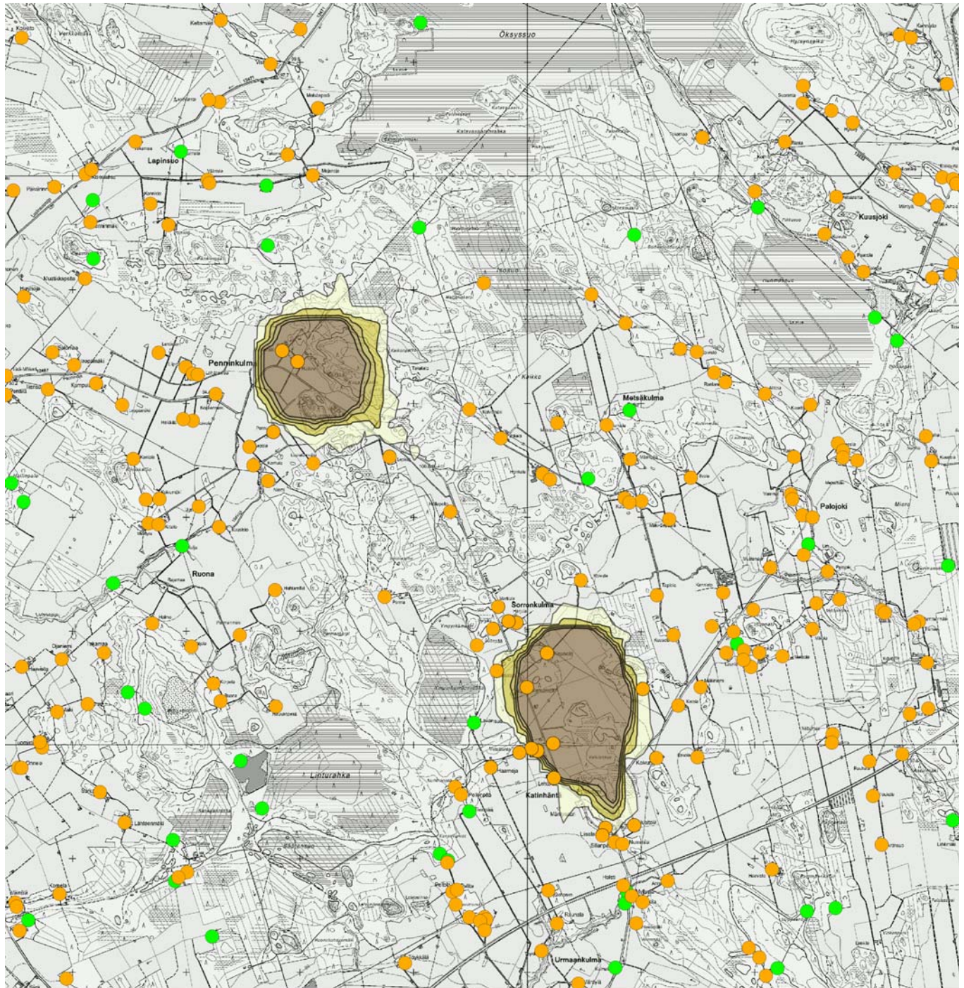
Liitekuva 25. Vaihtoehto VE3, hajutuntien (pitkäaikainen haju) osuus vuodessa, melko voimakas, tunnistettava haju (5 HY/m 3 ). Asuinrakennukset on merkitty oransseilla palloilla ja lomarakennukset vihreillä palloilla.
