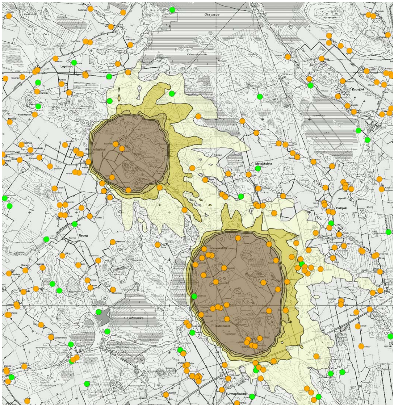
Liitekuva 23. Vaihtoehto VE3, hajutuntien (pitkäaikainen haju) osuus vuodessa, juuri havaittava haju (1 HY/m 3 ). Asuinrakennukset on merkitty oransseilla palloilla ja lomarakennukset vihreillä palloilla.
