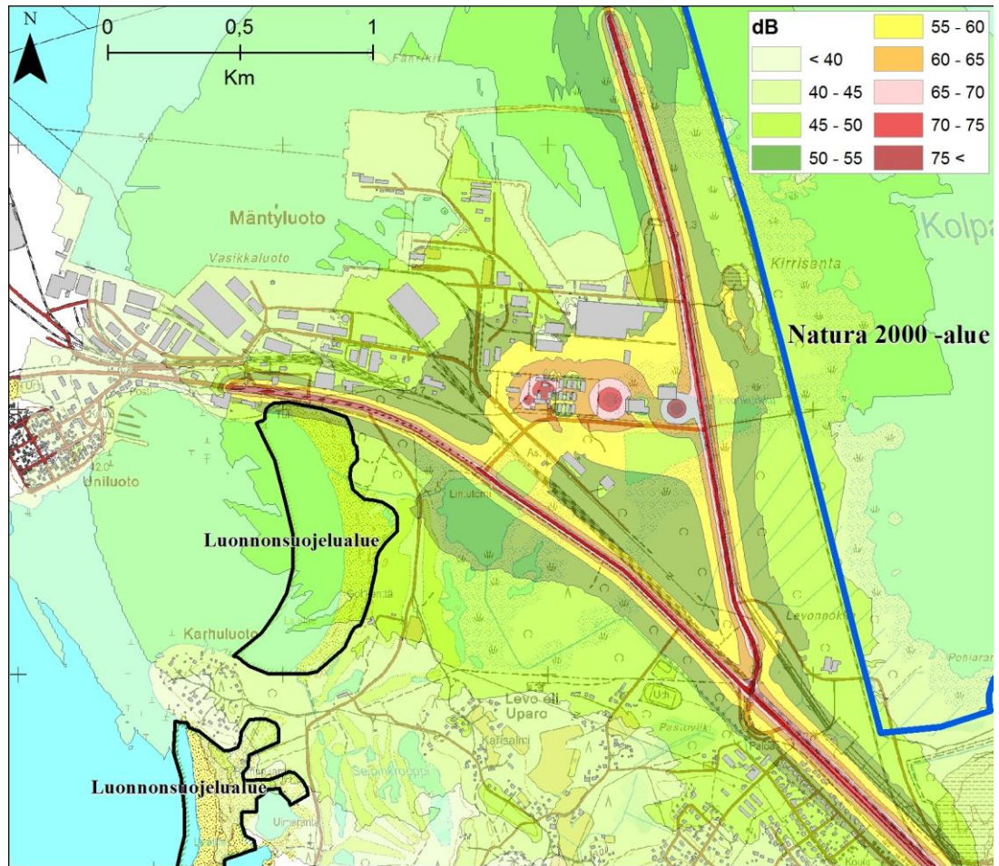
Kuva 14. Ekokemin teollisuusjätekeskuksen laajennuksen melumallinnus. Melutasot kuvastavat maksimitilannetta (Ecobio 2014).
