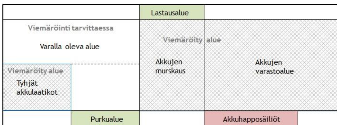
Kuva 2. Suunnitellun akkuterminaalin pohjapiirros. Akkujen käsittelyalueet on viemäroity umpikaivoihin, joista akkuhapot ohjataan asianmukaisesti maanpäällisiin akkuhapposäiliöihin.
