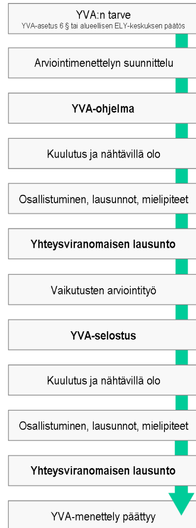
Kuva 10. YVA-prosessin eteneminen.
