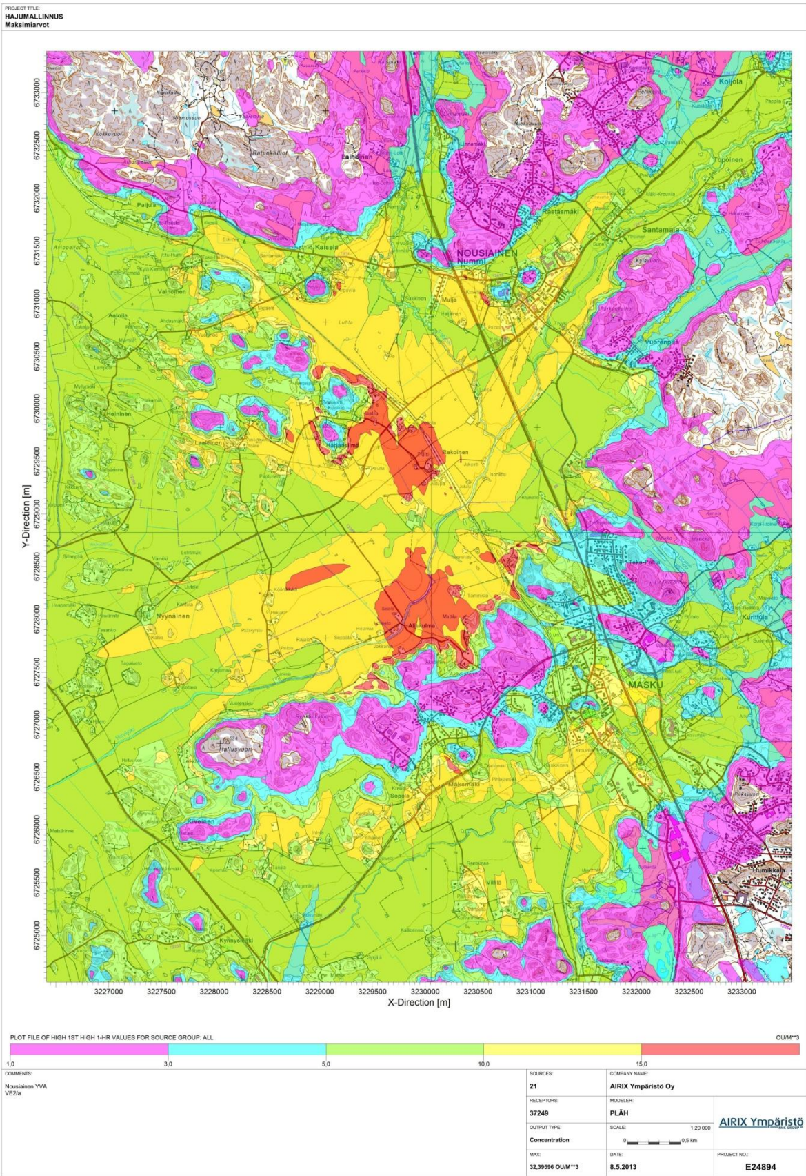
Kuva 12 Vaihtoehto VE2/a Maksimi-arvot, yhden tunnin hajua
