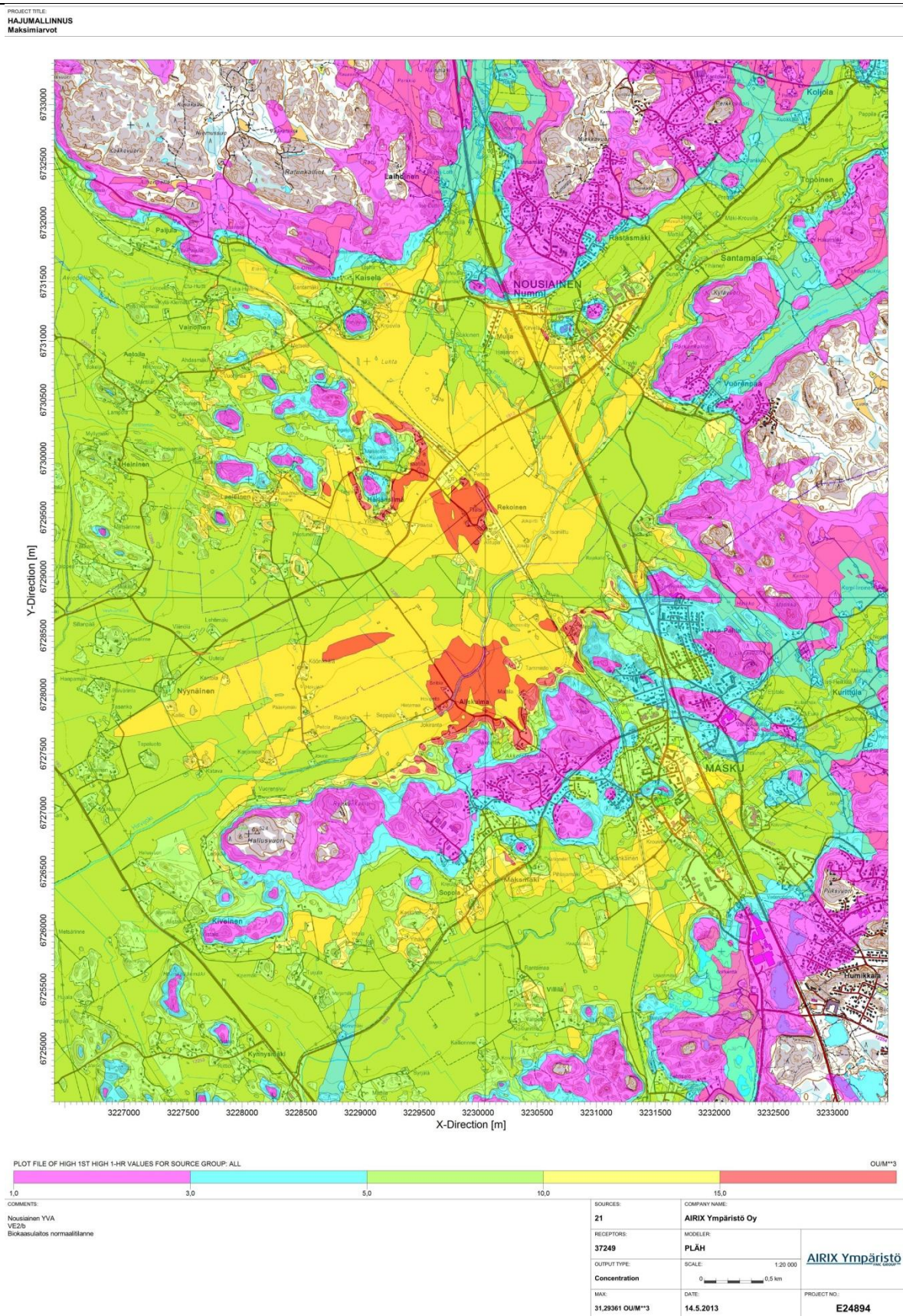
Kuva 13 Vaihtoehto VE2/b, biokaasulaitos normaalitilanne Maksimi-arvot, yhden tunnin hajuu
