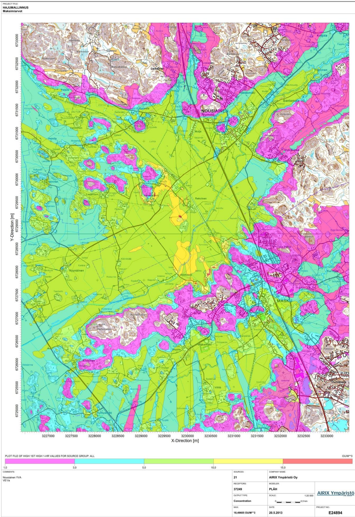
Kuva 9 Vaihtoehto VE1/a Maksimi-arvot, yhden tunnin hajua
