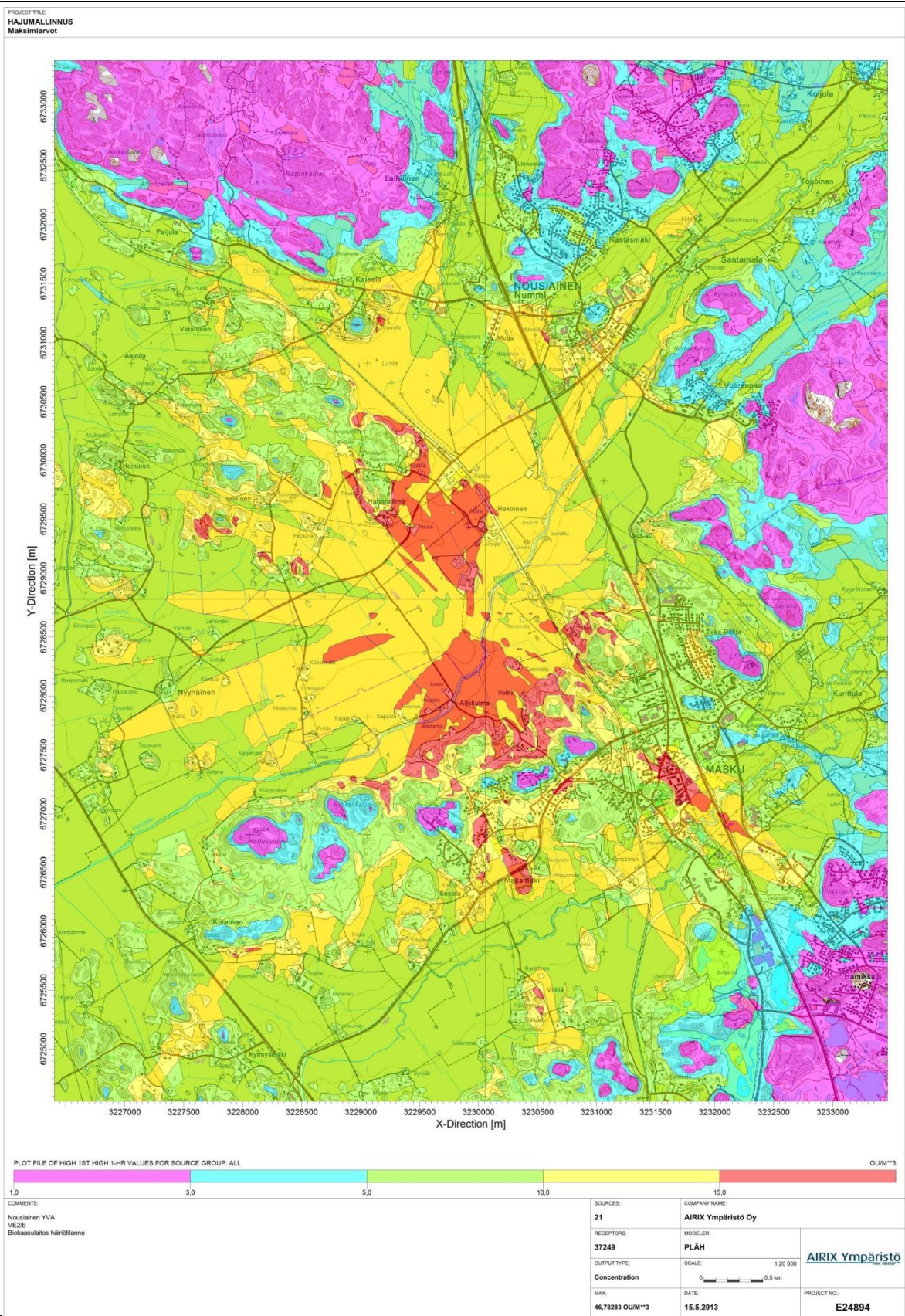
Kuva 14 Vaihtoehto VE2/b, biokaasulaitos häiriötilanne Maksimi-arvot, yhden tunnin haju
