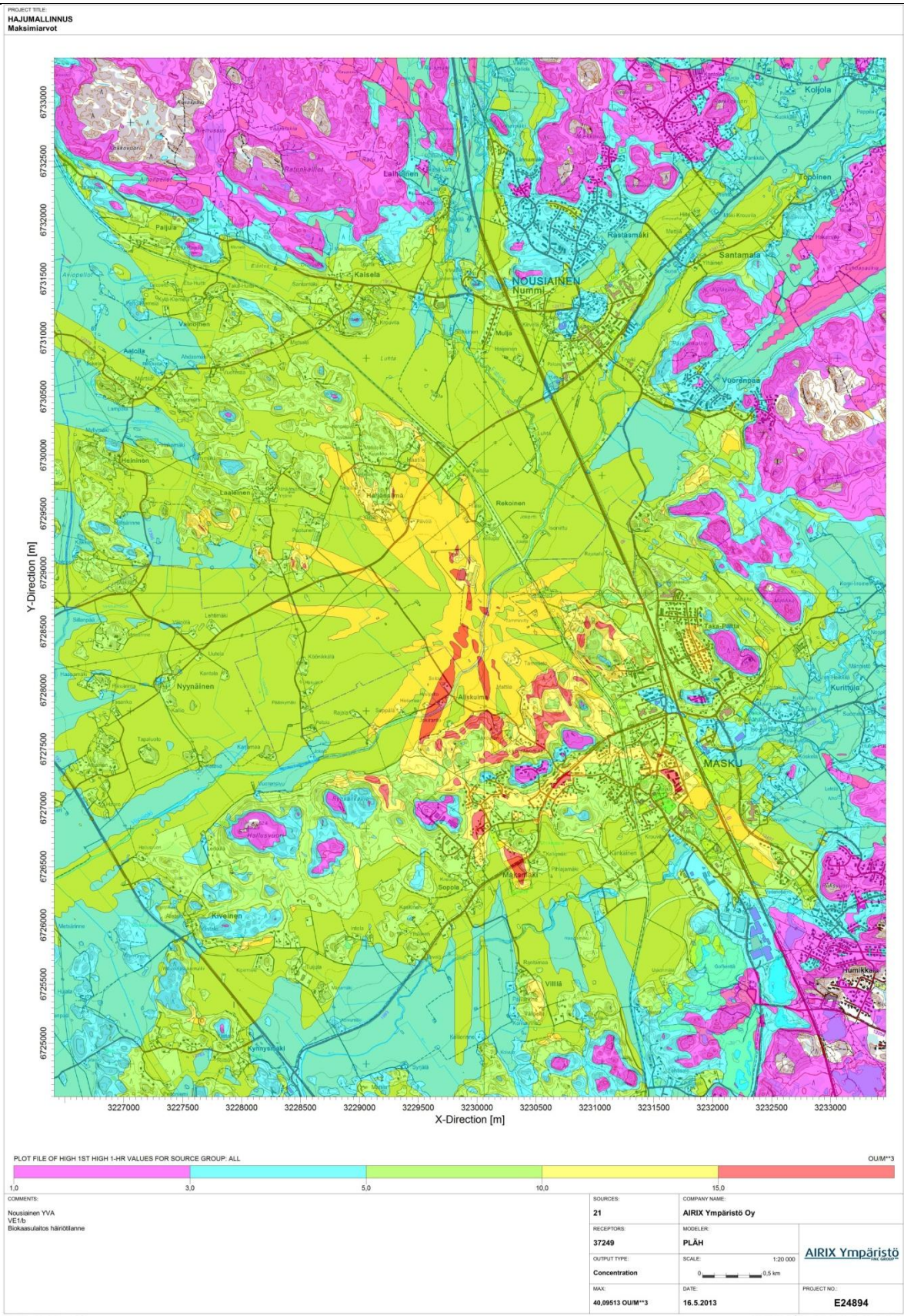
Kuva 11 Vaihtoehto VE1/b, biokaasulaitos häiriötilanne Maksimi-arvot, yhden tunnin hajua
