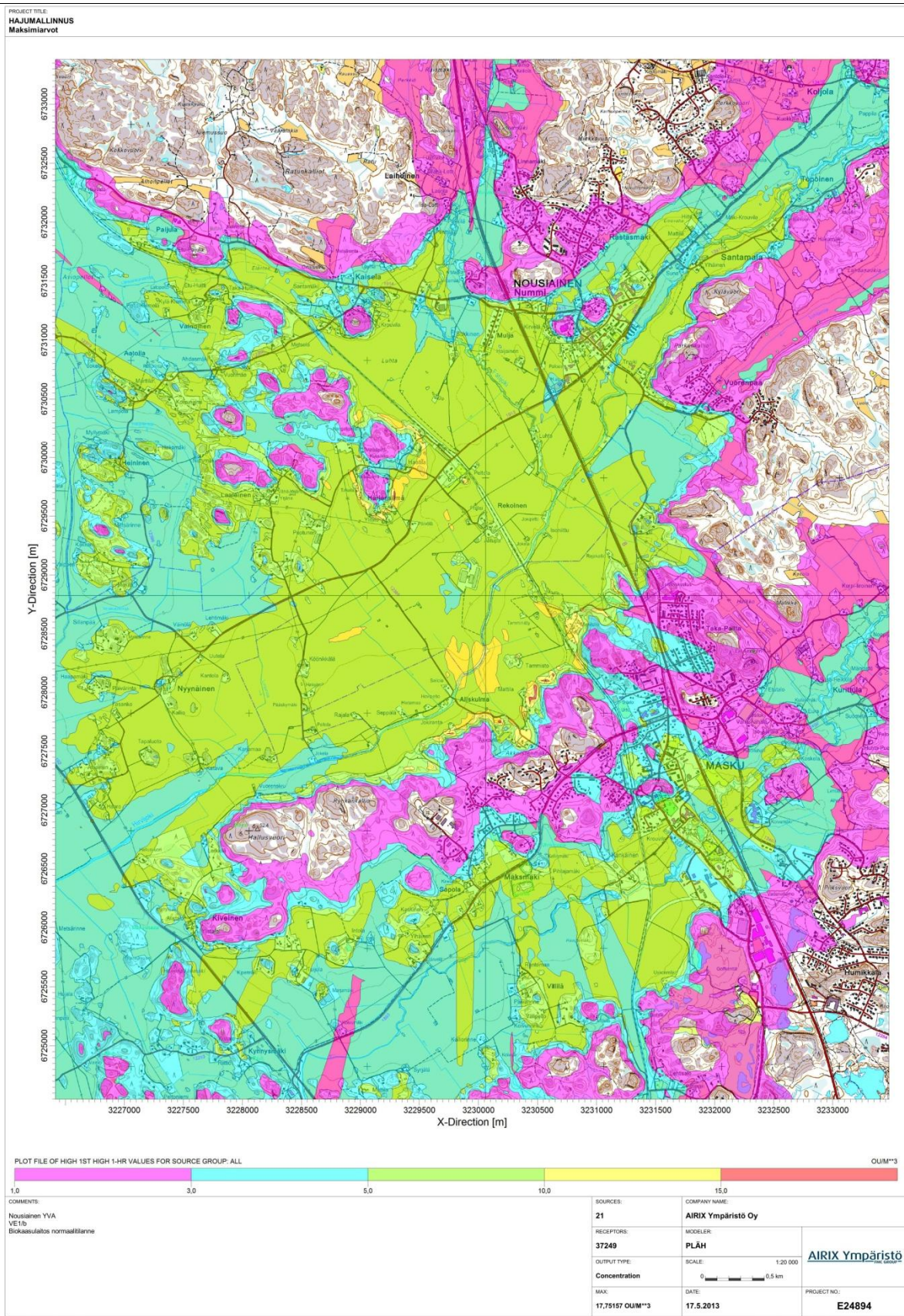
Kuva 10 Vaihtoehto VE1/b, biokaasulaitos normaalitilanne Maksimi-arvot, yhden tunnin hajua
