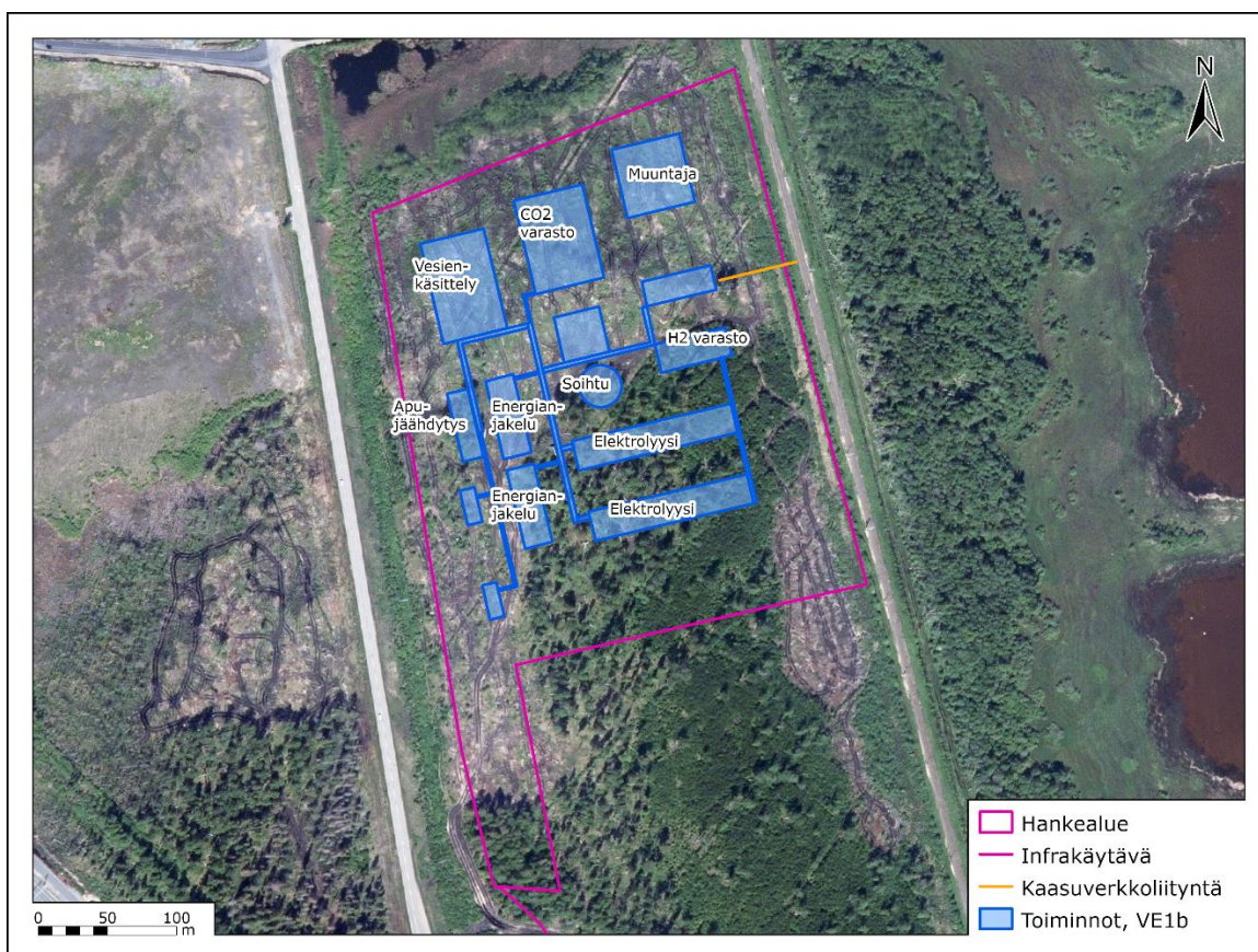
Kuva 3-2. Hankealueen ja laitostoimintojen sijainti Porin Kirrinsannan teollisuusalueella vaihtoehdossa VE1b. Taustana Maanmittauslaitoksen ortokuva.
