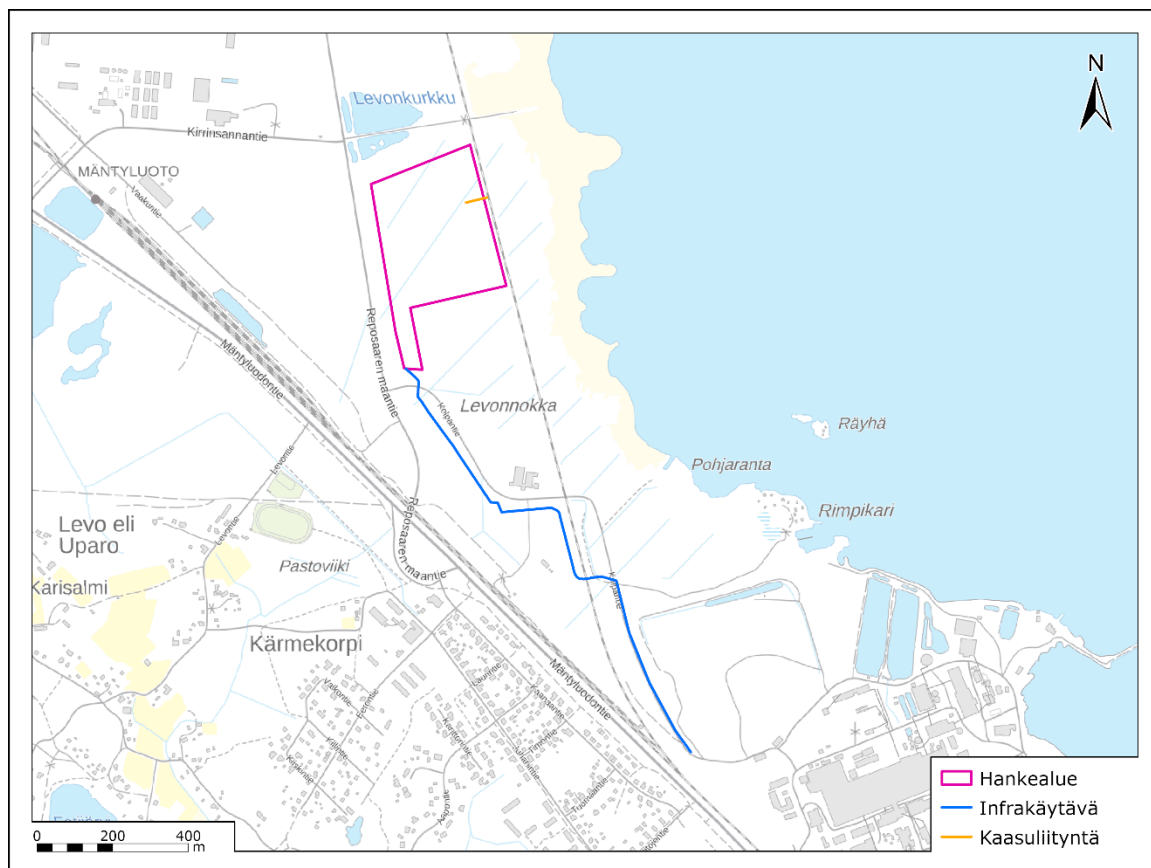
Kuva 3-3. Suunniteltu infrakäytävä Kaanaaseen. Maanalaisessa infrakäytävässä kulkevat kaukolämpölinjat, mahdolliset puhdas- ja jätevesilinjat sekä CO 2 -siirtoputki. Kaasuliityntä metaanikaasulle tehdään hankealueen itäreunassa sijaitsevaan kaasuverkkoon.
