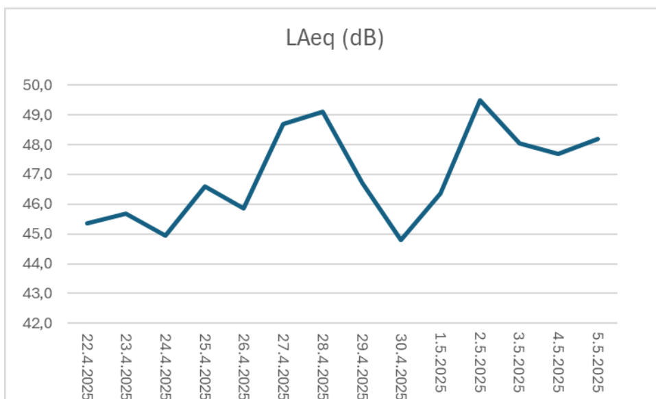
Kuva 11-3. Päiväajan nykytilan keskiäänitaso LAeq Natura-alueella.
