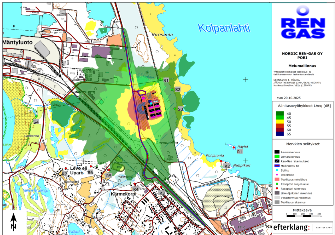
Kuva 11-11. Hankevaihtoehtoon VE1a meluvyöhykkeet skenaariotilanteen aikana 22–07. P2G-laitos on toiminnassa 24 tuntia vuorokaudessa.
