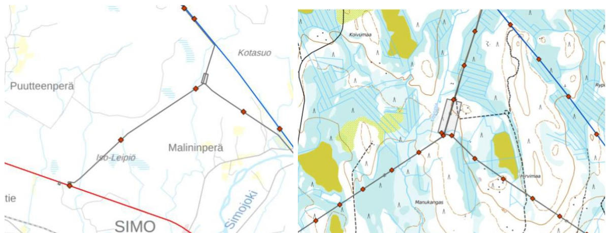
Kuva 16. Suunnitellun Sijojen sähköaseman alustava sijoitussuunnitelma (Fingrid Oyj 06/2019).
