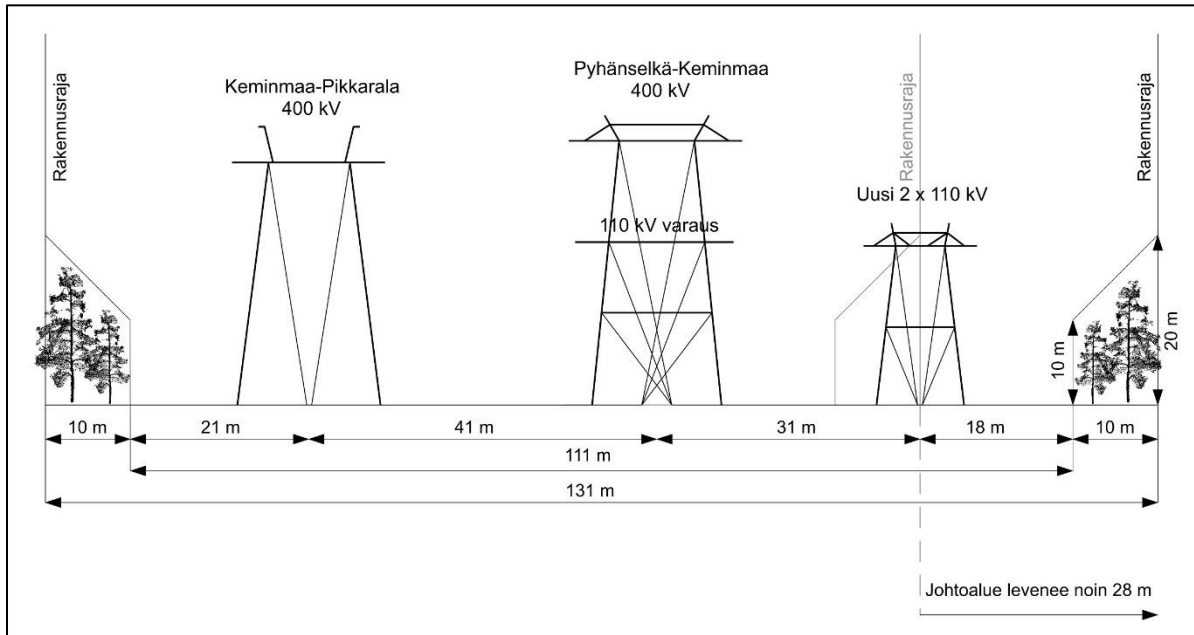
Kuva 18. Periaatepoikkileikkauskuva voimajohtoalueesta hankevaihtoehdossa SVE B. Fingridin suunniteltu uusi Pyhänselkä-Keminmaa 400+100 kV voimajohto nykyisen Keminmaa-Pikkarala 400 kV voimajohdon rinnalla. Yli-Olhavan 110 kV voimajohto sijoittuisi uuden 400 kV pylvään rinnalle (kuvan tilanne). Kuvassa esitetty kaksivirtapiirinen johto-osuus A-B-C.
