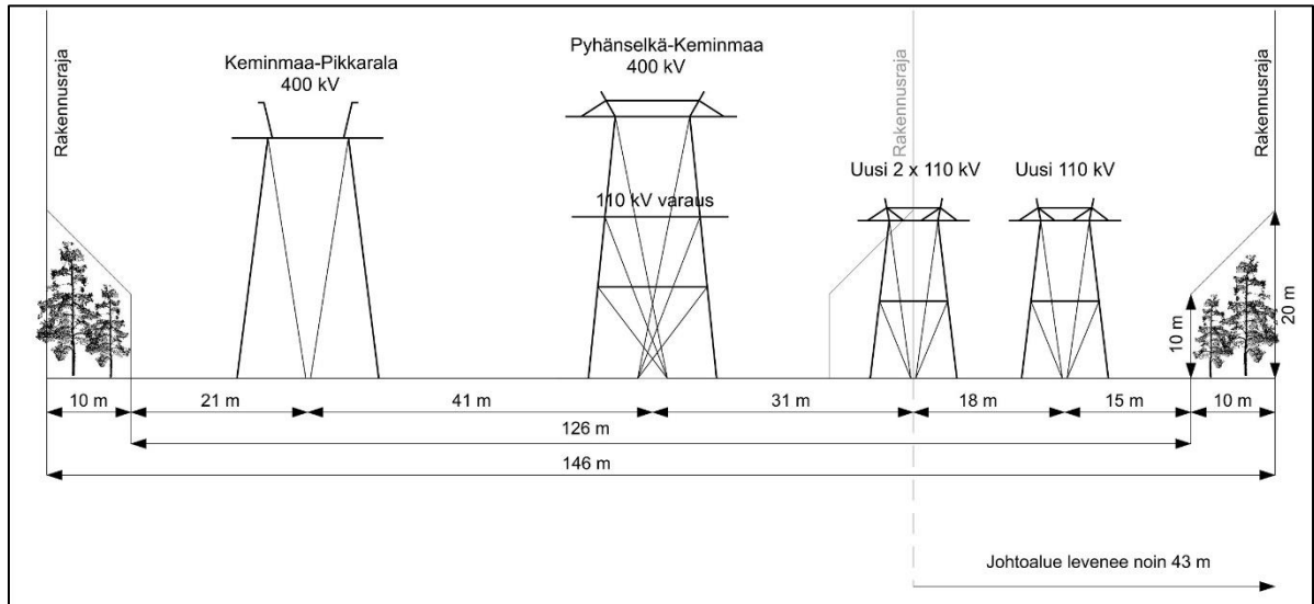
Kuva 20. Periaatepoikkileikkauskuva voimajohtoalueesta hankevaihtoehdossa SVE E. Fingridin suunniteltu uusi Pyhänselkä-Keminmaa 400+100 kV voimajohto nykyisen Keminmaa-Pikkarala 400 kV voimajohdon rinnalla. Yli-Olhavan 110 kV voimajohto sijoittuisi uuden 400 kV pylvään rinnalle (kuvan tilanne). Kuvassa esitetty johto-osuus D- Hervan sähköasema, kun tuulivoimapuiston kokonaisteho on yli 500 MW ja tarvitaan kaksi rinnakkaista 110 kV:n voimajohtoa.
