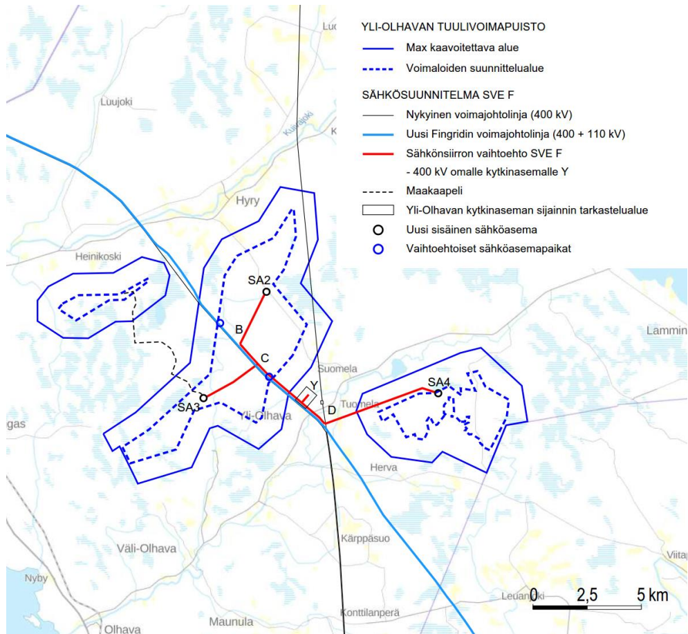
Kuva 14. Yli-Olhavan tuulivoimapuiston sähkönsiirtovaihtoehto SVE F.
