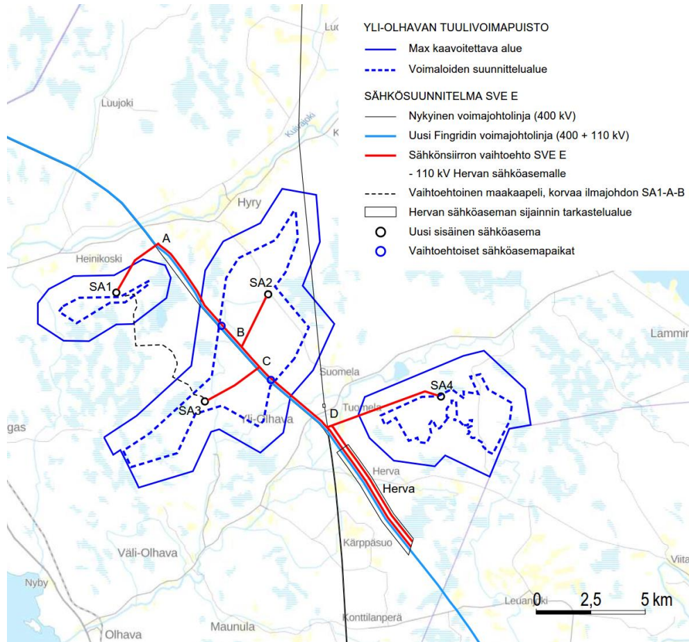
Kuva 13. Yli-Olhavan tuulivoimapuiston sähkönsiirtovaihtoehto SVE E.
