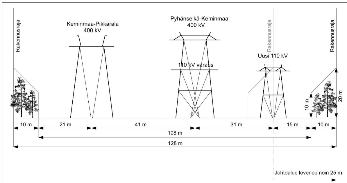
Kuva 19. Periaatepoikkileikkauskuva voimajohtoalueesta hankevaihtoehdossa SVE B. Fingridin suunniteltu uusi Pyhänselkä-Keminmaa 400+100 kV voimajohto nykyisen Keminmaa-Pikkarala 400 kV voimajohdon rinnalla. Yli-Olhavan 110 kV voimajohto sijoittuisi uuden 400 kV pylvään rinnalle (kuvan tilanne). Kuvassa esitetty yksivirtapiirinen johto-osuus C-D.
