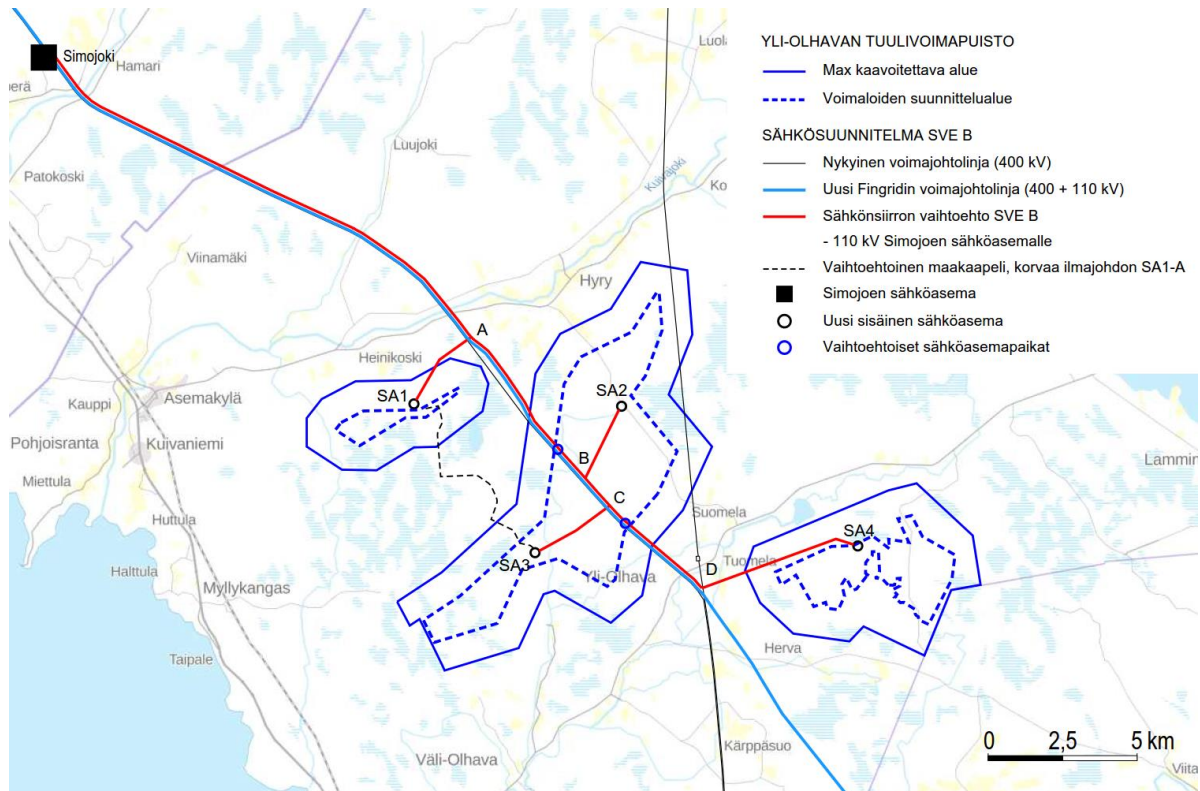
Kuva 12. Yli-Olhavan tuulivoimapuiston sähkönsiirtovaihtoehto SVE B.
