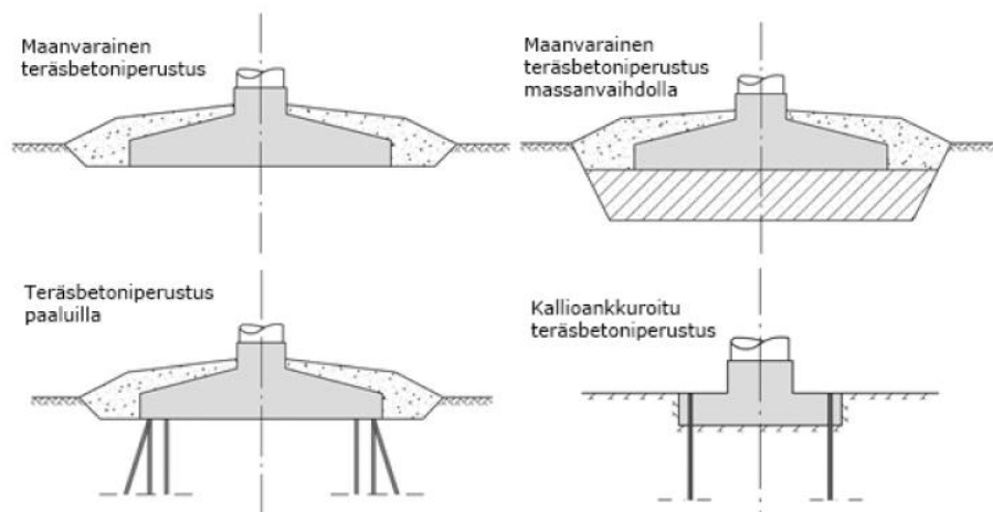
Kuva 8. Tuulivoimalaitosten perustamistekniikoita.
