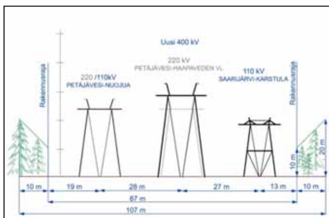
Kuva 29. Poikkileikkaus 2A e-f (Löytänä–Oinoskylä).
