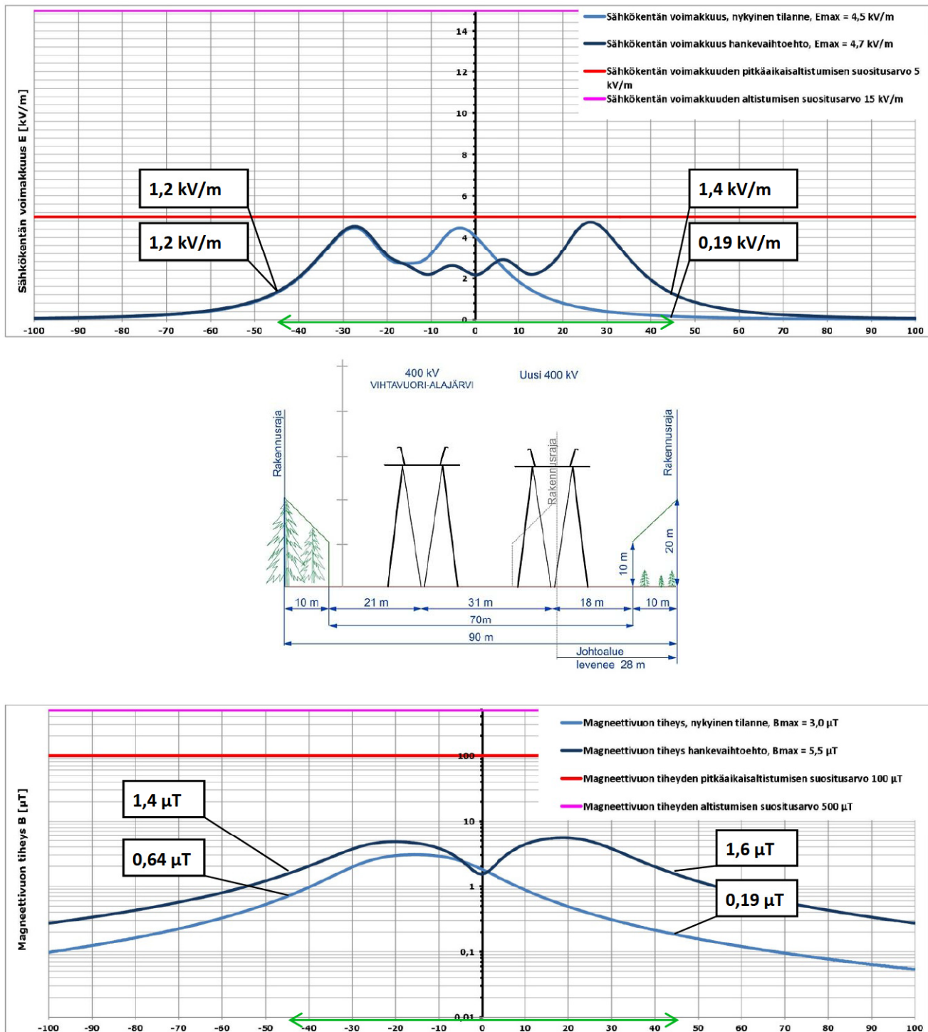
Kuva 157. Esimerkki sähkö- ja magneettikenttien voimakkuudesta ja ulottuvuudesta nykyisessä ja tulevassa tilanteessa poikkileikkauksessa 1B b-c (Pukinpohja – Puskianmäki). Vihreä nuoli havainnollistaa johtoalueen leveyttä.
