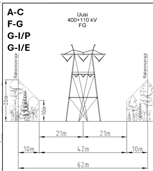
Kuva 4-5: Voimajohdon poikkileikkaukset reittisuudella Lahdenperä–Pysäysperä.
