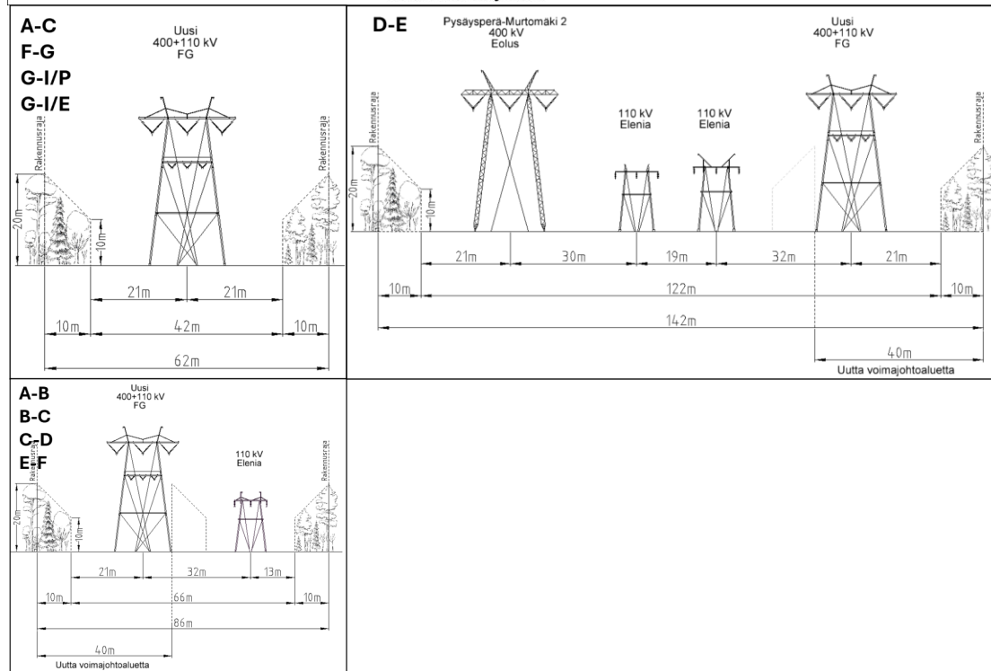
Kuva 4-4: Voimajohdon poikkileikkaukset reittiosuudella Kaakkuri–Lahdenperä.
