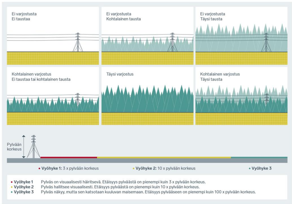
Kuva 5-20. Voimajohdon näkyvyyteen vaikuttavia tekijöitä (Maisema-arkkitehdit Byman ja Ruokonen Oy 2001).
