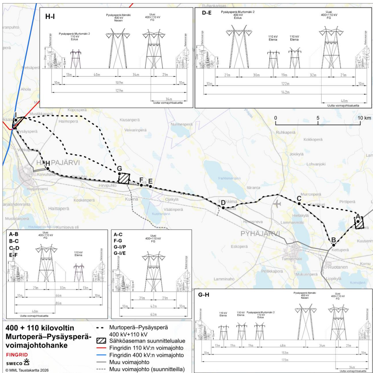
Kuva 4-2. Suunniteltujen voimajohtojen poikkileikkausvälit.
