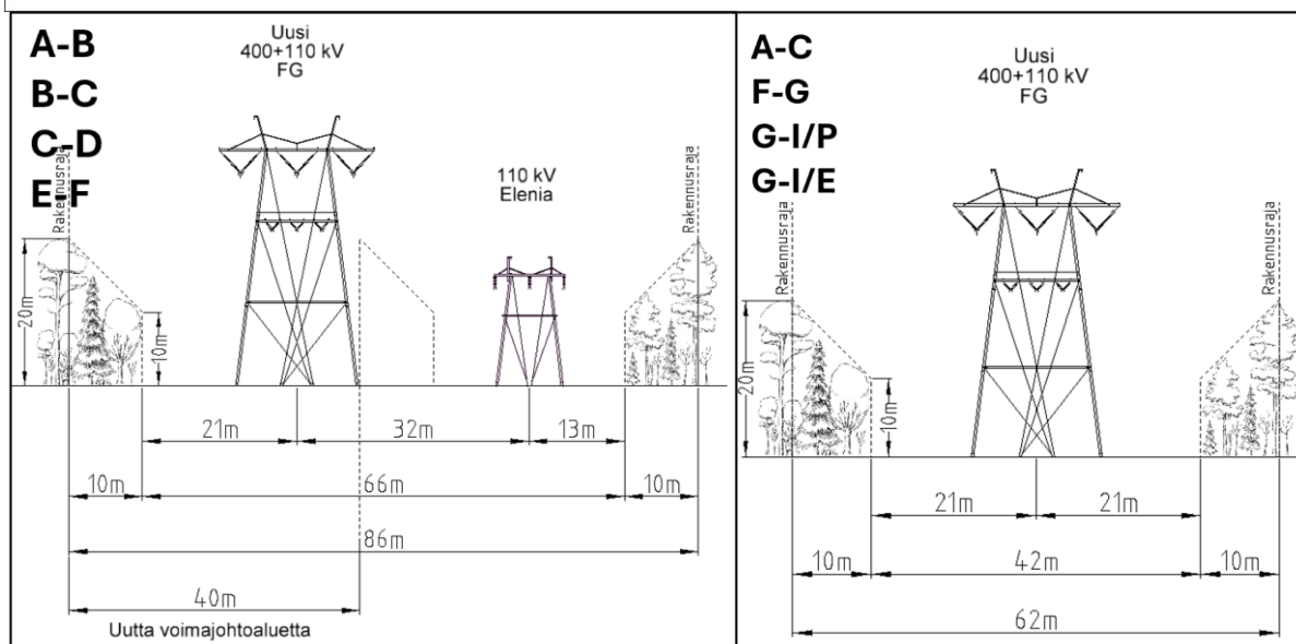
Kuva 4-3. Voimajohdon poikkileikkaukset reittisuudella Murtoperä–Kaakkuri.
