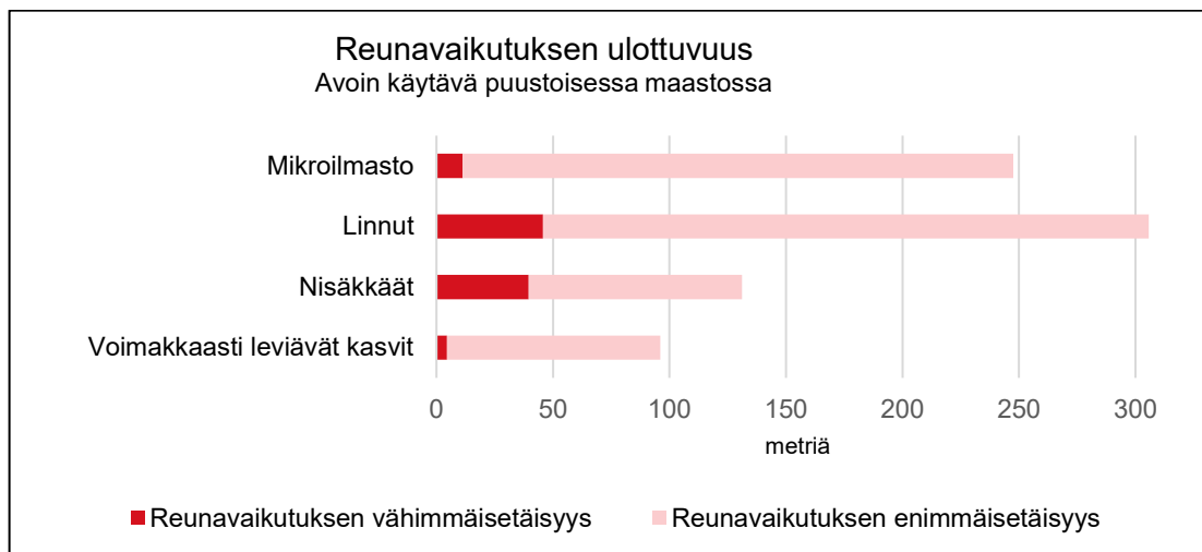
Kuva 5-26. Reunavaikutuksen todettuja ulottuvuuksia eri lajiryhmissä ja pienilmastossa puustoisessa maastossa (mukaillen Bentrup 2008).
