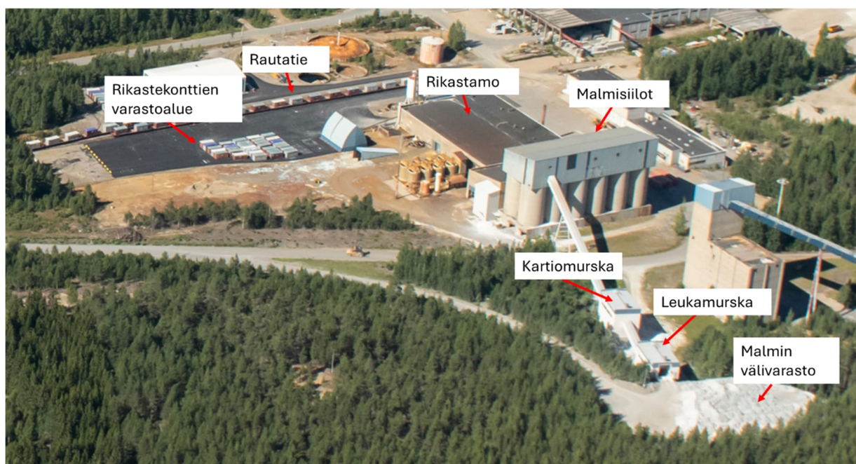
Kuva 3-3. Toimintojen sijoittuminen rikastamoalueelle.
