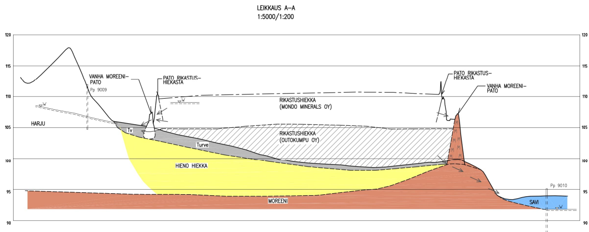
Kuva 6-14. Poikkileikkaus (ote) rikastushieka-altaan alueelta (Lassila ja Viitanen 2003).
