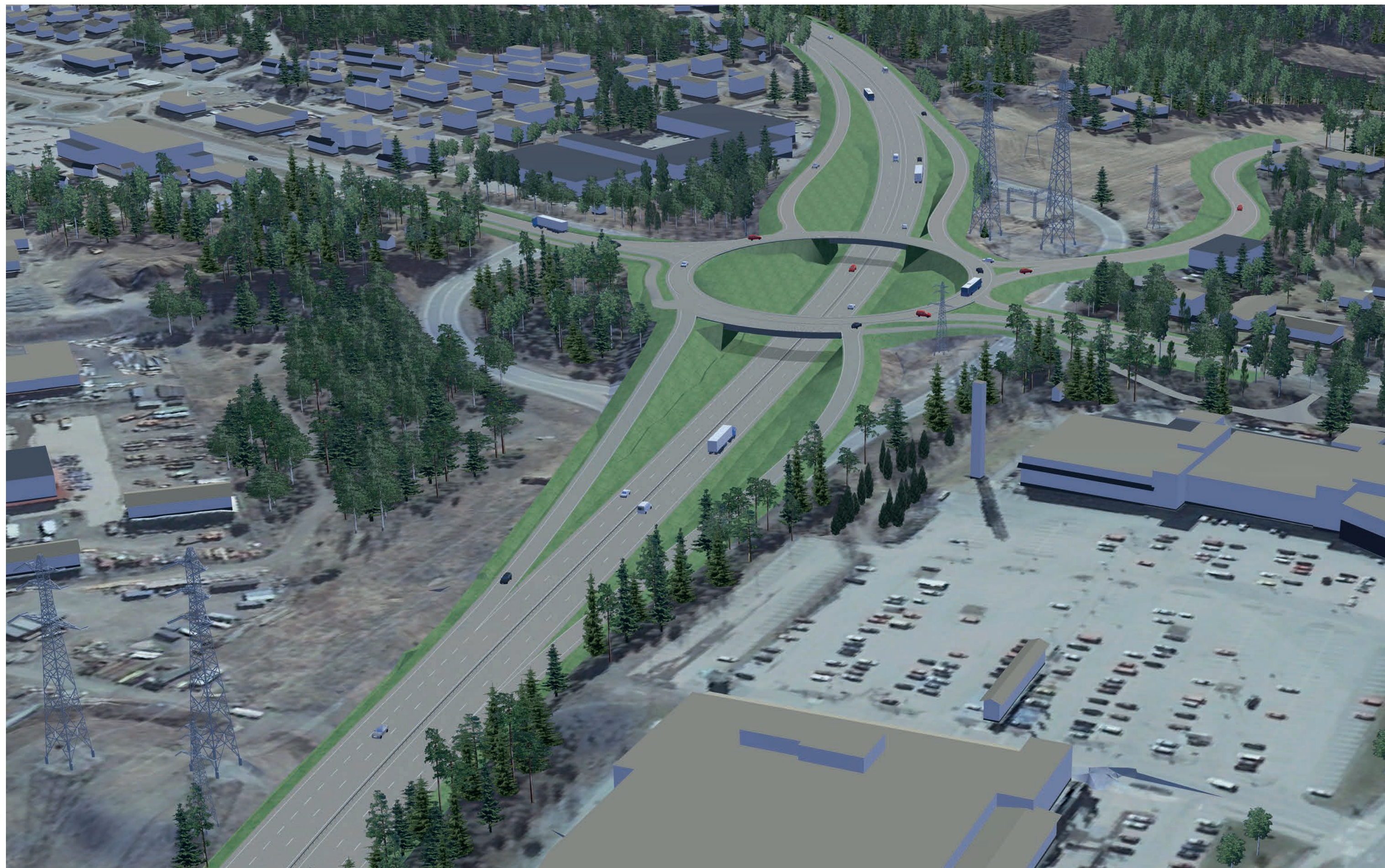
LENTOLAN ERITASOLIITTYMÄ E5 vaihtoehto 1
