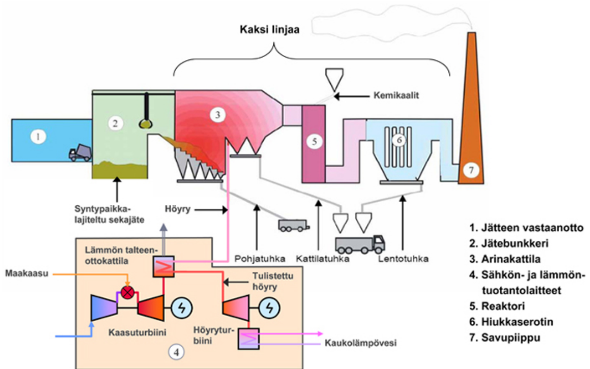
Kuva 3-2. Jätevoimalan toimintaperiaate.
