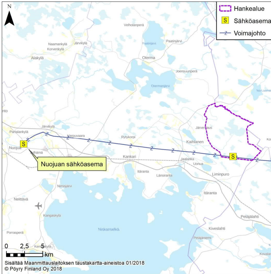
Kuva 5. Tuulipuiston sähkönsiirtoreitti.
