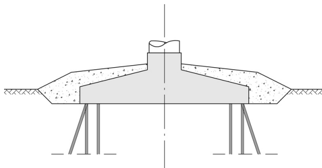
Kuva 4-6 Paaluperustus.
