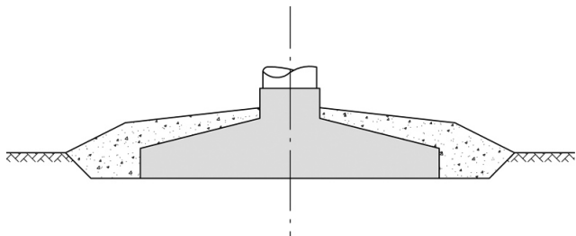
Kuva 4-4 Maavarainen teräsbetoniperustus.
