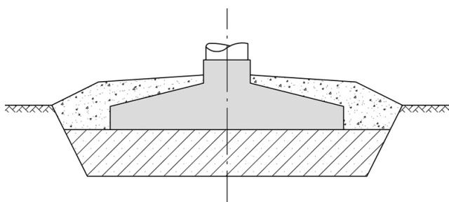
Kuva 4-5 Perustus massanvaihdolla.
