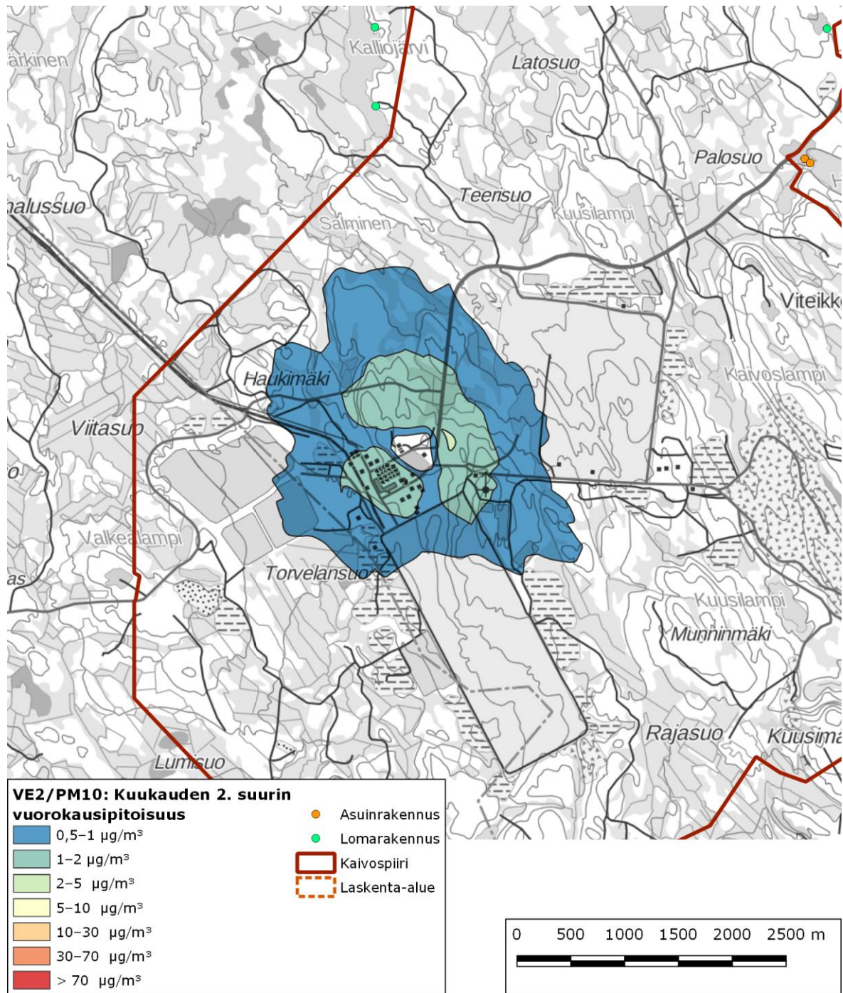
Kuva 8-11. Mallinnuksen mukaiset, PM 10 -vuorokausiohjearvoon (70 µg/m³) verrannolliset akkukemikaalitehtaan ja lämpölaitoksen päästöjen aiheuttamat pitoisuuslisät toteutusvaihtoehdossa VE2. Kaikki hiukaspäästö ei muodostu hengitettävistä hiukkasista, joten mallinnustulokset ovat esitettyjä arvoja pienemmät.
