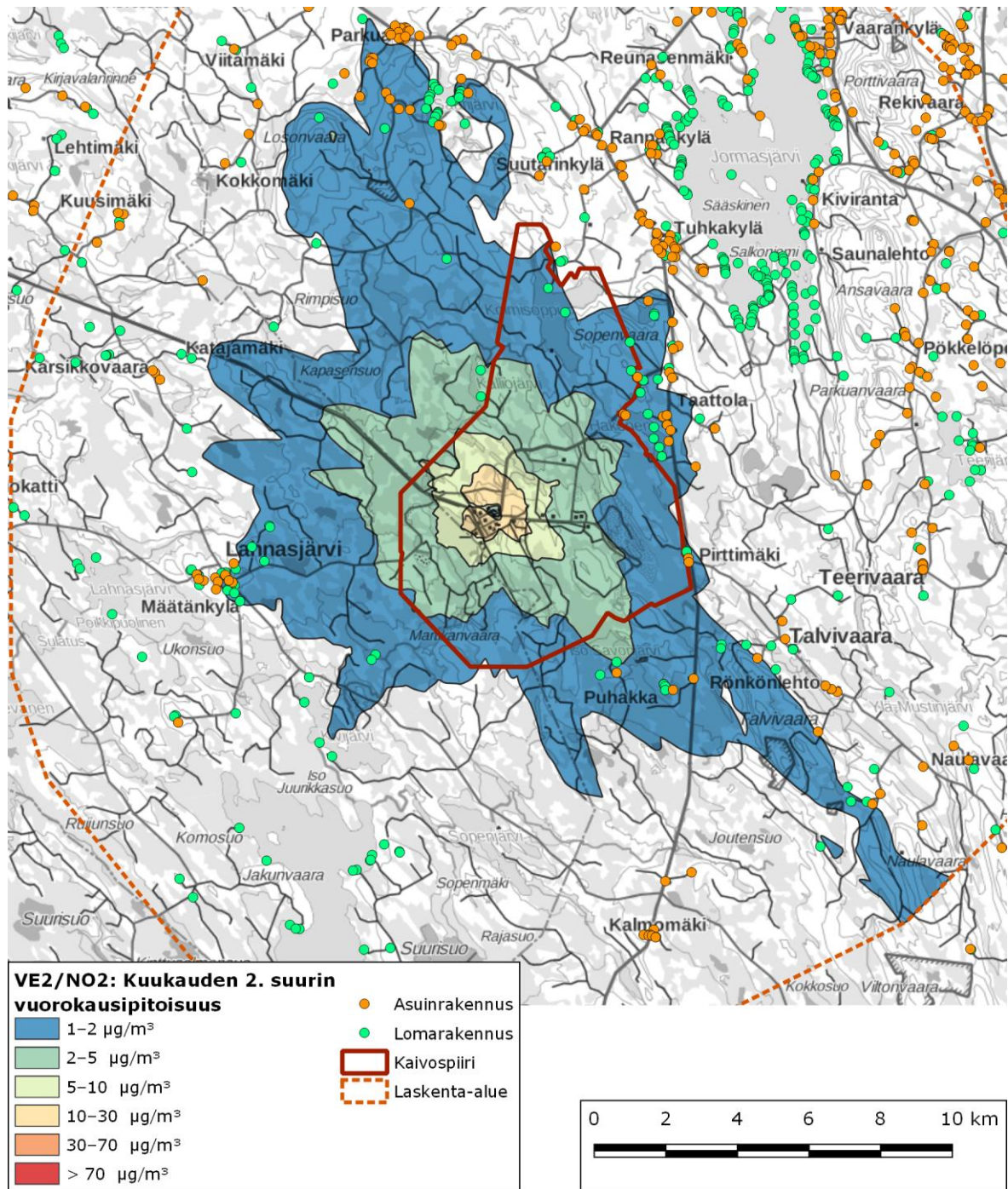
Kuva 8-8. Mallinnuksen mukaiset, vuorokausihaarvoon (70 µg/m 3 ) verrannolliset akkukemikaalitehtaan ja lämpölaitoksen päästöjen aiheuttamat NO 2 -pitoisuuslisät toteutusvaihtoehdossa VE2.
