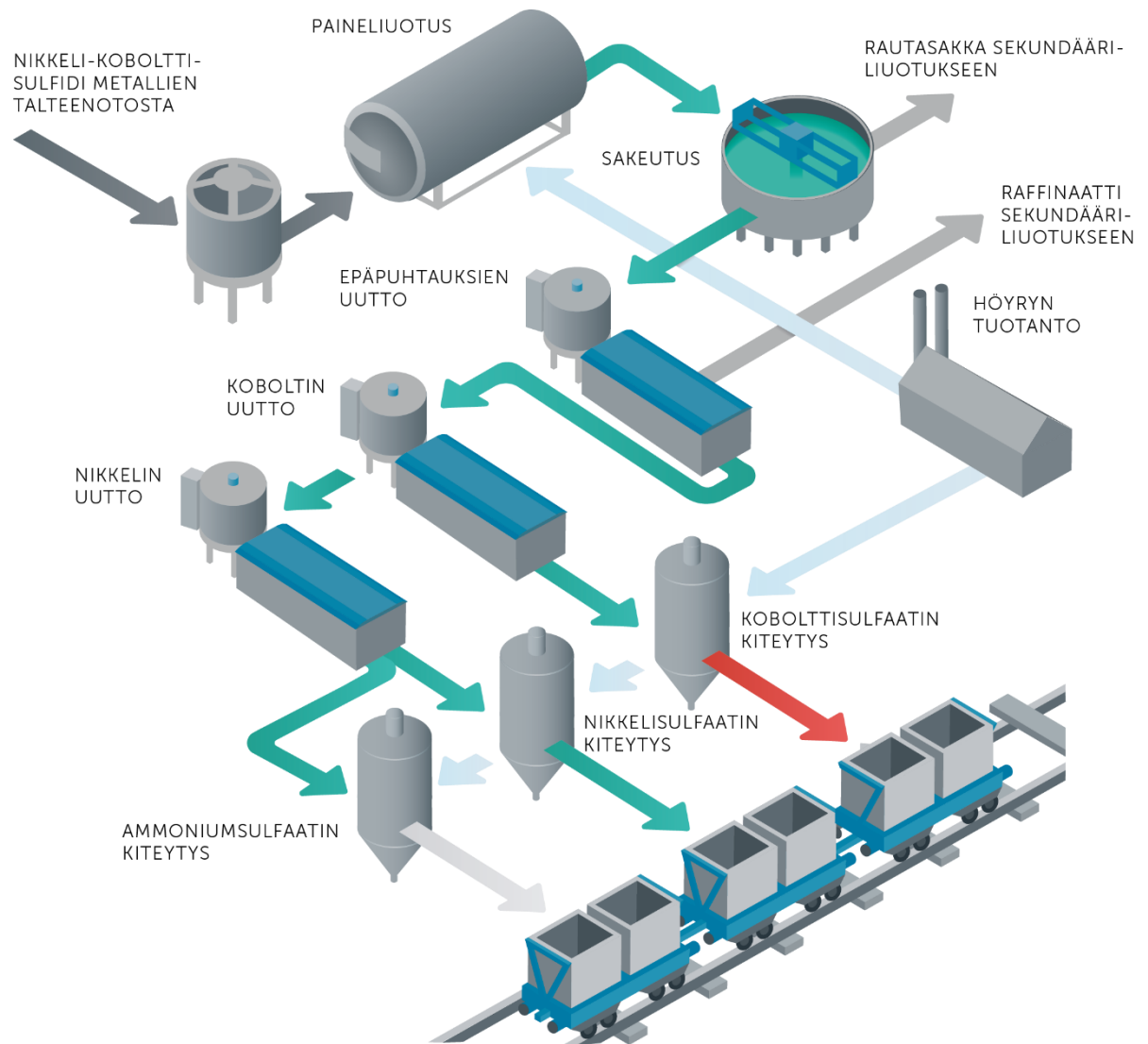
Kuva 3-6. Havainnekuva nikkeli- ja koboltisulfaattien tuotantoprosessista.
