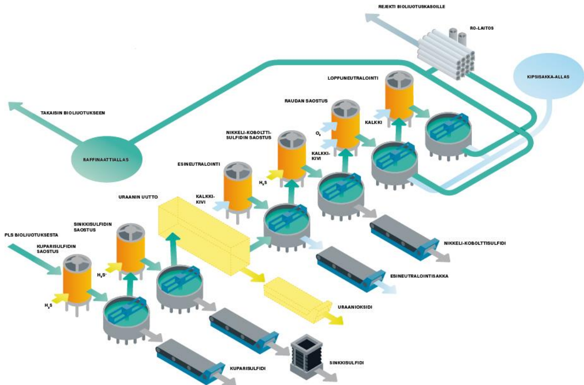
Kuva 3-3. Metallien talteenotto.
