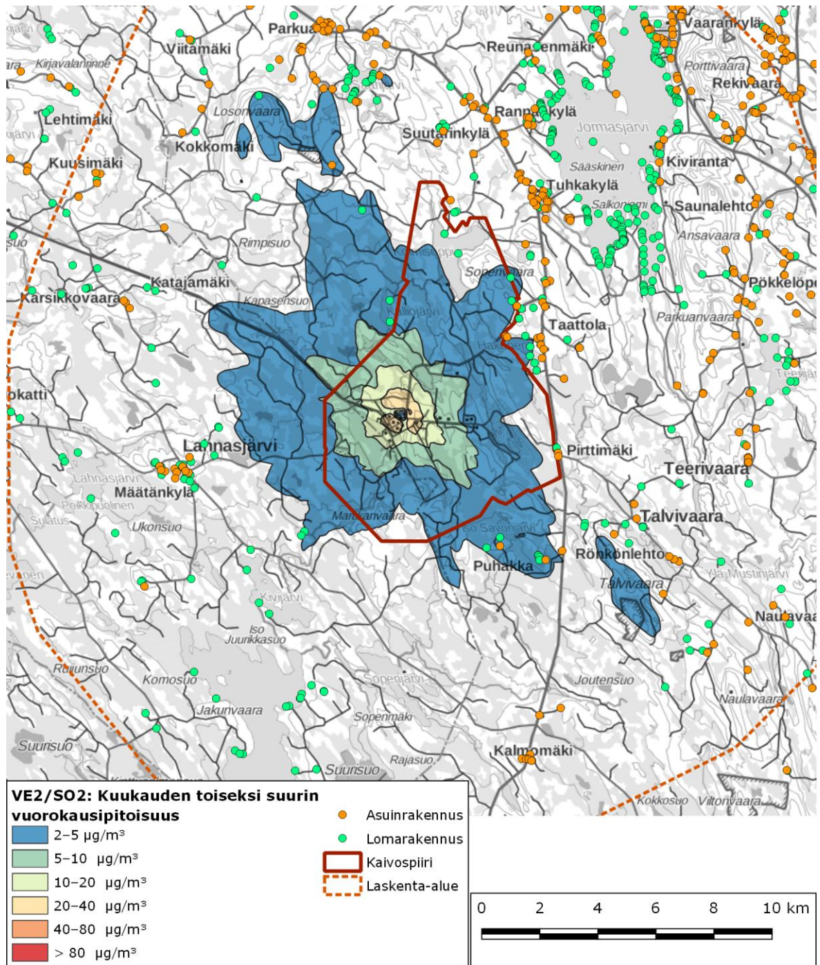
Kuva 8-10. Mallinnuksen mukaiset, vuorokausiohjearvoon ( 80 \mu\text{g}/\text{m}^3 ) verrannolliset akkukemikaalitehtaan ja lämpölaitoksen päästöjen aiheuttamat \text{SO}_2 -pitoisuuslisät toteutusvaihtoehdossa VE2.
