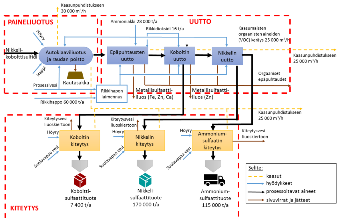
Kuva 3-7. Yksinkertaistettu prosessikaavio.
