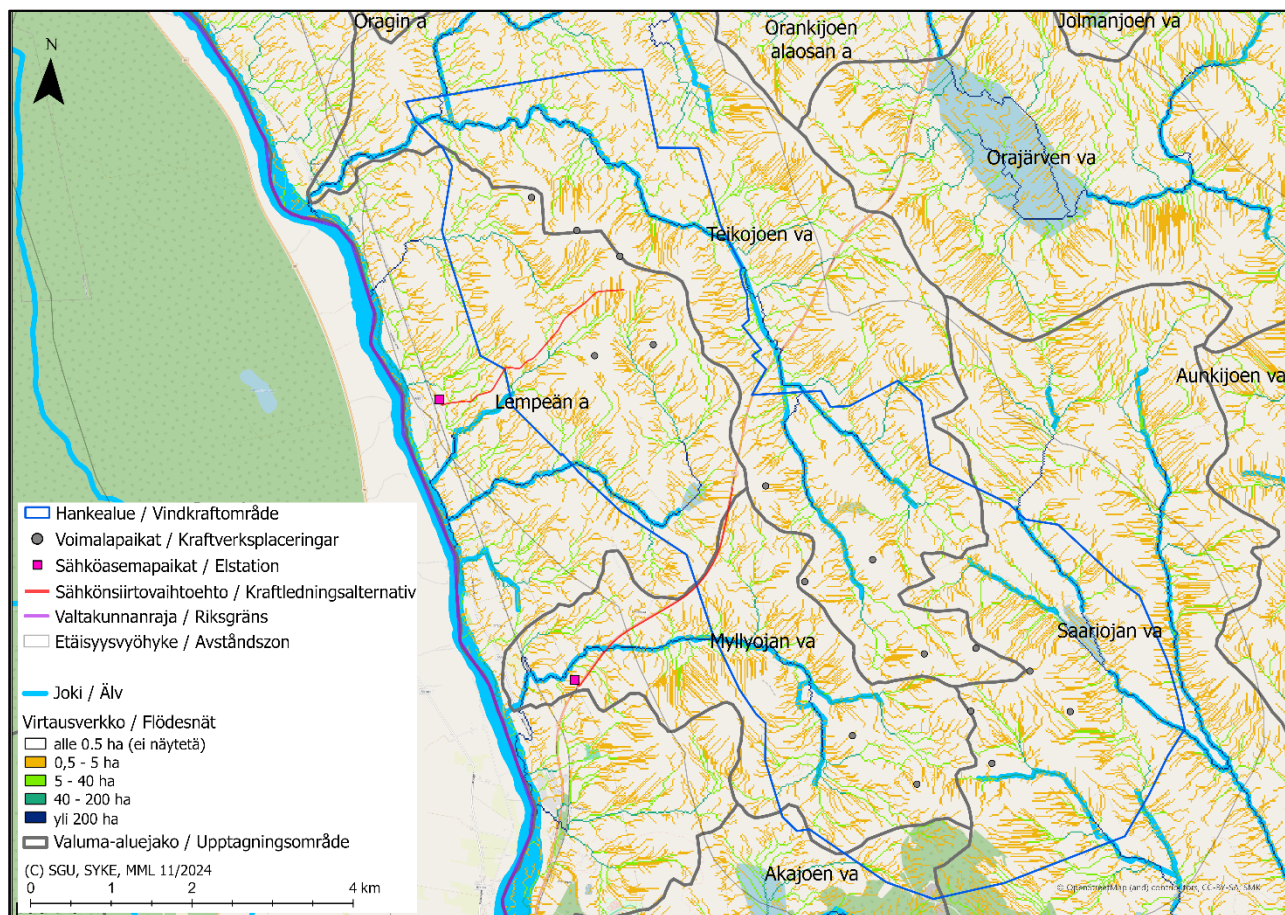
Bild 20. Projektområdets avrinningsområdesfördelning och ytvattens flödesnätverk.
