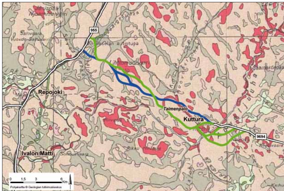
Govva 4.2. Plánenguovllu eanavuodđu. gártačilgehus: čuvgesruškes =morena, rukses=bákteeana, čuvgesrukses =juovva, juovva ja rášša, čuvgesruoná =čievra ja sáttu, čohkkesruoná =čorut, ránis=lavdnji. Gáldu Anára eanavuodđogárta 1:400 000, Geologian tutkimuskeskus, Espoo.
