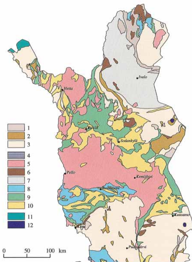
Govva 4-1 Yleistetty Pohjois-Suomen kallioperä (Johansson & Kujansuu 2005). Gártačilgehus: 1=gránihtalaš geađggit, 2=vulkanihtat ja daidda laktáseaddji sedimentageađggit, 3=gneissat, 4=sátto- ja ráktogeađgegeardi, 5=gránihtta, gránodiorihtat, tonalihtat, kvarcadiorihtat ja montsonihtat, 6=diorihtat, anortosihtat, gabroa ja peridotihtat, 7=Lappi gránulihttaavádaga gránáhtaigneissat ja diorihhtat, 8=kiilleráktu, gneissat ja migmatihtat, 9=vulkanhtat ja daidda laktáseaddji sedimentageađggit, 10=kvacihtta ja konglomeráhtat, 11=kaledonisialaš rávttut, gneissat ja intrusiivágeađggit, 12=álkálágeađggit ja kárbonáhta.
