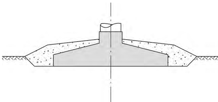
Kuva 3-8 Maavarainen teräsbetoniperustus.
