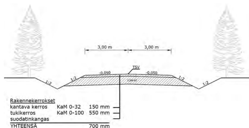
Kuva 3-12 Huoltotierakenteiden periaatepiirros.
