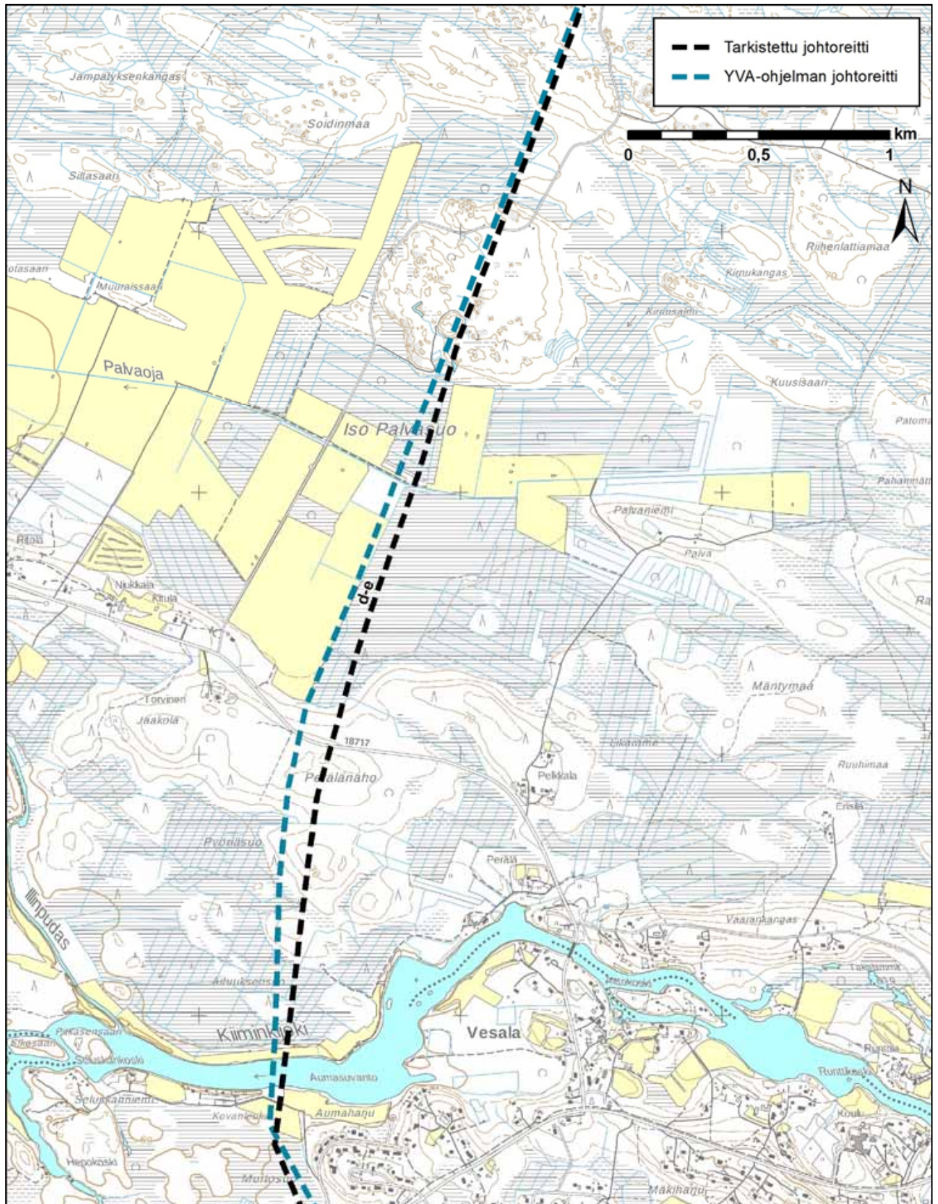
Kuva 17. Johtoreititarkistus Kiiminkijoen ja Iso Palvasuon välillä.
