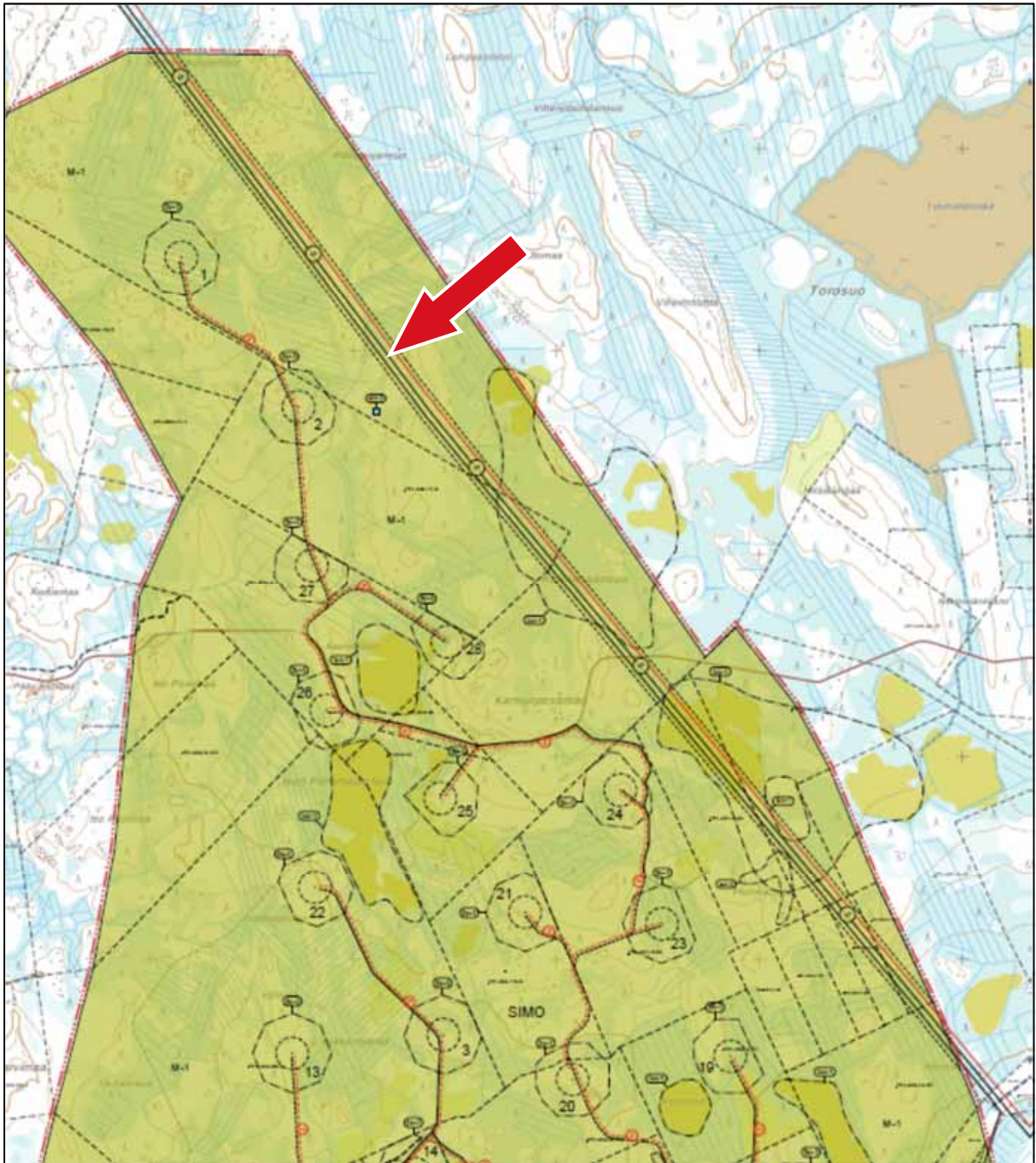
Kuva 51. Ote Leipiön tuulivoimapuiston laajennuksen yleiskaavasta. Tutkittava johtoreitti on osoitettu kaavassa varauksena. Punainen nuoli havainnollistaa tutkitavan voimajohtoreitin sijaintia.
