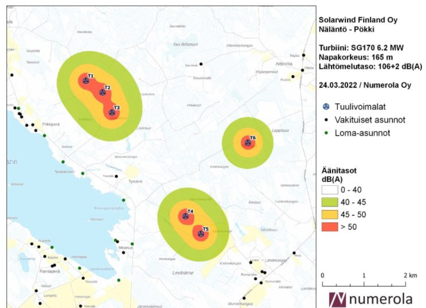
Kuva 4. Alustavan melumallinnuksen tulokset.
