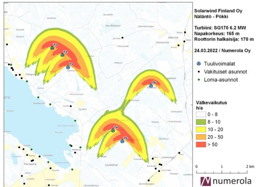
Kuva 5. Alustavan välkevarjostusmallinnuksen tulokset.
