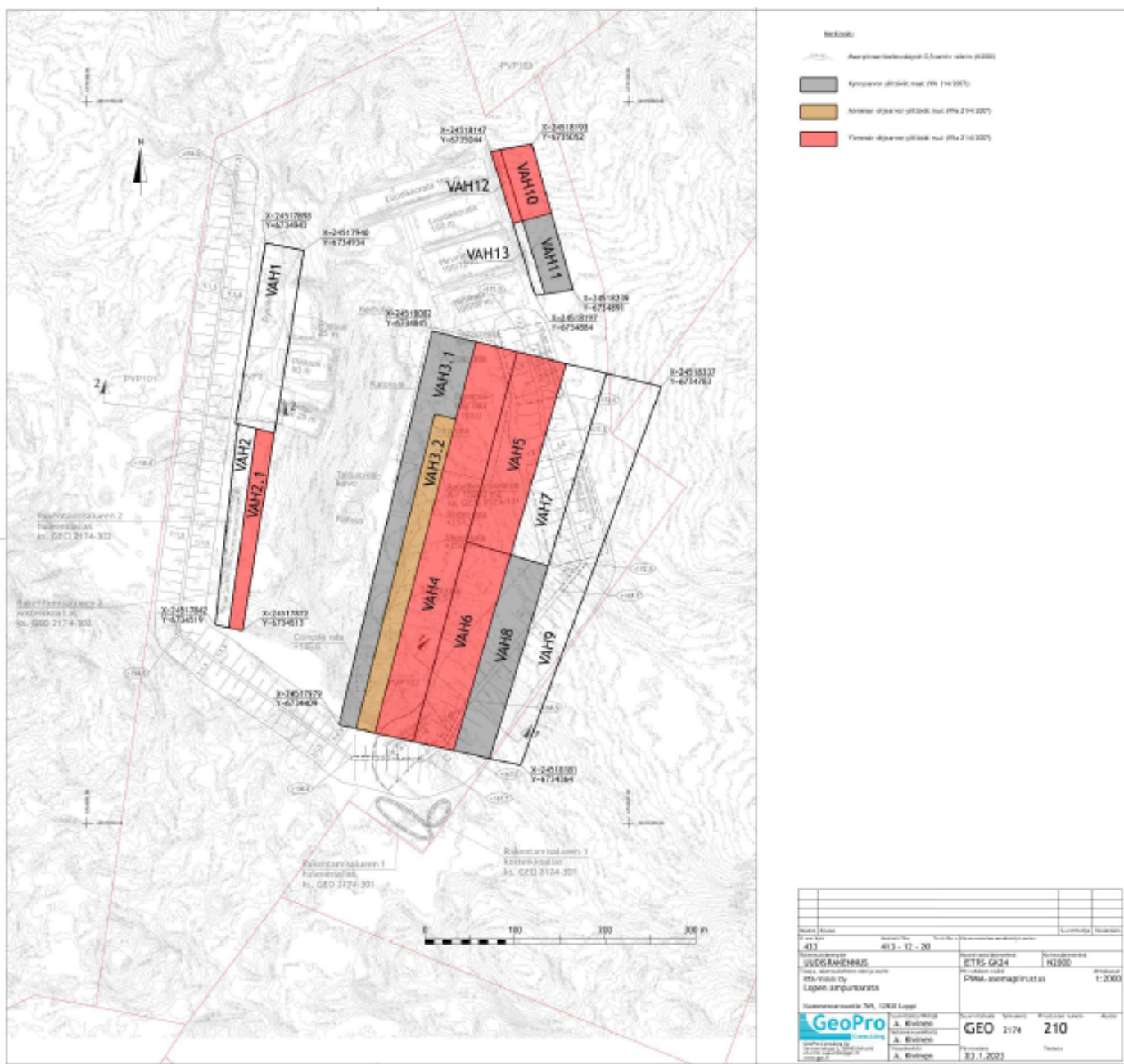
Kuva 3. PIMA-asemapiirustus. GeoPro Consulting Oy 23.1.2023.
