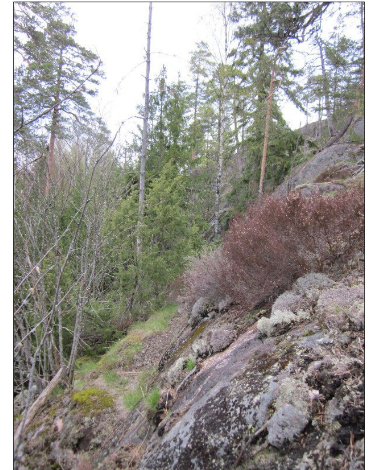
Kuva 7.16. Långkärrsbergetin länsireunassa on 200 metrin matkalla jyrkkä, 15–20 metriä korkea kallioseinä, jossa on sekä käveltäviä nousuja että pystysuoria seinämiä. Bild 7.16. I Långkärrsbergets västra utkant finns en 200 meter lång brant, 15–20 meter hög bergvägg, där finns både stigningar som man kan gå uppför och lodräta väggar.
