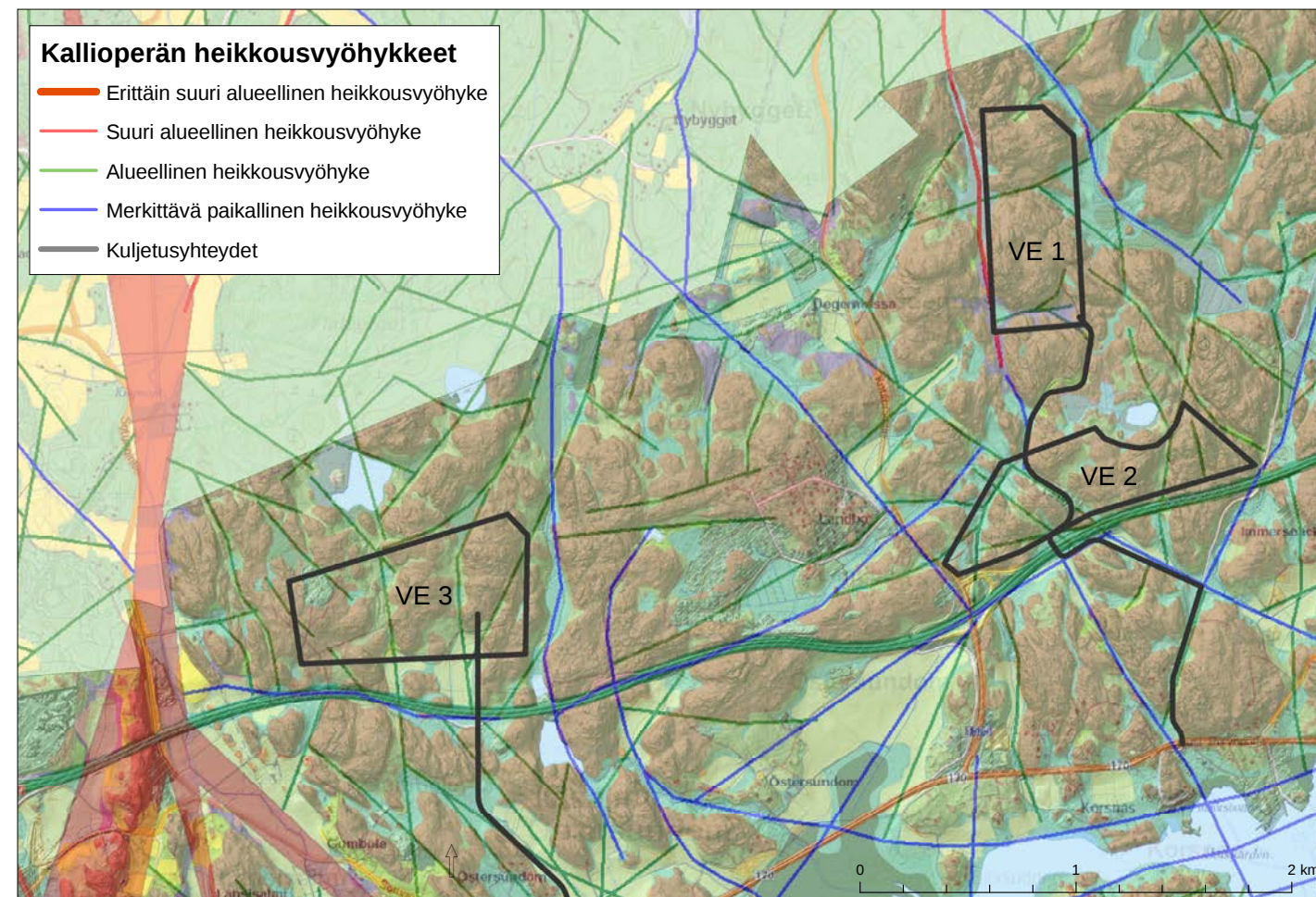
Kuva 7.20. Kallioperän heikkousvyöhykkeet ( http://geomaps2.gtk.fi/geotieto/ 12.5.2015) sekä maaperäkartta. Bild 7.20. Skölar i berggrunden. ( http://geomaps2.gtk.fi/geotieto/ 12.5.2015) samt jordmånskarta.
