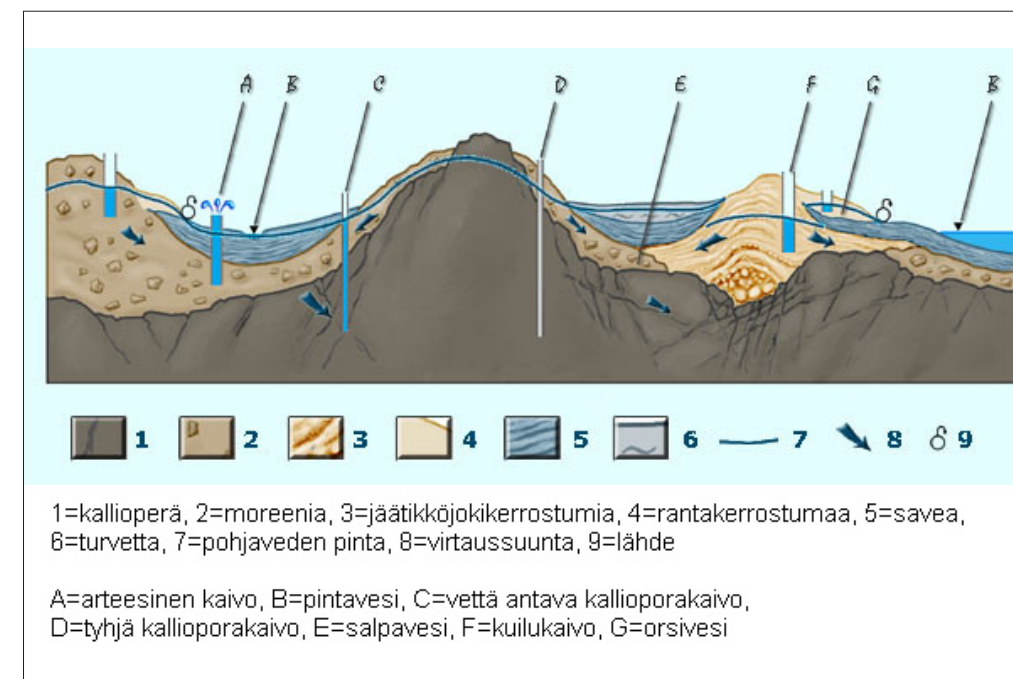
Pohjaveden esiintyminen. Piirros:Harri Kutvonen (lähde:GTK)
