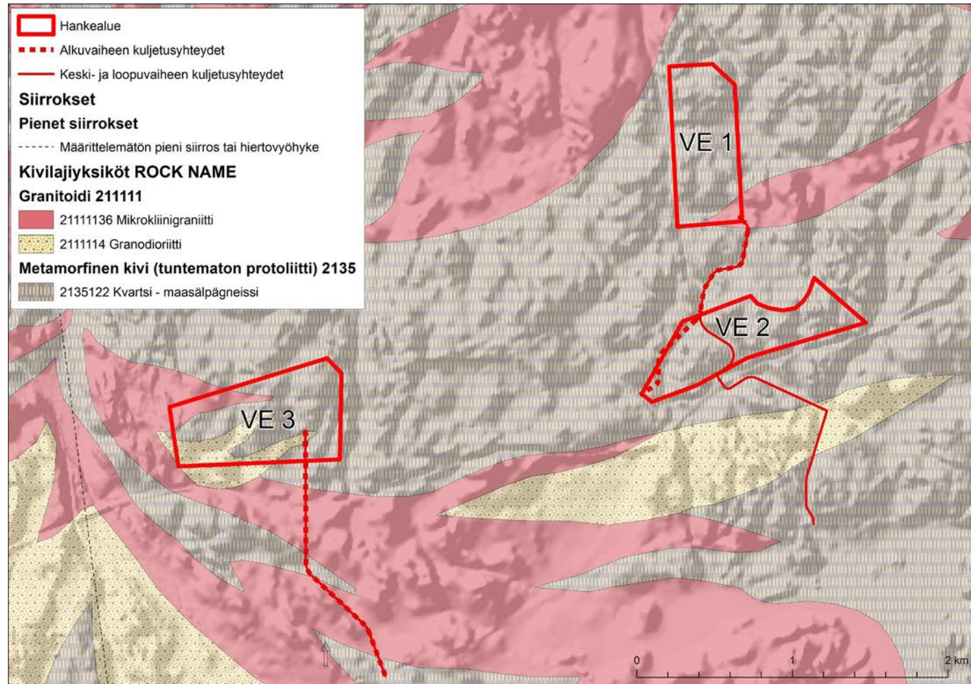
Kuva 7.15. Östersundomin kallioperäkartta. Gneissialueet ovat pääosin migmatiittisia eli seoksisia, joissa graniitit ja gneissit ovat limittäin (GTK).
