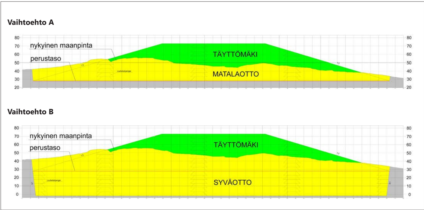
Kuva 4.2. Esimerkkipoikkileikkaukset matalan oton vaihtoehdoista A ja syväoton vaihtoehdoista B. Bild 4.2. Exempelgenomsärningsbilder av A-alternativen med grund täkt och B-alternativen med djup täkt.
