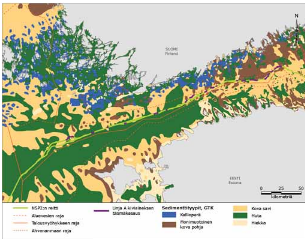
Kuva 4-3 Putkilinjojen käytön aikaisten liikkumisen vähentämisaikat ja sedimenttien luokittelu, GTK /4/. Osuuksilla, jonne kiviaineksen kasausta on suunniteltu, kiviainespenkereet rakennetaan 50 m välein.
