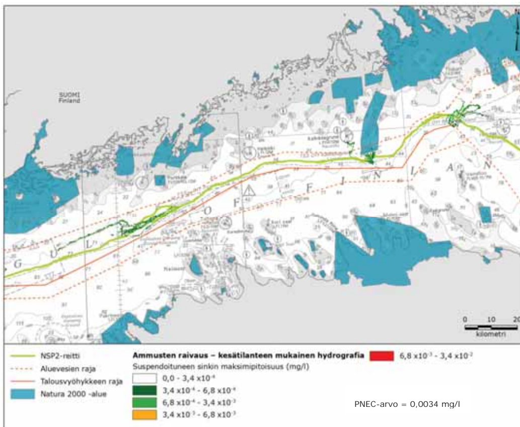
Kuva 6-43 Sinkin suurin pitoisuus ammusten raivaamisen aikana tyypillisissä kesäolosuhteissa. Suomenlahden itäosaa.
