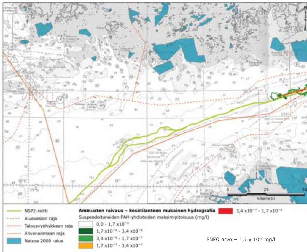
Kuva 6-28 Bentso(a)pyreenin (PAH) suurin pitoisuus ammusten raivaamisen aikana tyypillisissä kesäolosuhteissa. Suomenlahden länsiosaa.
