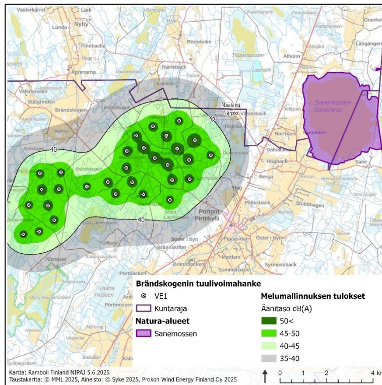
Kuva 5-1. Brändskogenin tuulivoimahankkeen aiheuttama toiminnan aikainen melu vaihtoehdossa VE1 Ramboll 2025d mukaisesti.
