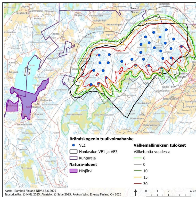
Kuva 5-4. Brändskogenin tuulivoimahankkeen aiheuttama toiminnan aikainen välke vaihtoehdossa VE1 välkemallinnuksen mukaisesti.
