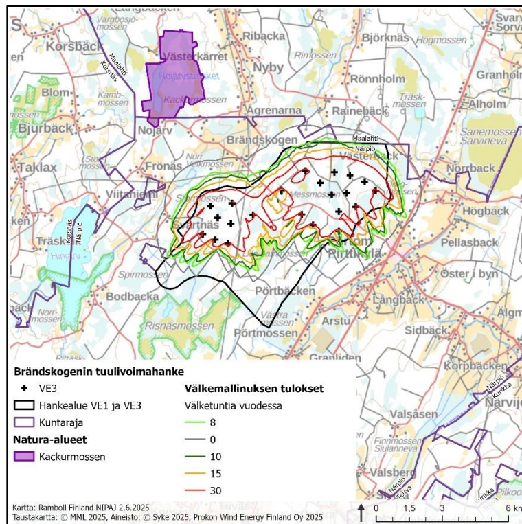
Kuva 5-6. Brändskogenin tuulivoimahankkeen aiheuttama toiminnan aikainen välke vaihtoehdossa VE3 Ramboll 2025g mukaisesti.
