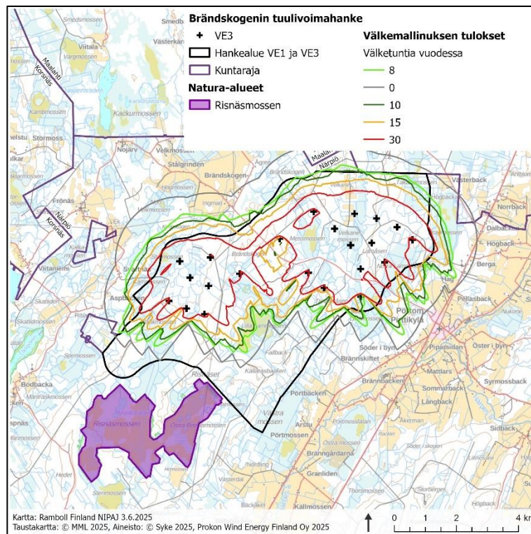
Kuva 5-6. Brändskogenin tuulivoimahankkeen aiheuttama toiminnan aikainen välke vaihtoehdossa VE3 välkemaalinnuksen mukaisesti.
