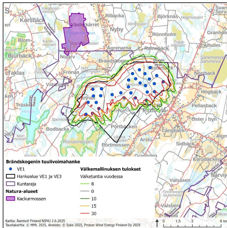
Kuva 5-4. Brändskogenin tuulivoimahankkeen aiheuttama toiminnan aikainen välike vaihtoehdossa VE1 Ramboll 2025g mukaisesti.
