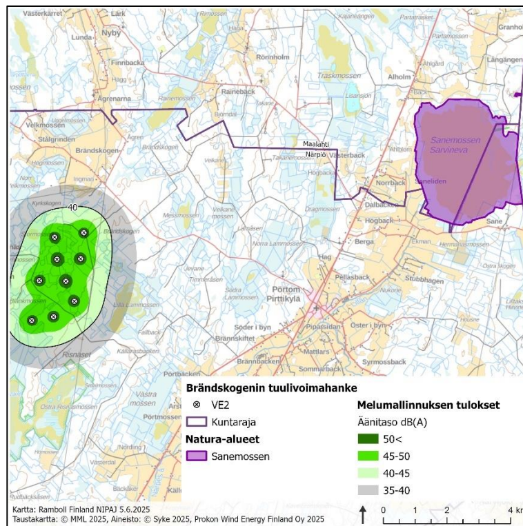
Kuva 5-2. Brändskogenin tuulivoimahankkeen aiheuttama toiminnan aikainen melu vaihtoehdossa VE2 Ramboll 2025d mukaisesti.
