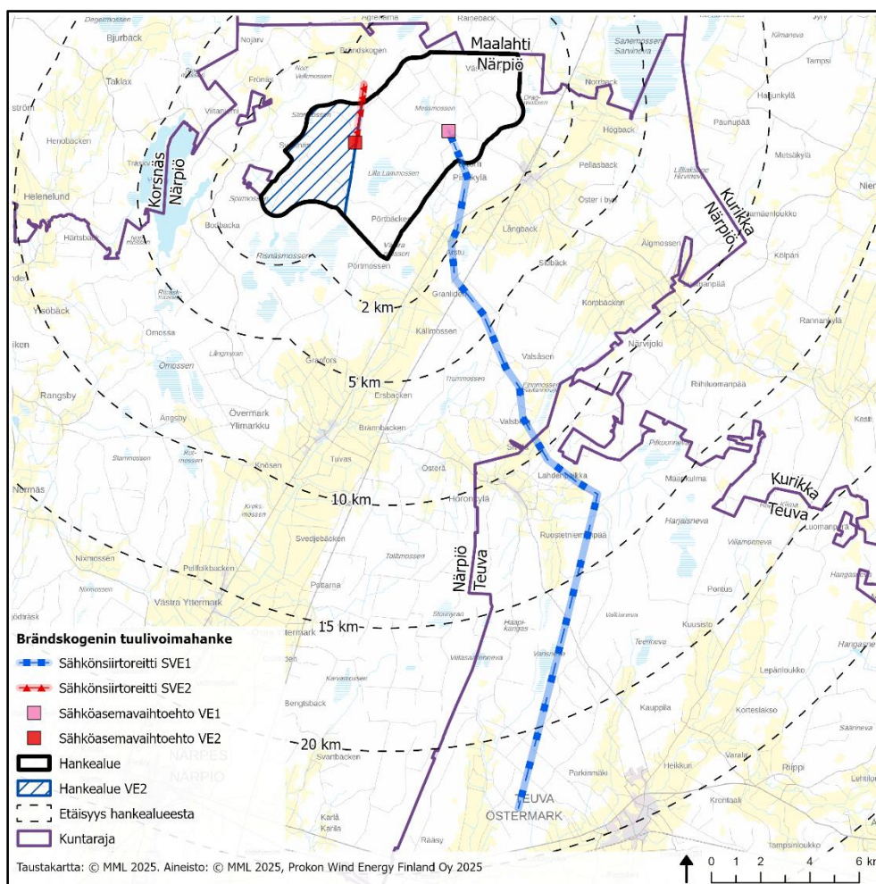
Kuva 4-3. Sähkönsiirtoreitin vaihtoehdot.
