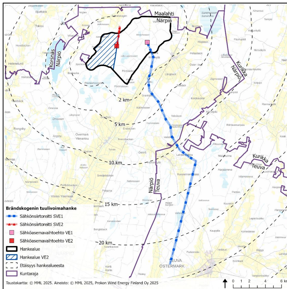
Kuva 4-3. Sähkösiirtoreitin vaihtoehdot.
