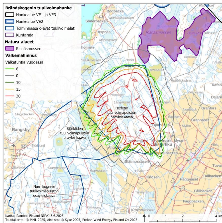
Kuva 6-10. Hedetin toiminnassa olevan tuulivoimahankkeen aiheuttama välkevaikutus Risnäs mossenin Natura-alueelle Ramboll 2025f mukaisesti.
