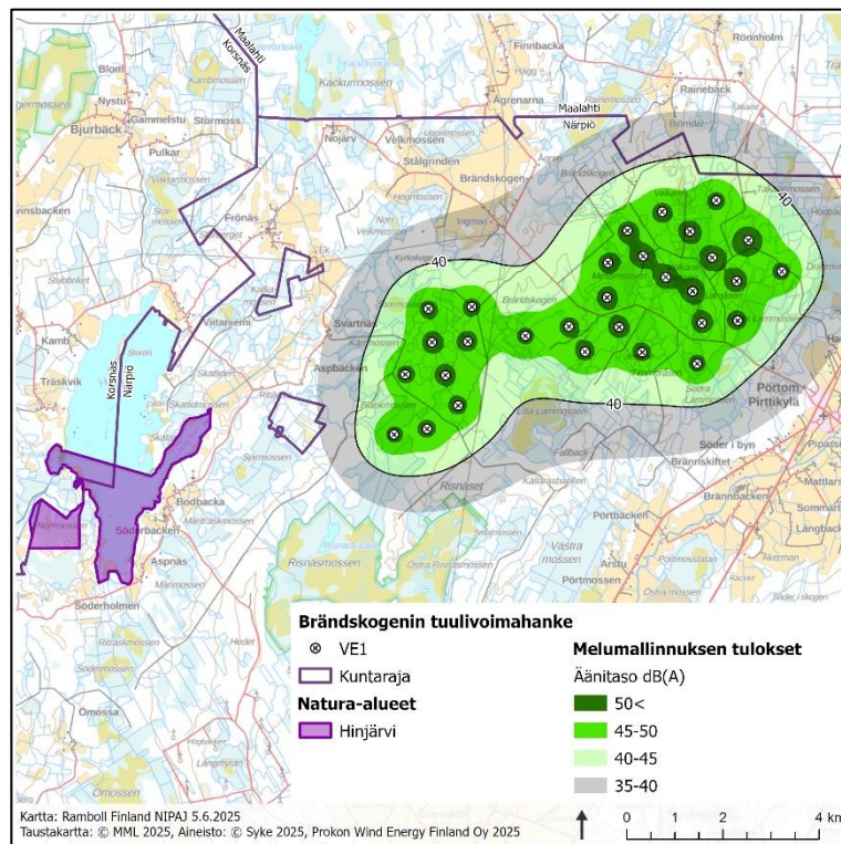
Kuva 5-1. Brändskogenin tuulivoimahankkeen aiheuttama toiminnan aikainen melu vaihtoehdossa VE1 mallinnuksen mukaisesti.
