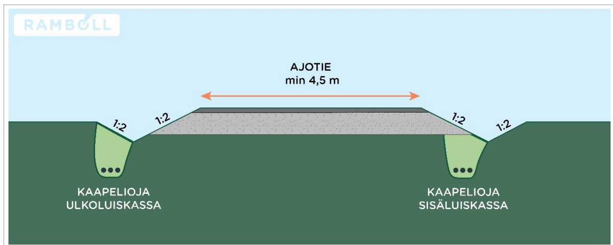
Kuva 4-7. Periaatekuva huoltotien rakenteesta.
