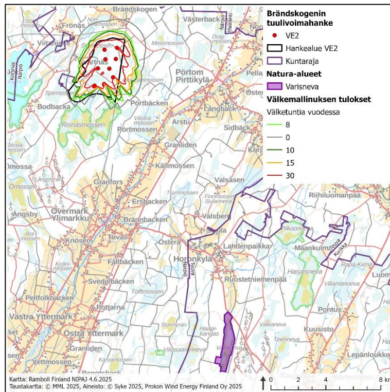
Kuva 5-5. Brändskogenin tuulivoimahankkeen aiheuttama toiminnan aikainen välke vaihtoehdossa VE2 Ramboll 2025d mukaisesti.
