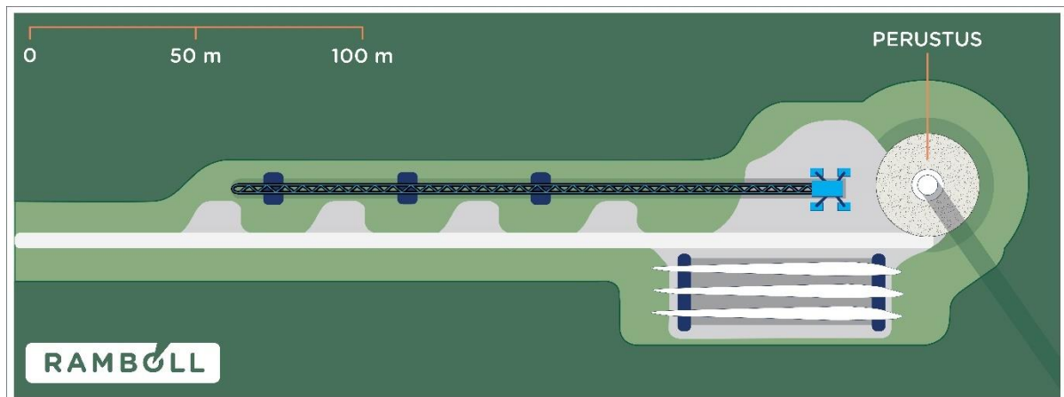
Kuva 4-6. Periaatekuva tuulivoimalan kenttä- ja nostoalueesta.
