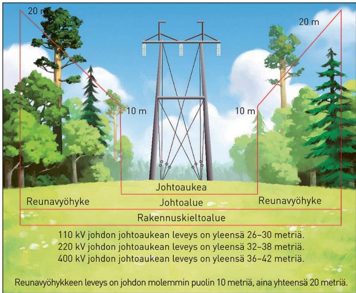
Kuva 4-8. Voimajohtoalueen poikkileikkaus sekä eri voimajohtojen johtoaukean leveydet (Ramboll 2025g).
