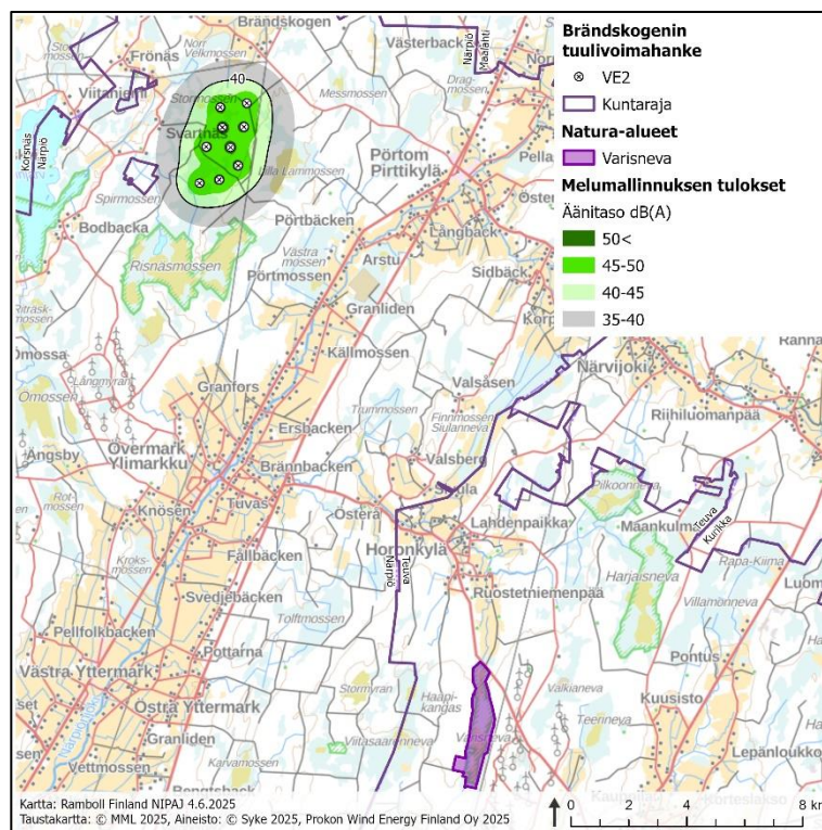
Kuva 5-2. Brändskogenin tuulivoimahankkeen aiheuttama toiminnan aikainen melu vaihtoehdossa VE2 Ramboll 2025c mukaisesti.
