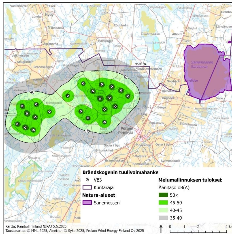
Kuva 5-3. Brändskogenin tuulivoimahankkeen aiheuttama toiminnan aikainen melu vaihtoehdossa VE2 Ramboll 2025d mukaisesti.
