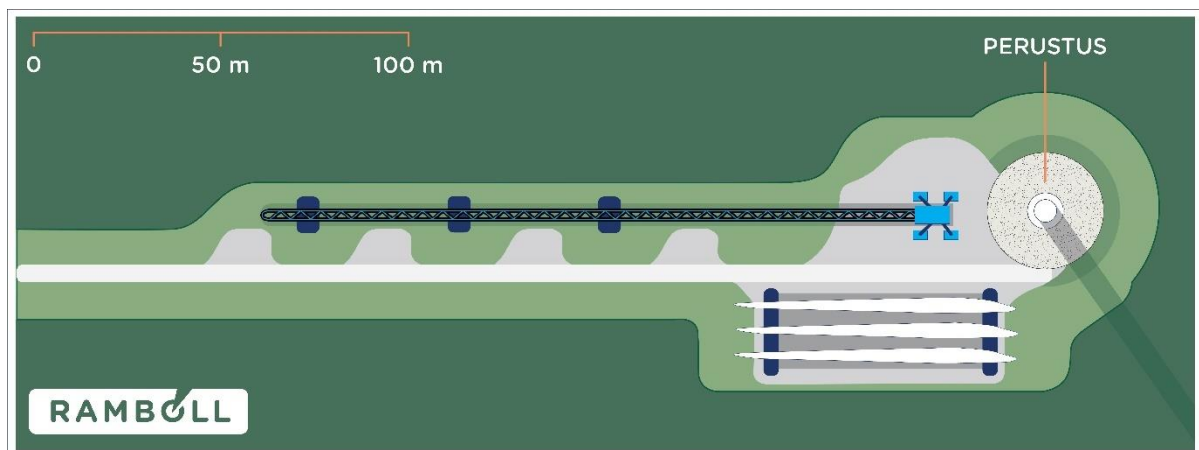
Kuva 4-6. Periaatekuva tuulivoimalan kenttä- ja nostoalueesta.
