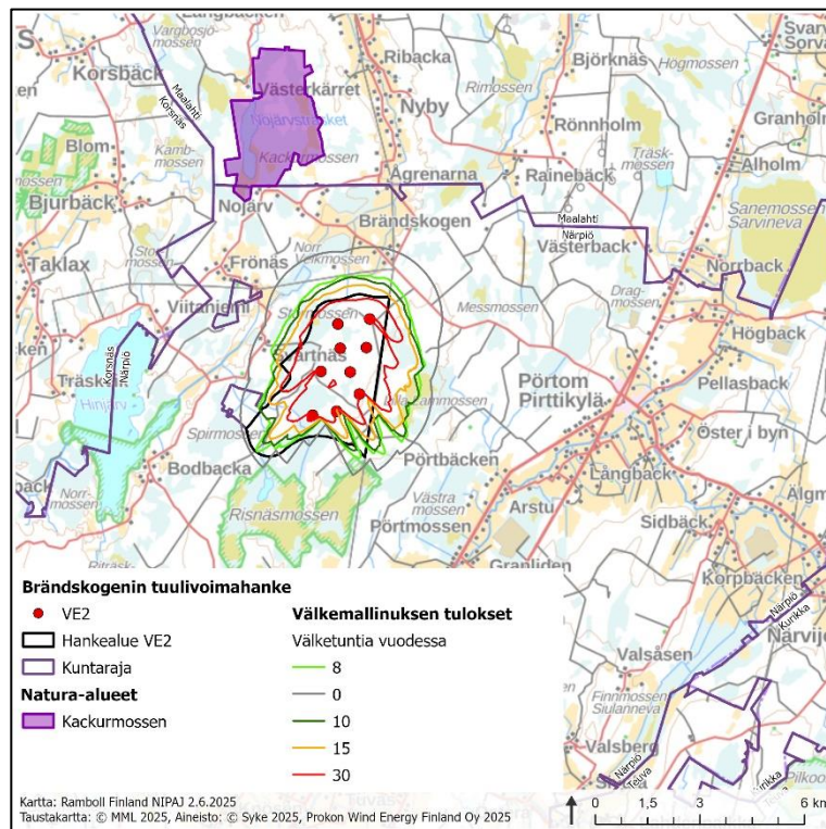
Kuva 5-5. Brändskogenin tuulivoimahankkeen aiheuttama toiminnan aikainen välke vaihtoehdossa VE2 Ramboll 2025g mukaisesti.
