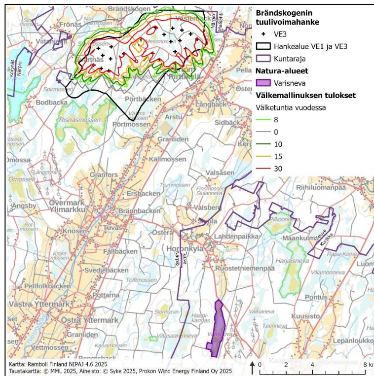
Kuva 5-6. Brändskogenin tuulivoimahankkeen aiheuttama toiminnan aikainen välke vaihtoehdossa VE3 Ramboll 2025d mukaisesti.
