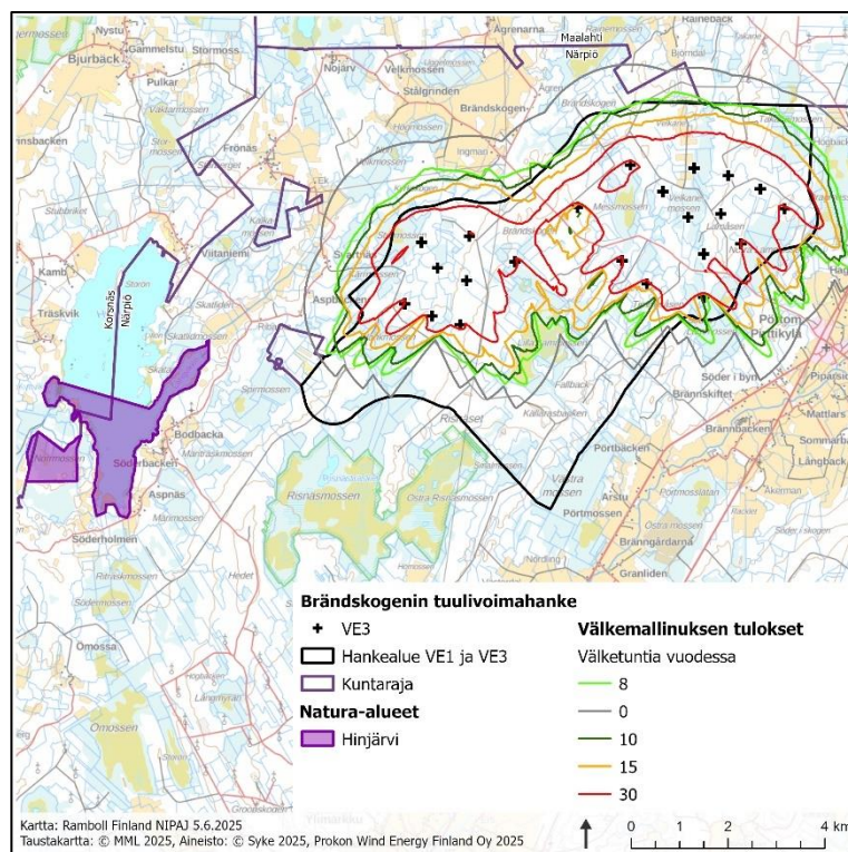
Kuva 5-6. Brändskogenin tuulivoimahankkeen aiheuttama toiminnan aikainen välke vaihtoehdossa VE3 välkemallituksen mukaisesti.
