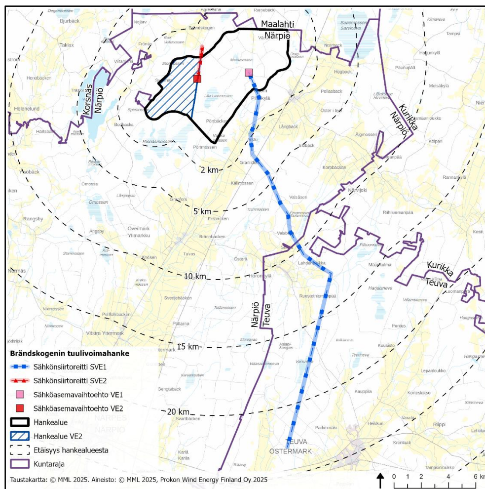
Kuva 4-3. Sähkönsiirtoreitin vaihtoehdot.
