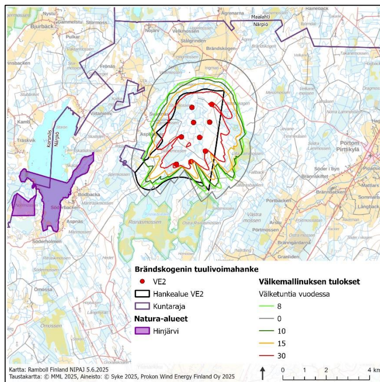
Kuva 5-5. Brändskogenin tuulivoimahankkeen aiheuttama toiminnan aikainen välke vaihtoehdossa VE2 välkemallituksen mukaisesti.
