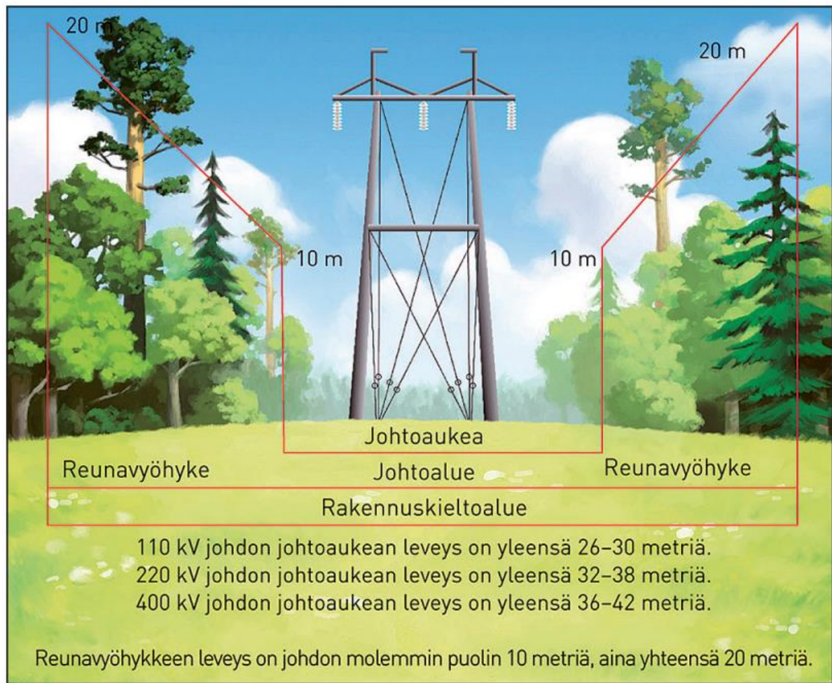
Kuva 4-8. Voimajohtoalueen poikkileikkaus sekä eri voimajohtojen johtoauekan leveydet (Ramboll 2025g).
