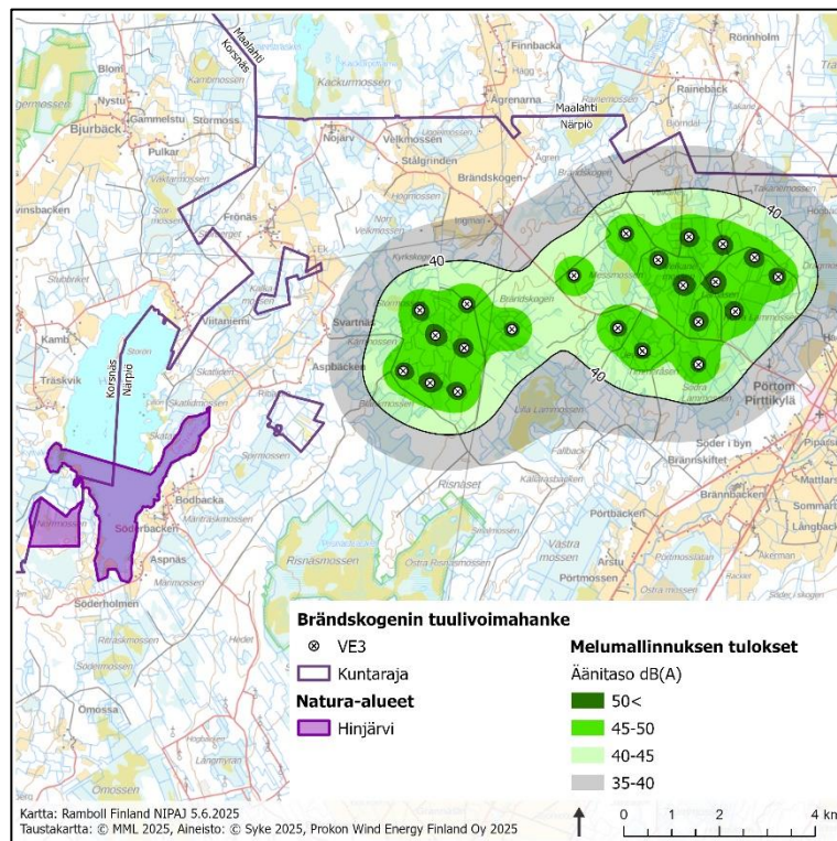
Kuva 5-3. Brändskogenin tuulivoimahankkeen aiheuttama toiminnan aikainen melu vaihtoehdossa VE3 mallinnuksen mukaisesti.
