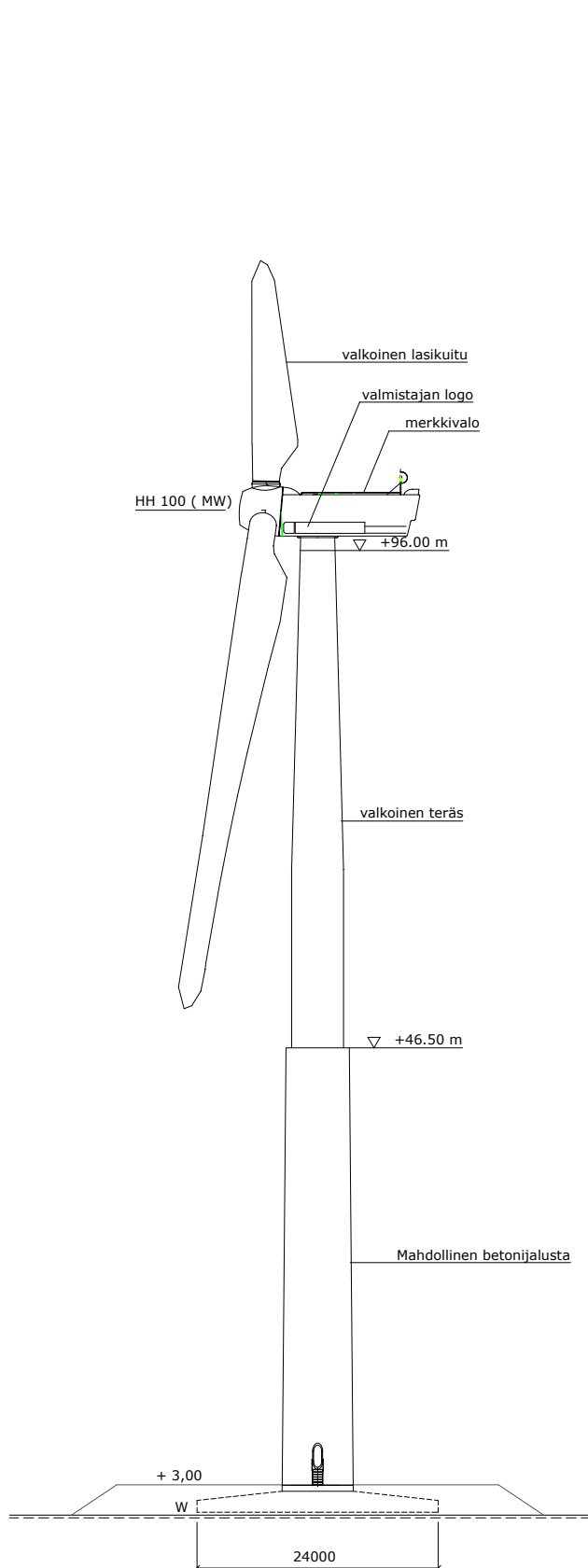
■ Kuva 4-5. 3 MW ja 5MW tuulivoimalaitosten periaatepiirros.
