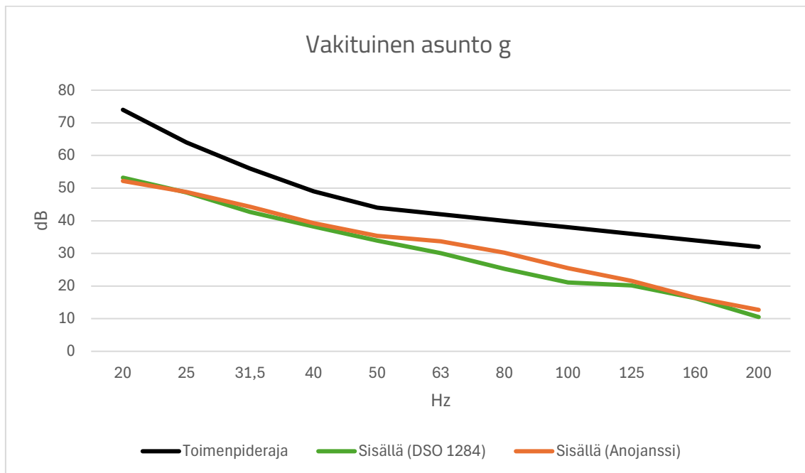
Kuva 8. Ympäristöministeriön ohjeistuksen mukainen pienitaajuisen melun laskenta sekä sosiaali- ja terveysministeriön toimenpiderajat vakituksessa asunnossa g.
