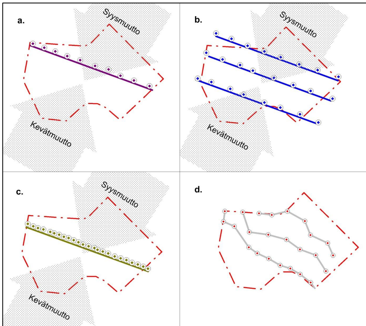
Kuva 15-10. Törmäysarviointien teoreettiset vaihtoehdot (VE 1:n mukaisesti): a. voimaloita 1. rivissä 10 (muiden voimaloiden osalta väistö), b. voimalat 3 rivissä ja jokaisen rivin osalta läpilento, c. voimalat tiivistetty yhteen riviin sekä d. VE1 mukaiset voimaloiden sijoituspaikat. Punaisella esitetty Mastokankaan hankealueen raja ja harmailla nuolilla pääasialliset muuttosuunnat.
