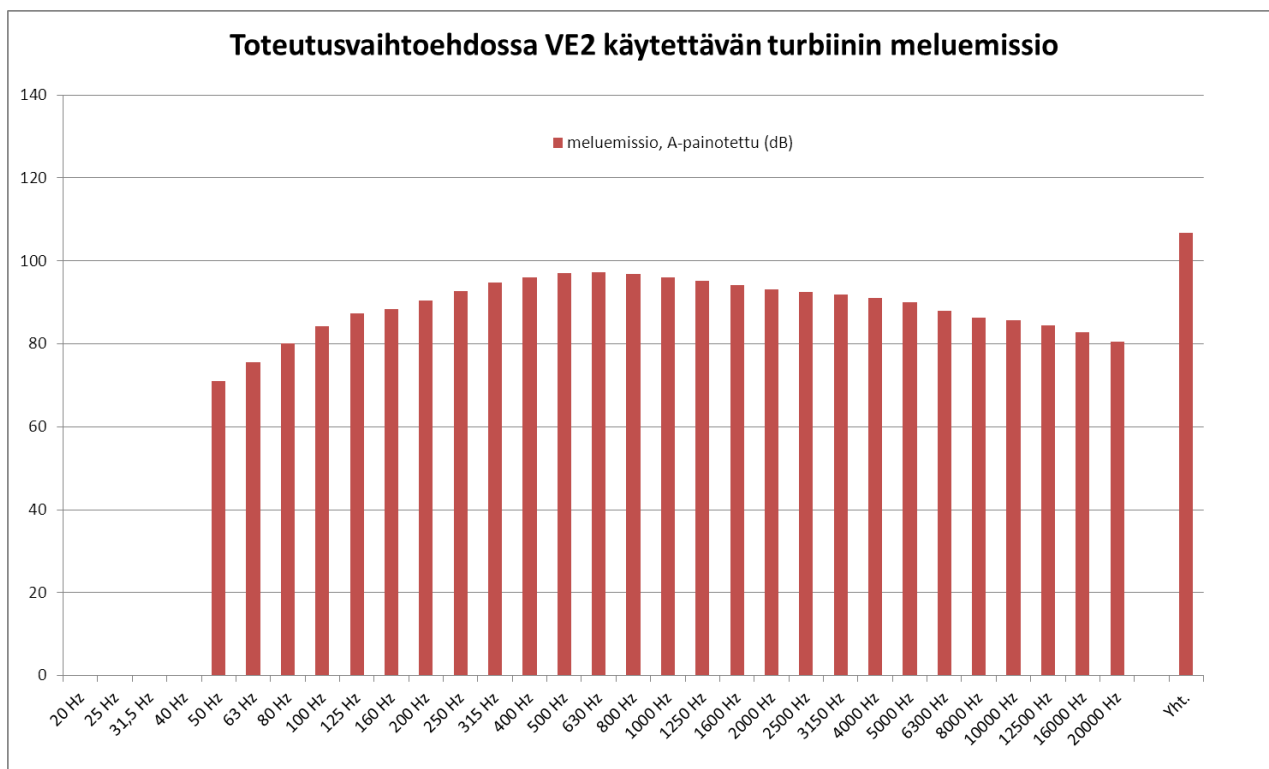
Kuva 7-2. Toteutusvaihtoehdossa VE2 käytettävän 4,5 MW tuulivoimalan A-painotettu meluemissio LW,A) terssikaistoittain tuulen nopeudella 8 m/s.
