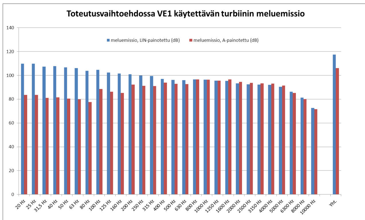
Kuva 7-1. Toteutusvaihtoehdossa VE1 käytettävän 3,0 MW tuulivoimalan A-painotettu meluemissio LW,A) ja painottamaton meluemissio (LW,LIN) terssikaistoittain tuulen nopeudella 8 m/s.
