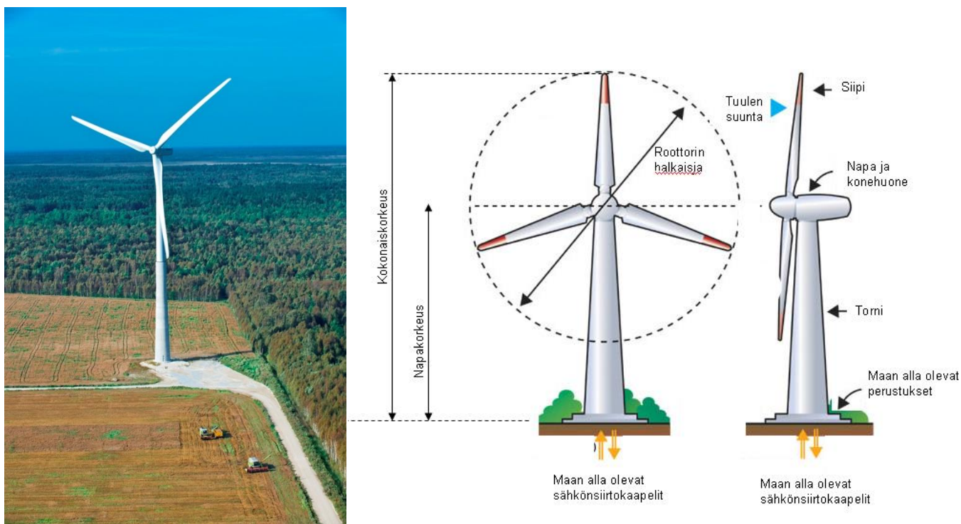
Kuva 4-3. Vasemmalla 3 MW:n tuulivoimalaitos, jonka tornin alaosa on betonia ja yläosa terästä, napakorkeus ja roottori ovat 100 m (kuva: WinWinD). Oikealla on periaatekuva tuulivoimalasta (kuva: planete-energies.com).
