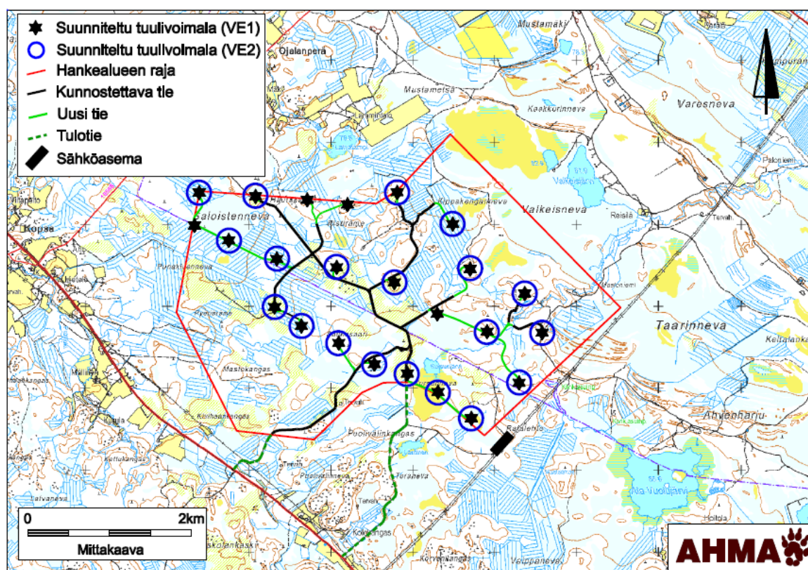
Kuva 4-6. Hankealueelle johtavat tulotiet ja sisäinen tiestö.
