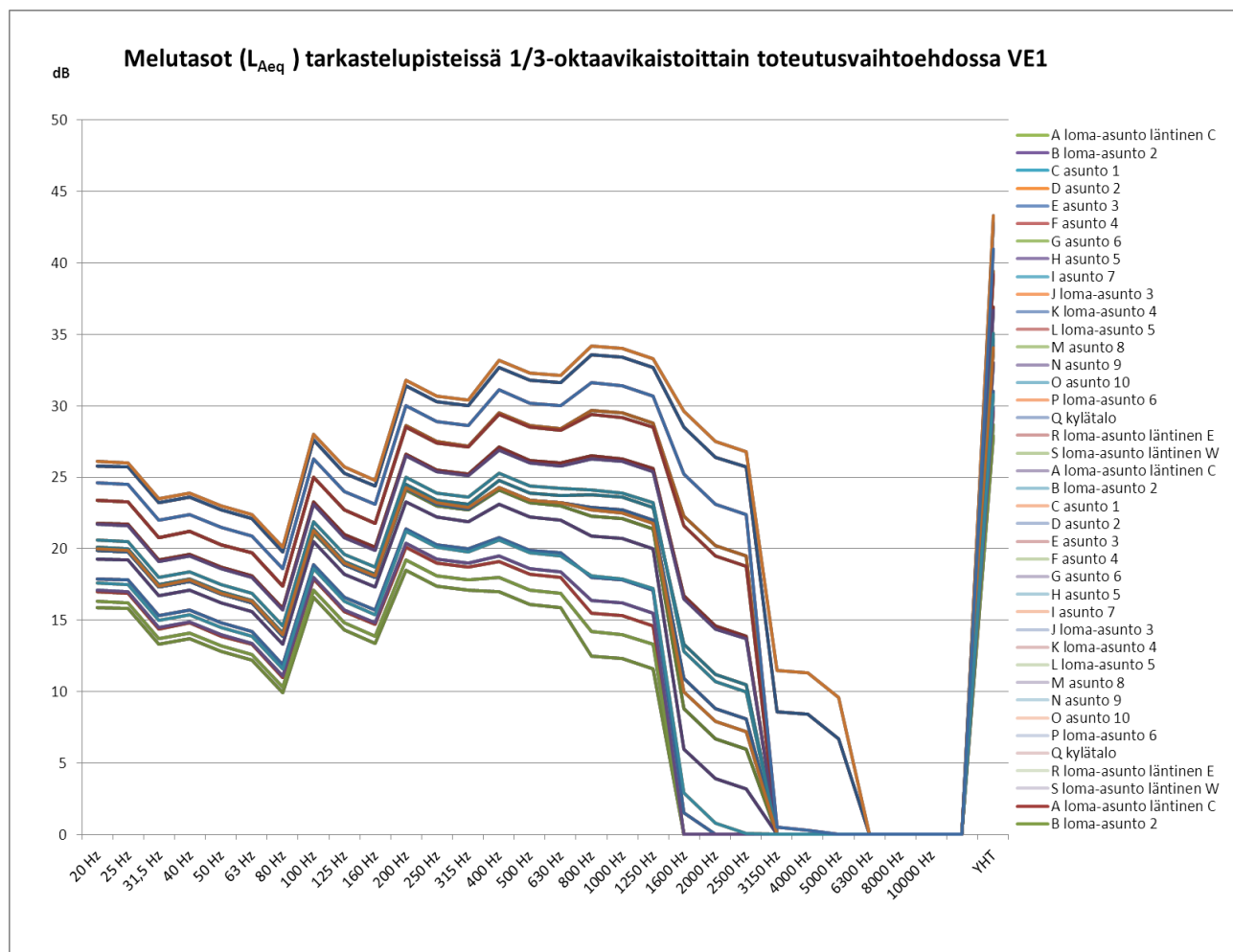
Kuva 7-4. Mastokankaan tuulivoimapuiston aiheuttamat melutasot taajuuskaistoittain vaihtoehdossa VE1.
