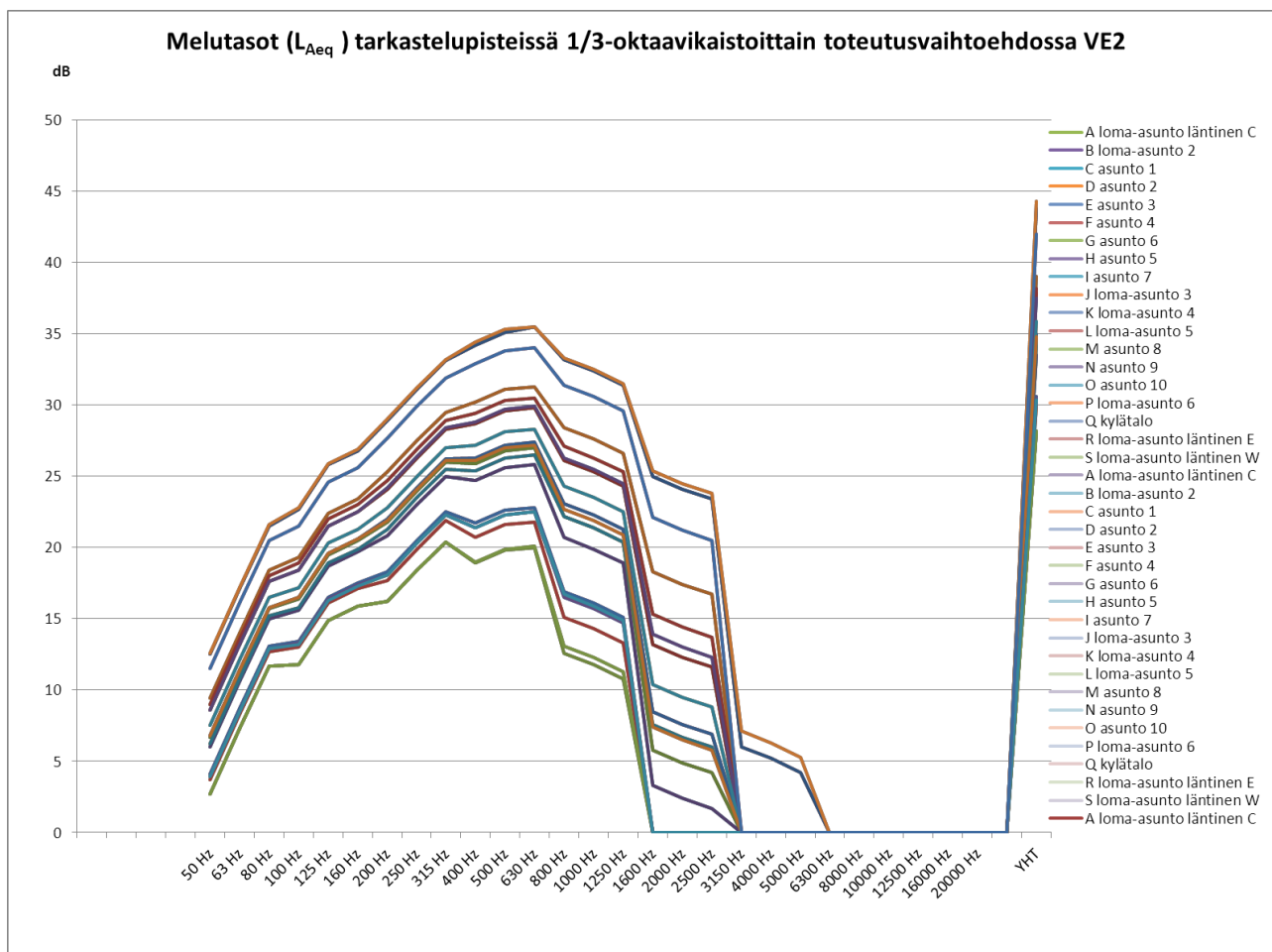
Kuva 7-6. Mastokankaan tuulivoimapuiston aiheuttamat melutasot taajuuskaistoittain vaihtoehdossa VE2.
