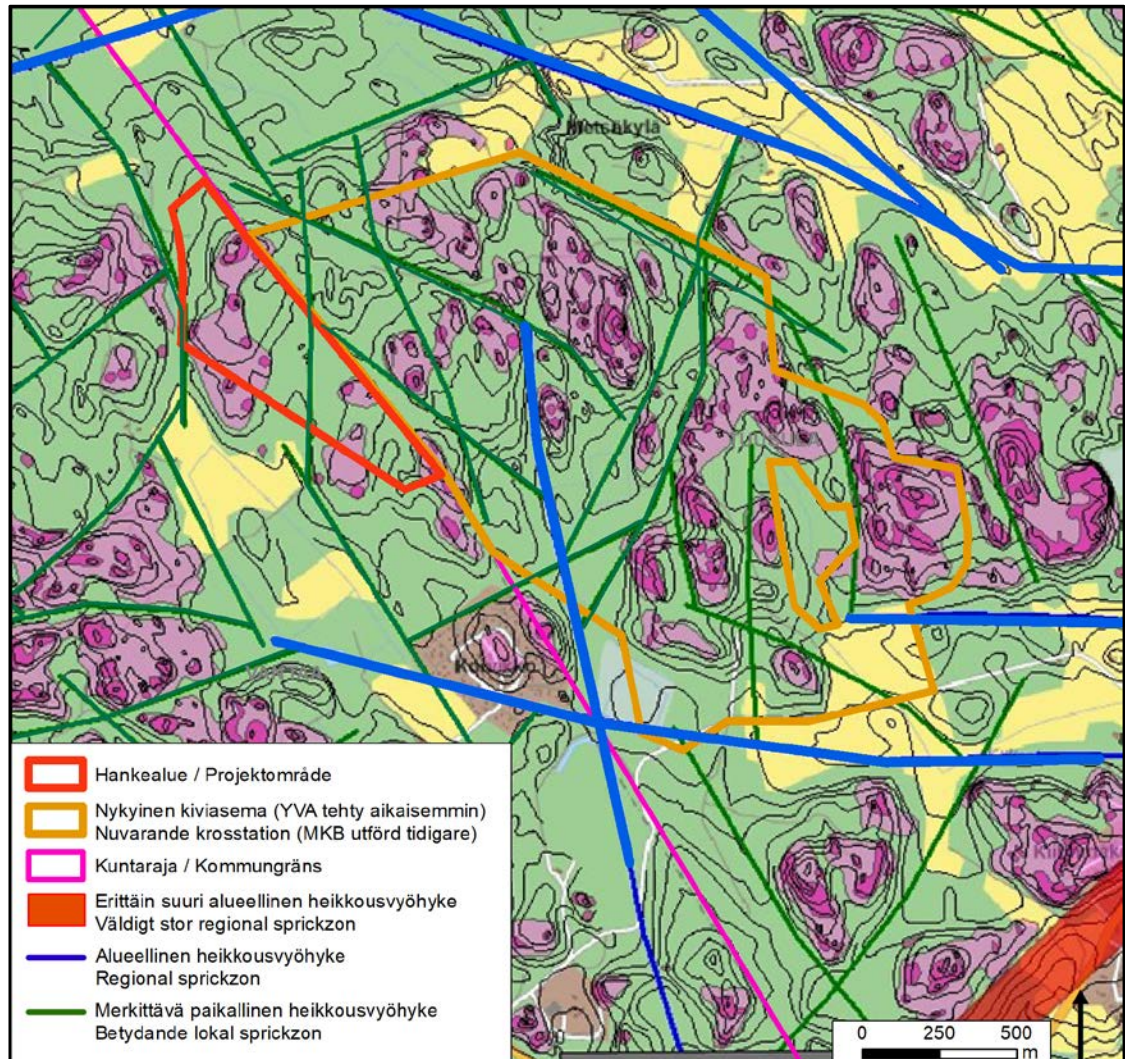
Kuva 5.4. Kallion rakennettavuuskartta. Bild 5.4. Karta över bergets byggbarhet.
