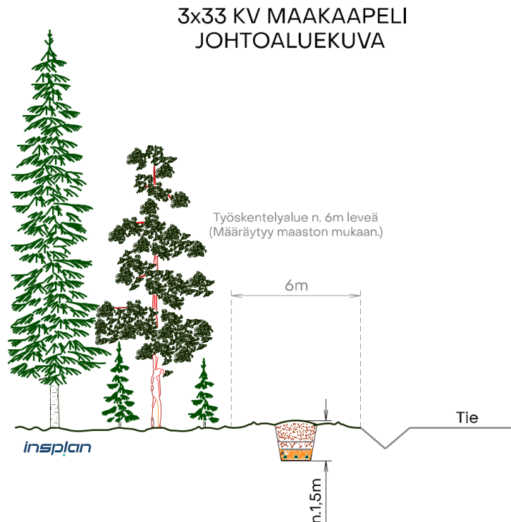
Kuva 9. Reittivaihtoehdossa SVE1b käytettävän 33 kV:n maakaapelin johtoaukean poikkileikkaus (Insplan Oy). Maakaapelin tilantarve on sama niin käytettäessä yhtä kuin useampaa kaapelia.
