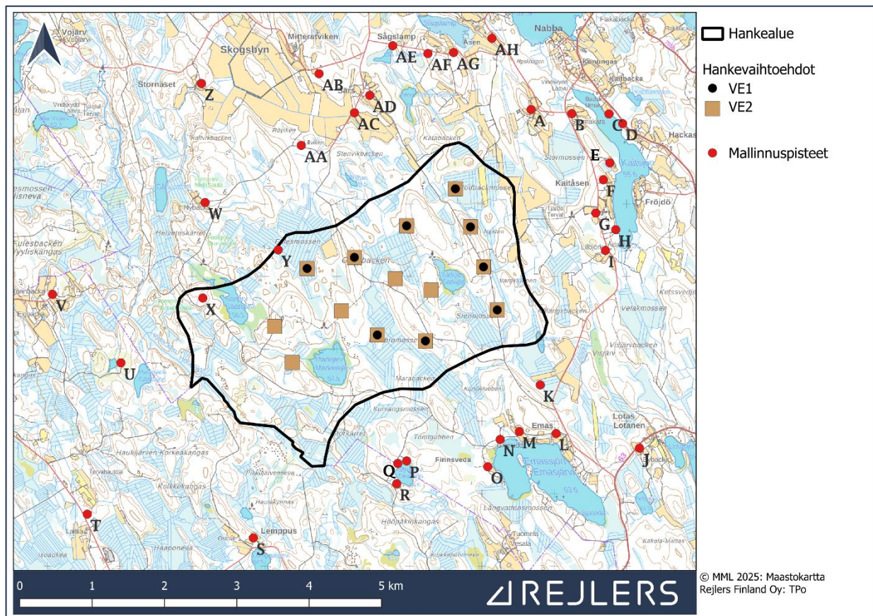
Kuva 74. Mallinnuspisteet, joihin pienitaajuisen sisämelun laskenta toteutettiin.
