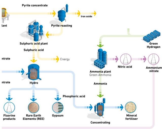
Kuva 6-1. Yleisprosessikaavio suunnitellusta tuotantoprosessista kokonaisuudessaan toteutetusta teollisuuspuistossa. Vertojen eri värit osoittavat laajennuksen eri vaiheita. Toteutusvaihe 1: sininen raide, toteutusvaihe 2: keltainen raide, toteutusvaihe 3: vihreä raide, toteutusvaihe 4: violetti raide.
