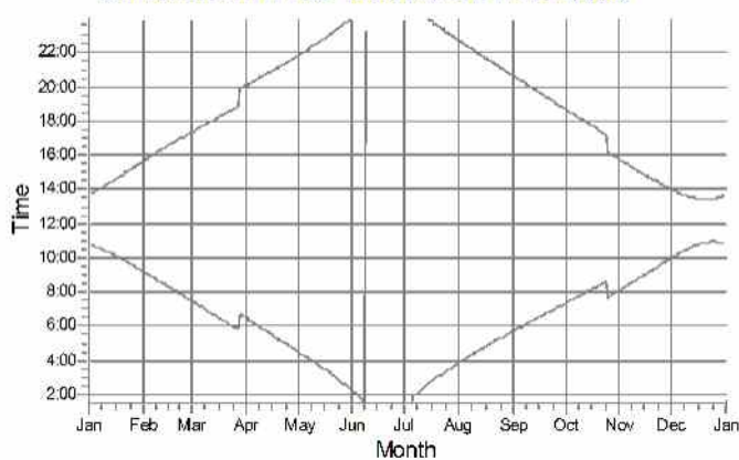
33: NORDEX N117 hub: 120.0 m (TOT: 178.5 m) (33)
