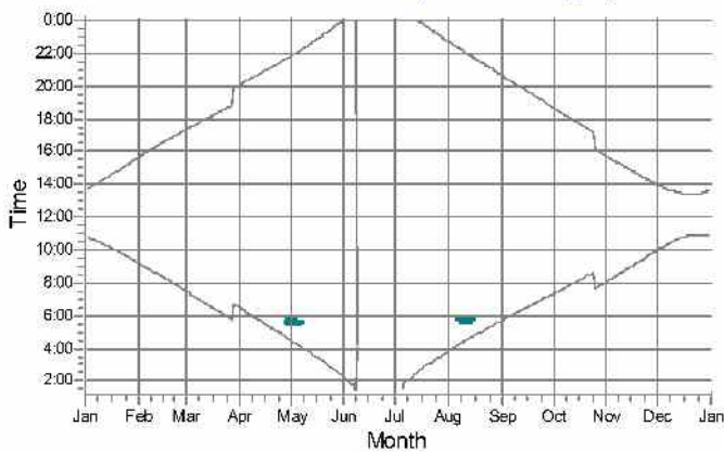
37: NORDEX N117 hub: 120.0 m (TOT: 178.5 m) (37)
