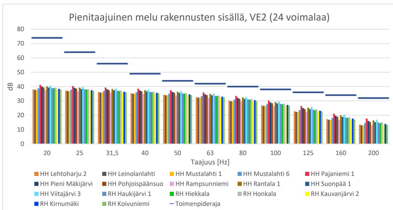
Kuva 10. Pienitaajuisen melun laskentatulokset sisätiloissa suhteutettuna STM:n asumisterveysasetuksen arvoihin. VE2, havaintopisteet 18–34.
