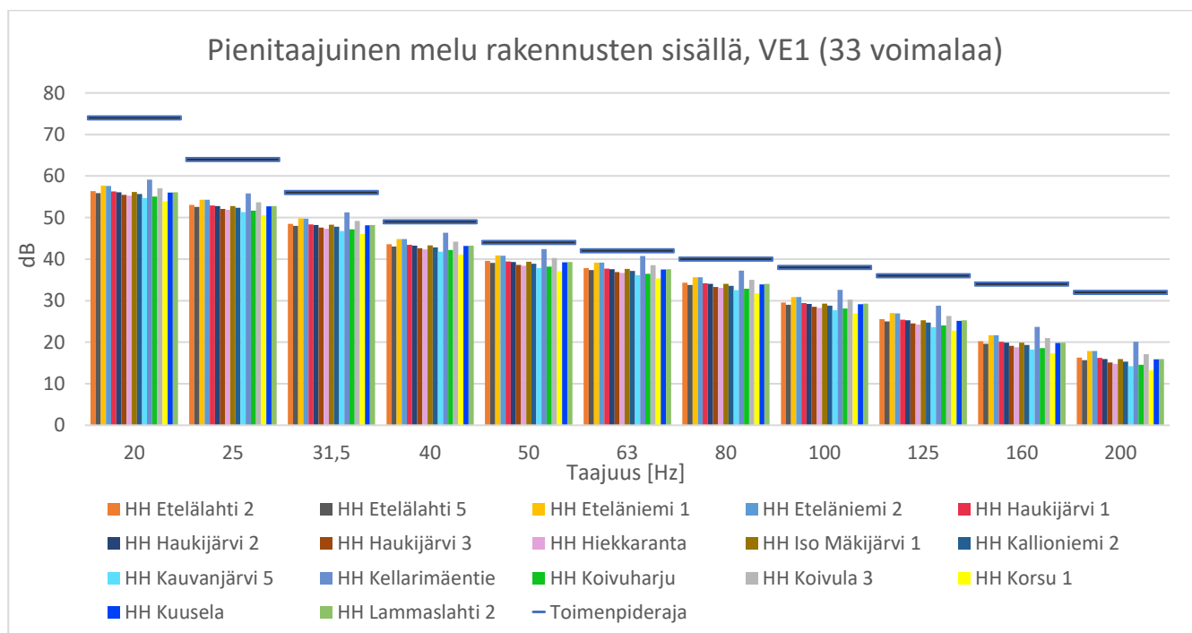
Kuva 1. Pienitaajuisen melun laskentatulokset sisätiloissa suhteutettuna STM:n asumisterveysasetuksen arvoihin. VE1, havaintopisteet 1–17.
