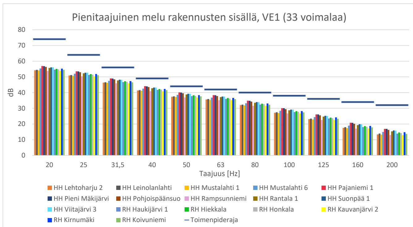
Kuva 2. Pienitaajuisen melun laskentatulokset sisätiloissa suhteutettuna STM:n asumisterveysasetuksen arvoihin. VE1, havaintopisteet 18–34.
