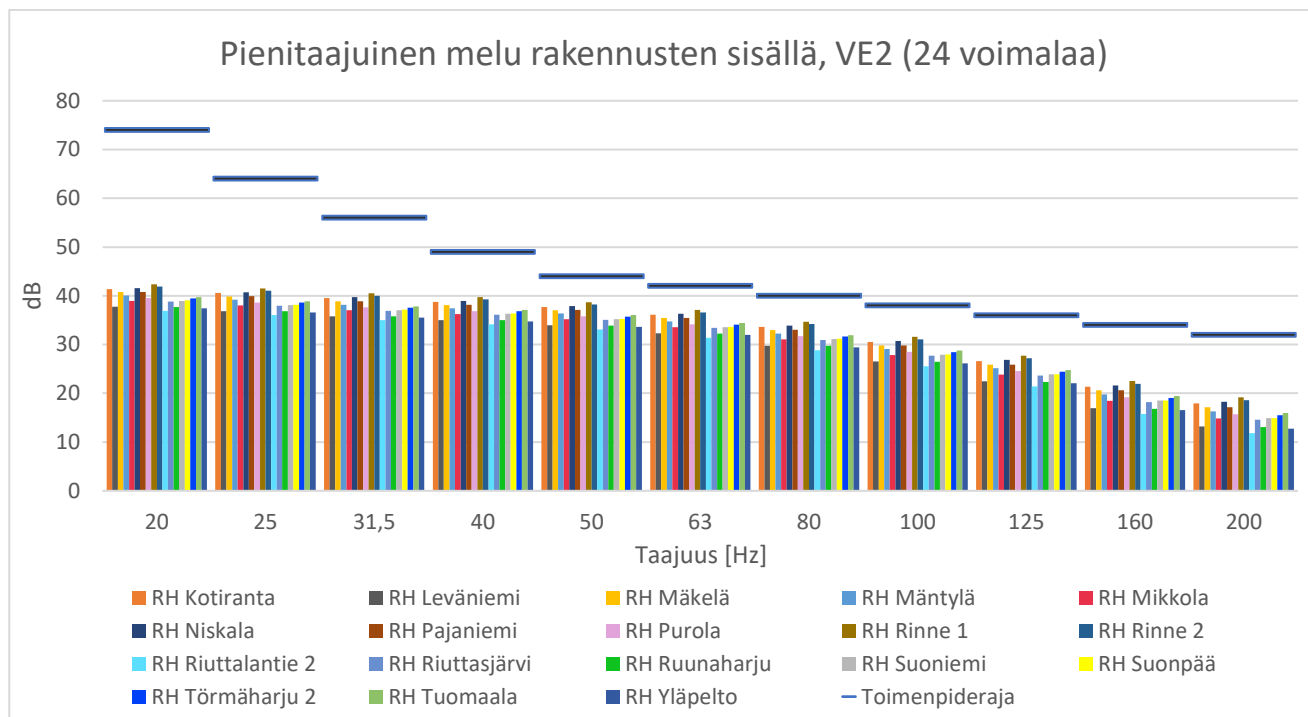
Kuva 11. Pienitaajuisen melun laskentatulokset sisätiloissa suhteutettuna STM:n asumisterveysasetuksen arvoihin. VE2, havaintopisteet 34–52.
