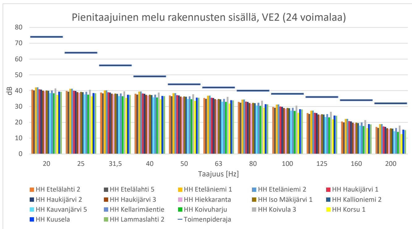
Kuva 4. Pienitaajuisen melun laskentatulokset sisätiloissa suhteutettuna STM:n asumisterveysasetuksen arvoihin. VE2, havaintopisteet 1–17.
