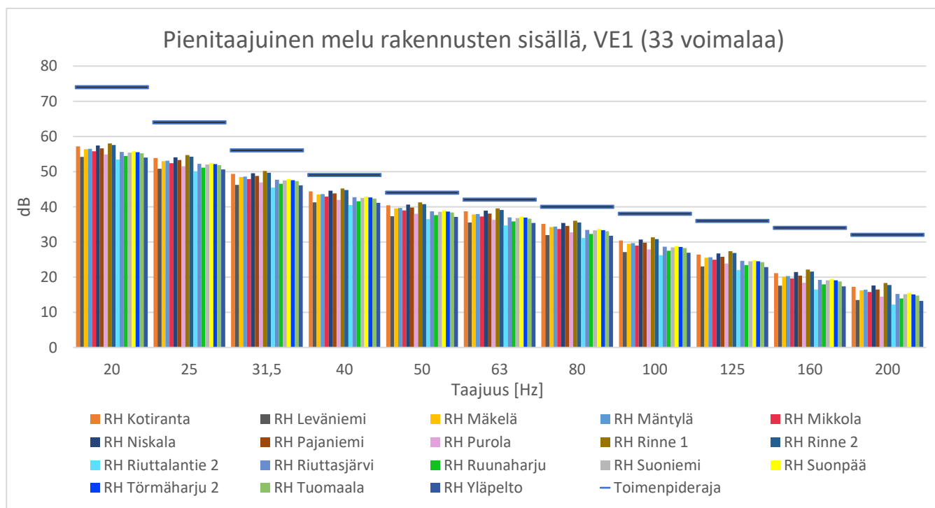
Kuva 3. Pienitaajuisen melun laskentatulokset sisätiloissa suhteutettuna STM:n asumisterveysasetuksen arvoihin. VE1, havaintopisteet 35–52.
