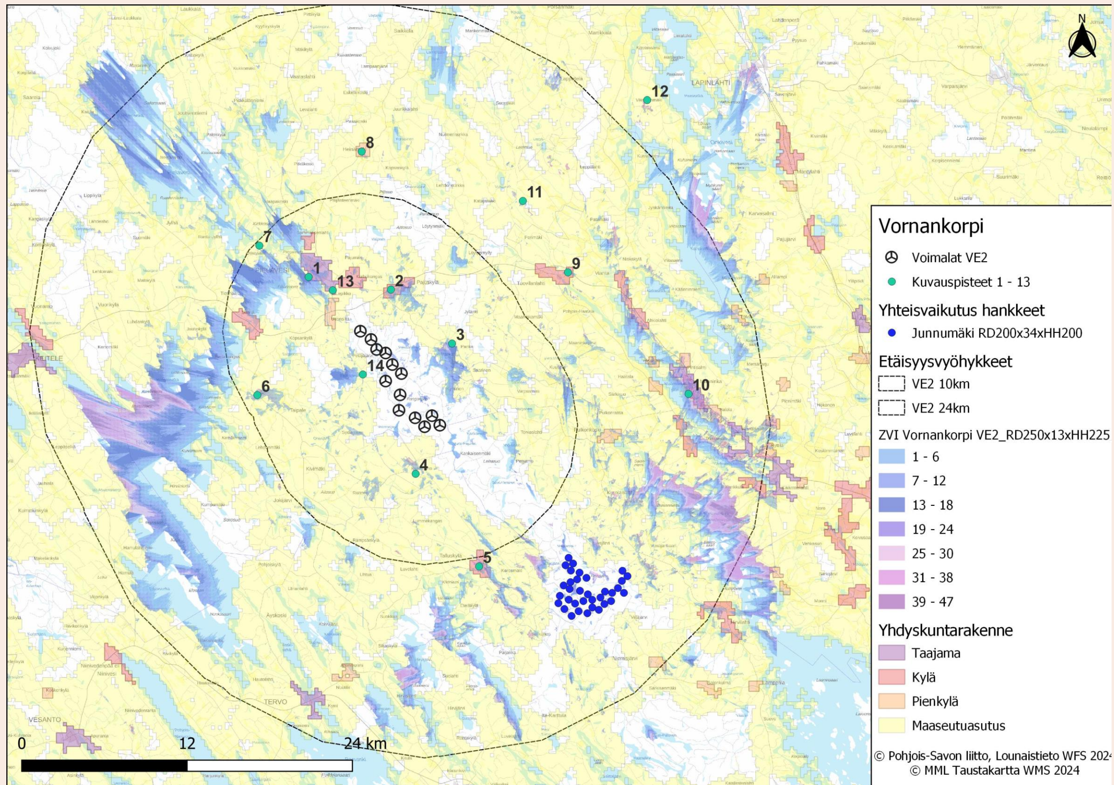
Kuva 12. Vornankorven tuulivoimahankkeen hankevaihtoehtoehdon VE2 näkymäalueanalyysin laskentatulokset voimaloiden Napakorkeudella mallinnettuna yhteisvaikutushankkeen Junnunmäki kanssa. Kuvauspisteet 1–13 sekä näkymäalueanalyysin mallinnusalueen yhdyskuntarakenne.
