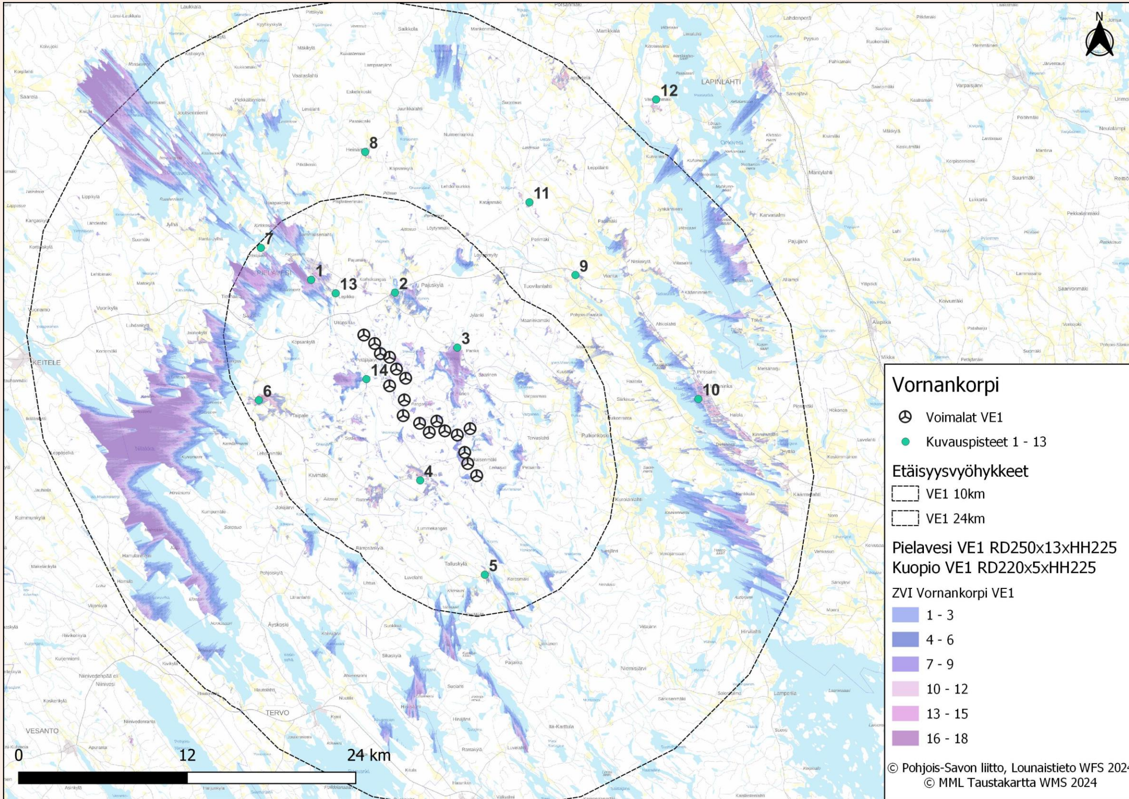
Kuva 1. Vornankorven tuulivoimahankkeen hankevaihtoehdon VE1 näkymäalueanalyysin laskentatulokset voimaloiden napakorkeudella mallinnettuna. Voimaloiden napakorkeus on Pielaveden ja Kuopion puolella 225 metriä. Kuvauspisteet 1–13.
