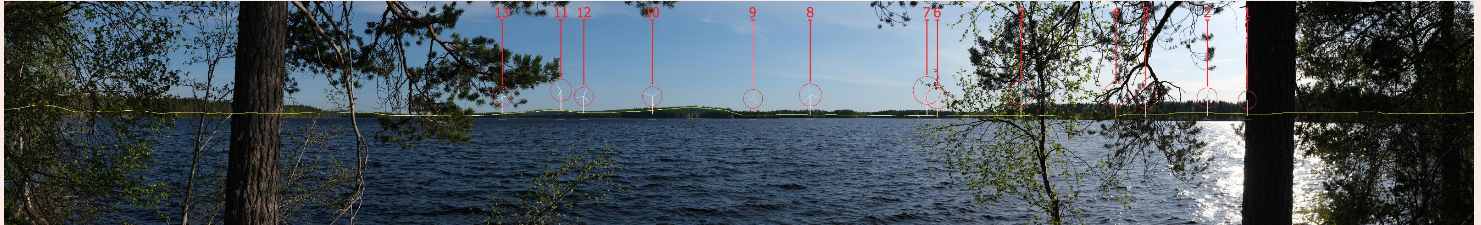
Kuva 25. Valokuvasovite kuvauspisteestä 3 hankevaihtoehdossa VE2 on otettu Iso-Panka-järven pohjoisosasta. Etäisyys lähimpiin Vornankorven voimaloihin on noin 4,3 kilometriä. Vornankorven tuulivoimalat on numeroitu ja roottoriympyrä korostettu punaisella.
