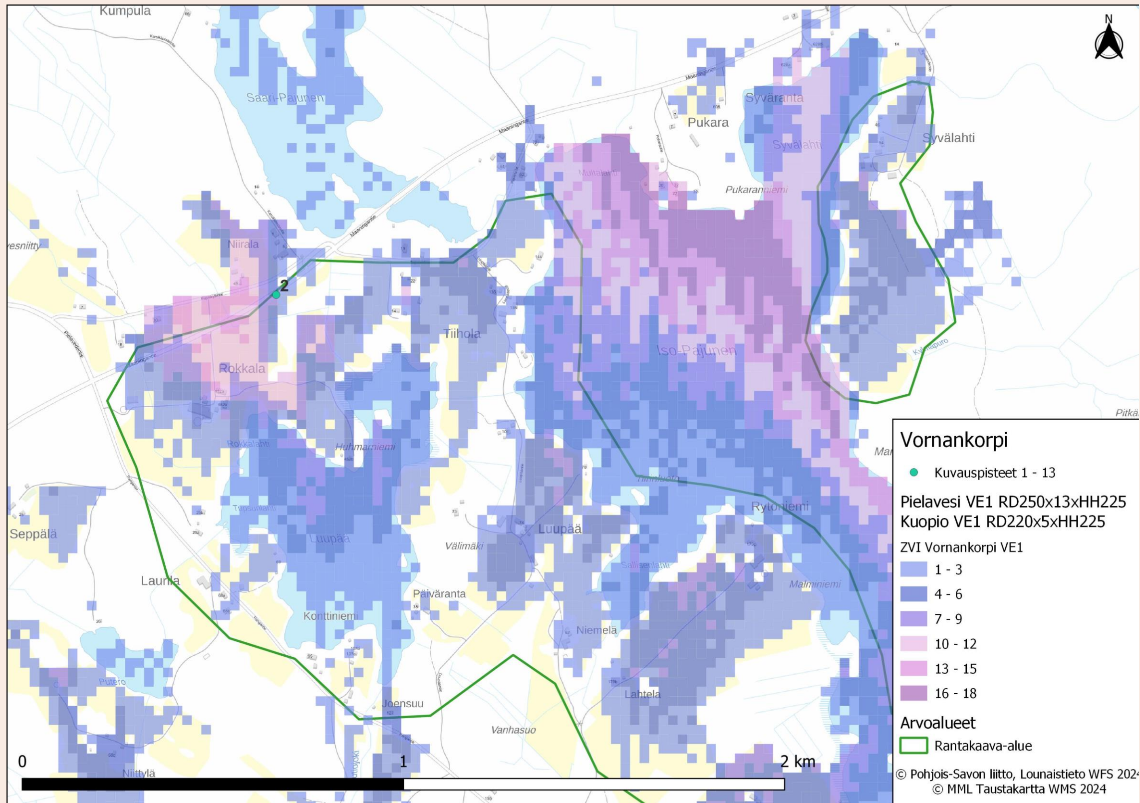
Kuva 17. Kuvauspaikka 2 Pielaveden Pajuskylässä. Näkymäalueanalyysi hankevaihtoehdosta VE1.
