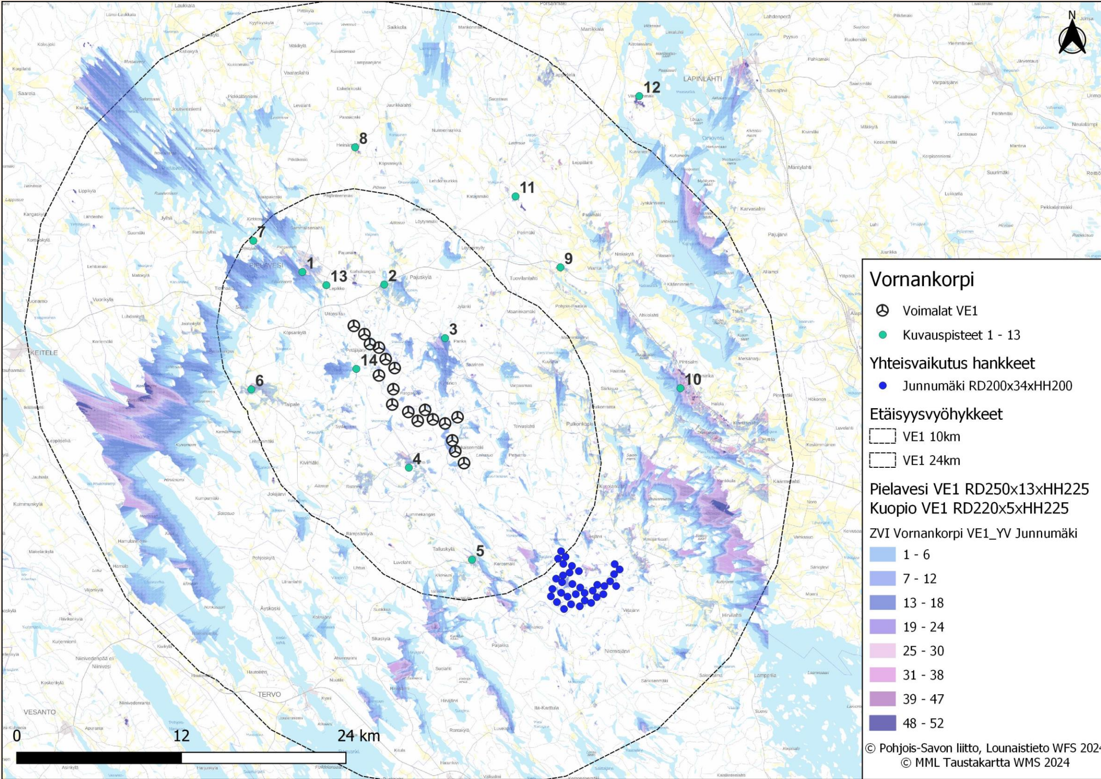
Kuva 2. Vornankorven tuulivoimahankkeen hankevaihtoehdon VE1 näkymäalueanalyysin laskentatulokset voimaloiden napakorkeudella mallinnettuna yhteisvaikutushankkeen Junnumäki kanssa. Junnumäen voimaloiden napakorkeus on 200 metriä. Kuvauspisteet 1–13.
