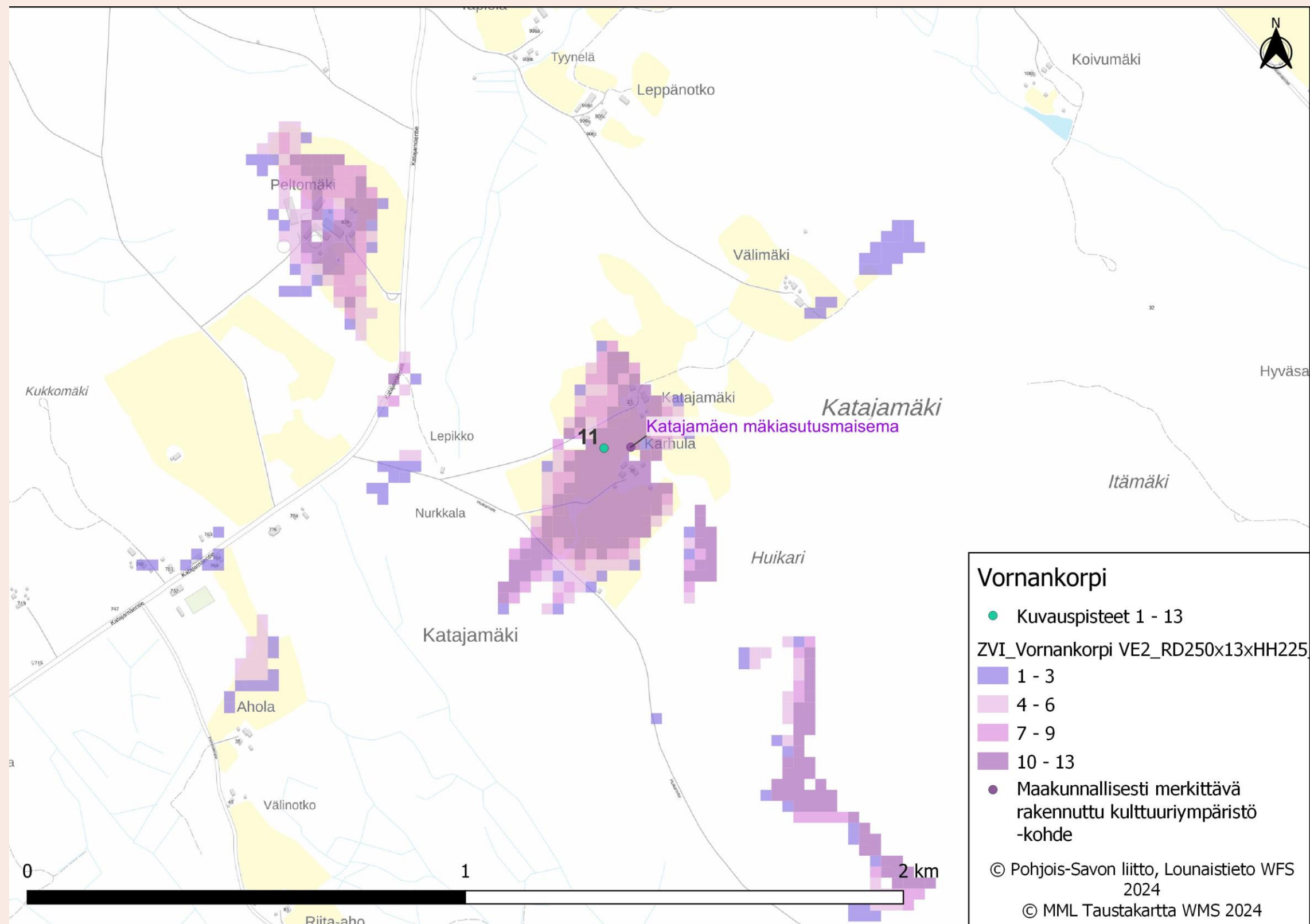
Kuva 68. Kuvauspaikka 11 Pielaveden Katajamäki. Näkymäalueanalyysi hankevaihtoehdosta VE2.
