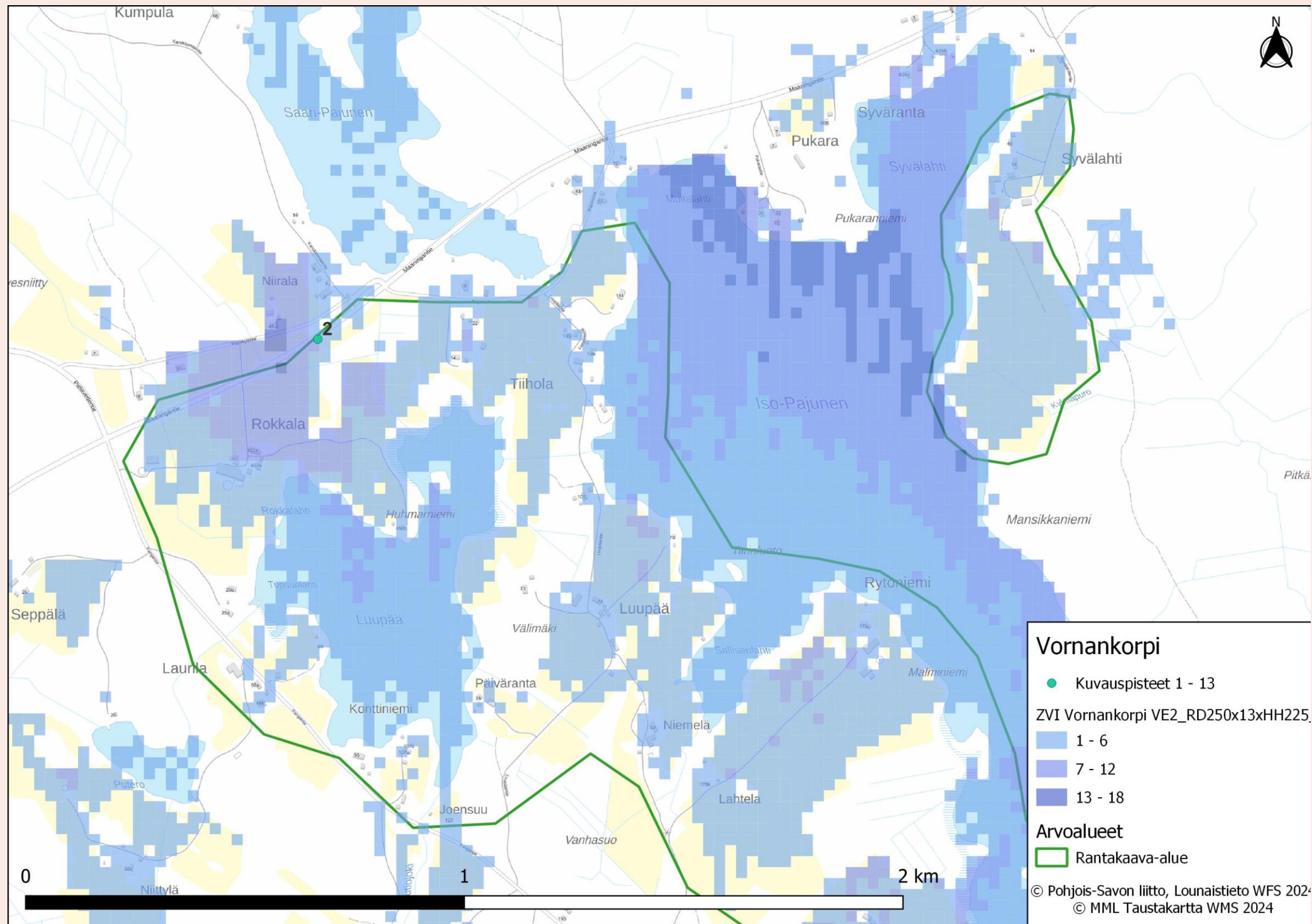
Kuva 92. Kuvauspaikka 2 Pielaveden Pajuskylässä. Näkymäalueanalyysissä hankevaihtoehdosta VE2 on huomioitu Junnunmäen suunniteltu tuulivoimahanke.
