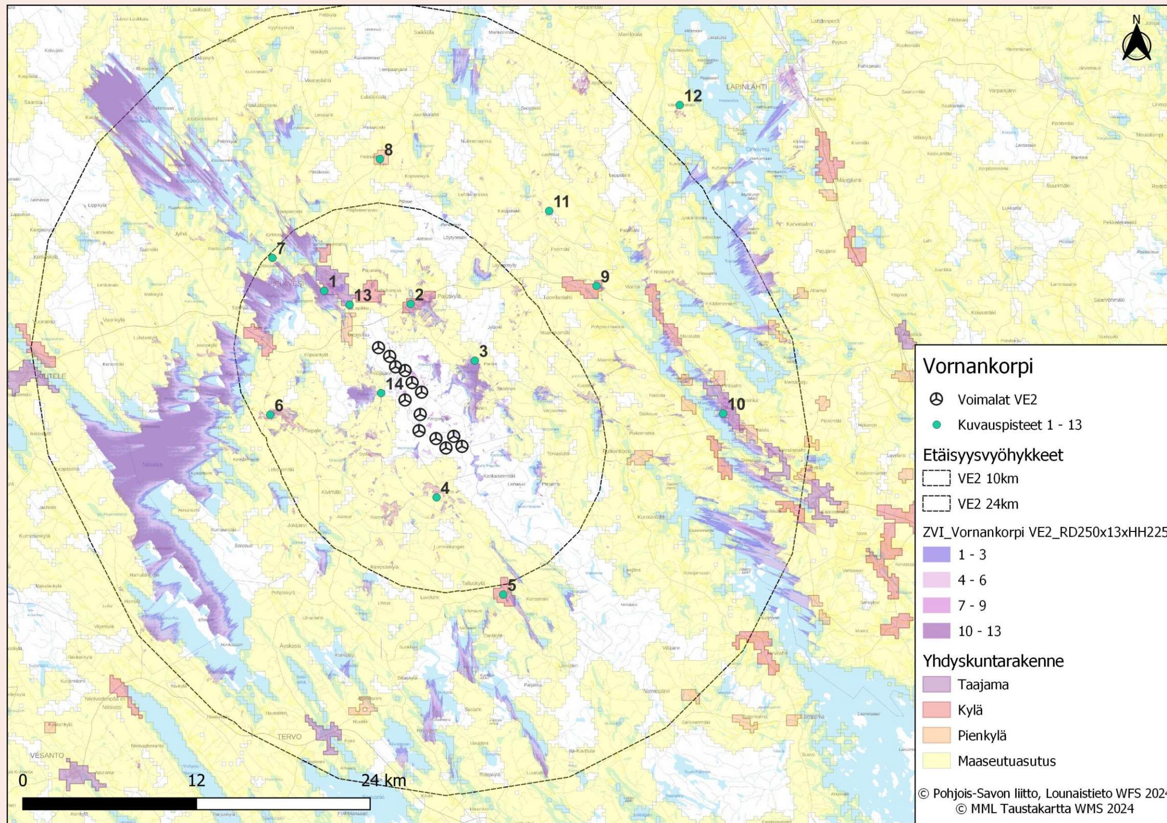
Kuva 11. Vornankorven tuulivoimahankkeen hankevaihtoehto VE2 näkymäalueanalyysin laskentatulokset voimaloiden napakorkeudella mallinnettuna. Voimaloiden napakorkeus on 225 metriä. Kuvauspisteet 1–13 sekä näkymäalueanalyysin mallinnusalueen yhdyskuntarakenne.
