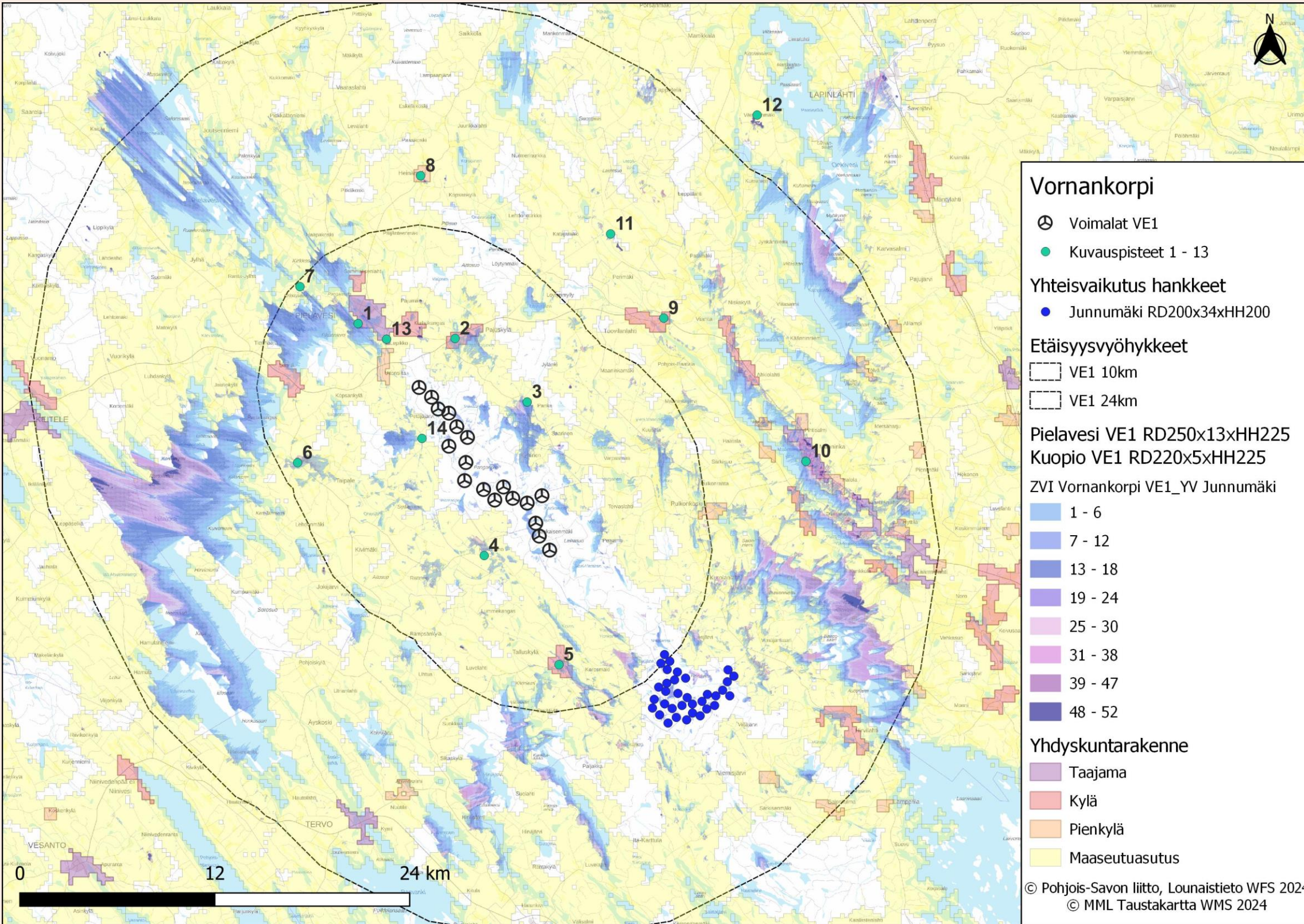
Kuva 6. Vornankorven tuulivoimahankkeen hankevaihtoehdon VE1 näkymäalueanalyysin laskentatulokset voimaloiden napakorkeudella mallinnettuna yhteisvaikutushankkeen Junnumäki kanssa. Kuvauspisteet 1–13 sekä näkymäalueanalyysin mallinnusalueen yhdyskuntarakenne.
