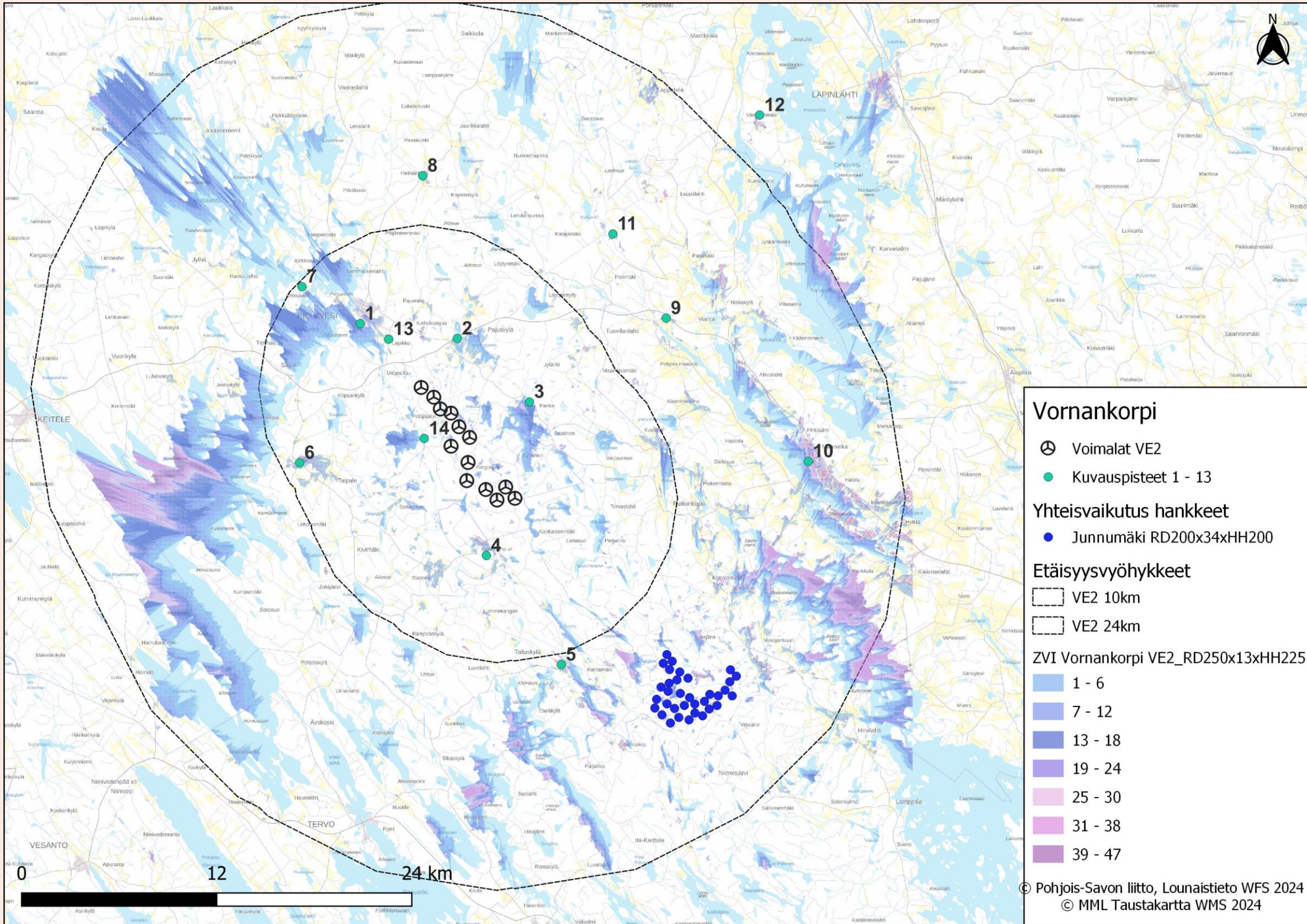
Kuva 8. Vornankorven tuulivoimahankkeen hankevaihtoehdon VE2 näkymäalueanalyysin laskentatulokset voimaloiden Napakorkeudella mallinnettuna yhteisvaikutushankkeen Junnumäki kanssa. Junnumäen voimaloiden napakorkeus on 200 metriä. Kuvauspisteet 1–13.
