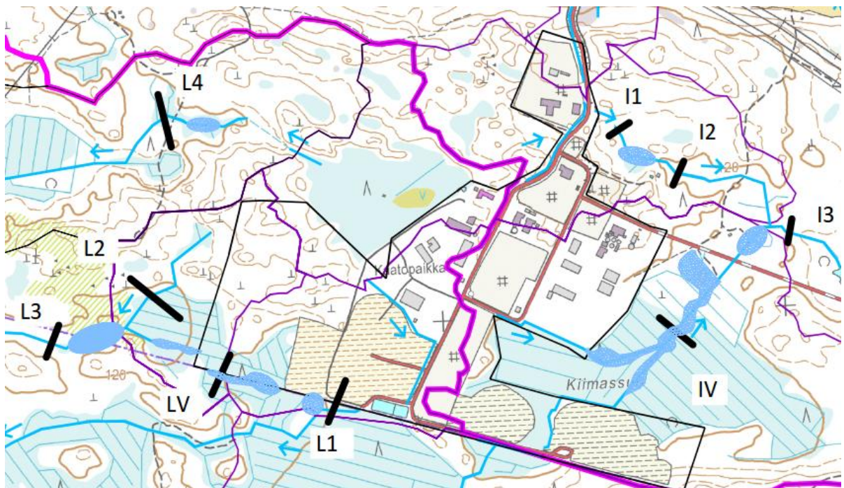
Kuva 2. Envitech -selvityksessä suositellut purku-uoman poikkileikkaukset, Ramboll 2013.
