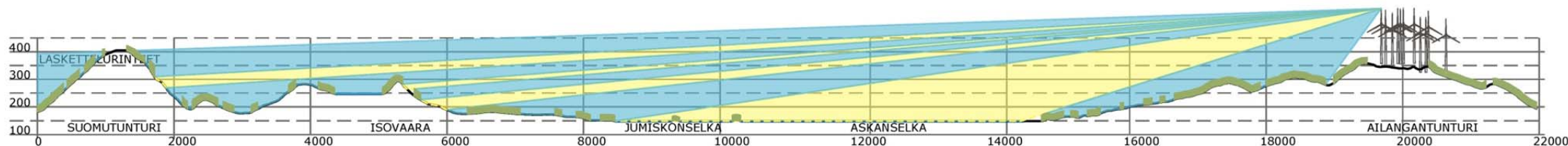
Kuva 13. Poikkileikkauskuva B – B Suomutunturilta Ailangantunturiin. Tuulivoimalat näkyvät keltaisilta näkemäsektoreilta, eli käytännössä pidemmiltä järvenselkäalueilta ja vaarojen Ailanganpuoleisilta rinteiltä. Sinisillä näkemäsektoreilla maastonmuodot ja puusto estävät suorat näkymät tuulivoimaloille. Suomun matkailukeskuksesta ja rinteiltä ei ole näköyhteyttä Ailangantunturin tuulivoimaloille, ihan Suomutunturin laelta voi puiden välistä erottaa yksittäisiä tuulivoimaloita kaukomaisemassa.
