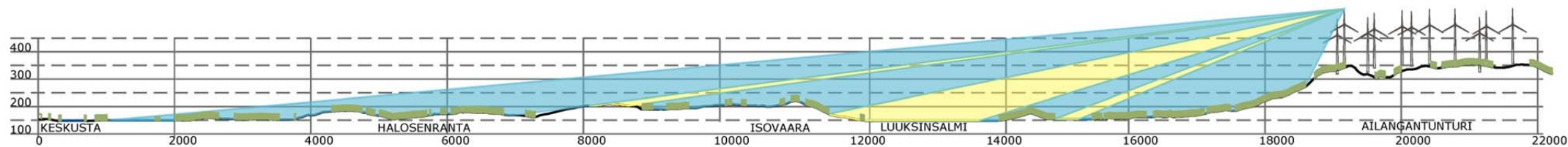
Kuva 12. Poikkileikkauskuva A – A Kemijärven keskustasta Ailangantunturiin. Tuulivoimalat näkyvät keltaisilta näkemäsektoreilta, eli käytännössä pidemmiltä järvenselkäalueilta ja vaarojen Ailanganpuoleisilta rinteiltä. Sinisillä näkemäsektoreilla maastonmuodot ja puusto estävät suorat näkymät tuulivoimaloille.
