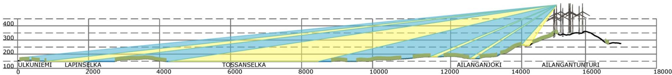
Kuva 14. Poikkileikkauskuva C – C Ulkuniemestä Ailangantunturiin. Tuulivoimalat näkyvät keltaisilta näkemäsektoreilta, eli käytännössä pidemmiltä järvenselkäalueilta. Sinisillä näkemäsektoreilla maastonmuodot ja puusto estävät suorat näkymät tuulivoimaloille.
