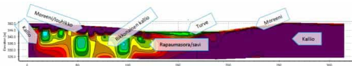
Kuva 3-8. Esimerkki alueen 3 (Kuva 3-7) maavastusluotauksen tuloksesta. Tulokset on esitetty pitkin mittaussuuntaa topografiaan sidottuina pystyinä n. 20 m korkeina leikkauskuvina, joissa sähköinen ominaisvastus on värikoodattu. Tumman punaruskeat sävyt edustavat korkeaa ominaisvastusta (kuiva moreeni tai louhikko, kiinteä kallio). Turve, kuivan kerroksen alapuolinen moreeni, tai rapakallio on esitetty keltaisen ja vihreän sävyin, jotka rikkonaisen kallion kohdalla yltyvät leikkauksen pohjalle saakka.
