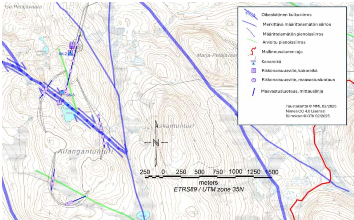
Kuva 4-7. Siirroksiin liittyvien rikkonaisuusvyöhykkeiden havaintoja kairausten ja maavastusluotausten perusteella pumppuvoimalan yläaltaan ja teknisten tilojen alueella.
