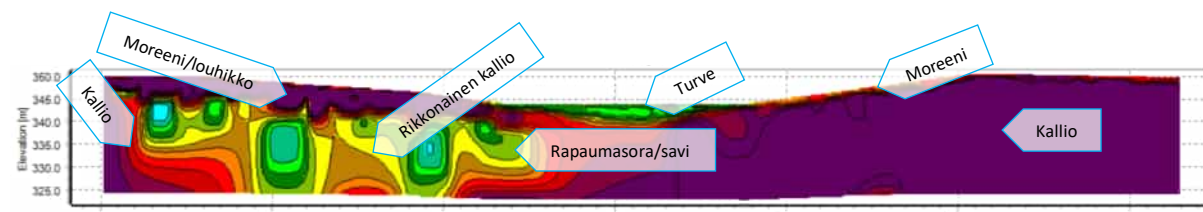
Kuva 5 Alue 3 -tulospystyleikkauksen X-akseli kuvaa maan päällä olevan mittauslinjan pituutta metreinä ja Y-akseli mittauksen syvyyttä metreinä. Mittauksen alkupisteen (kuvan vasen reuna) koordinaatit: 526203.8227 (X), 7379110.679 (Y), 349,82 (Z). Mittauksen loppupisteen (kuvan oikea reuna) koordinaatit: 526490.9357 (X), 7379229.9094 (Y), 349,5 (Z).
