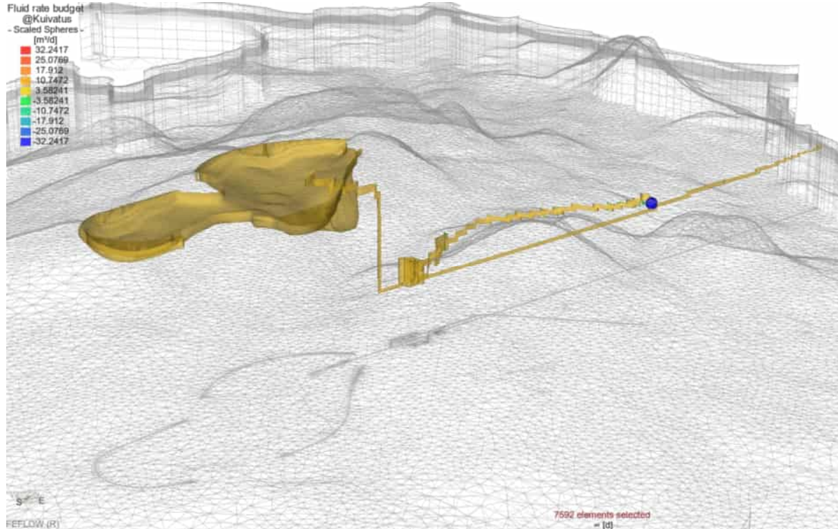
Kuva 6-13. Pohjaveden suotautumisen jakautuminen tunneliseinämälle, pallon koko ja väri kuvaa pohjaveden suotautumisen määrää. Kun tunnelia leikkaavat ruhjeet on tiivistetty, pohjavettä suotautuu tunneleihin eniten sisäänmenoaukon kohdalla.
