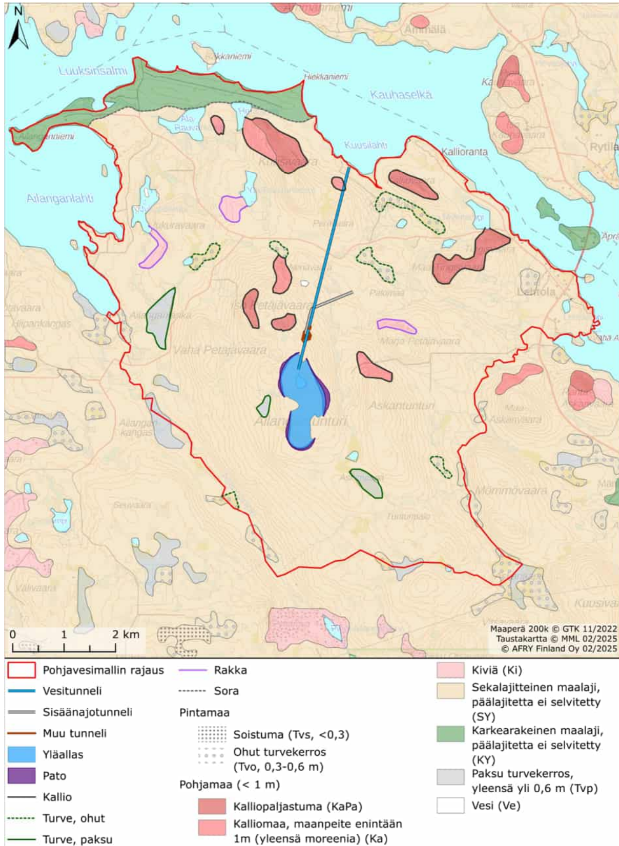
Kuva 5-3. Maaperäkartaan perustuvat malliin määritellyt turve- (ohut ja paksu kerros), moreeni-, sora- ja kallioalueet.
