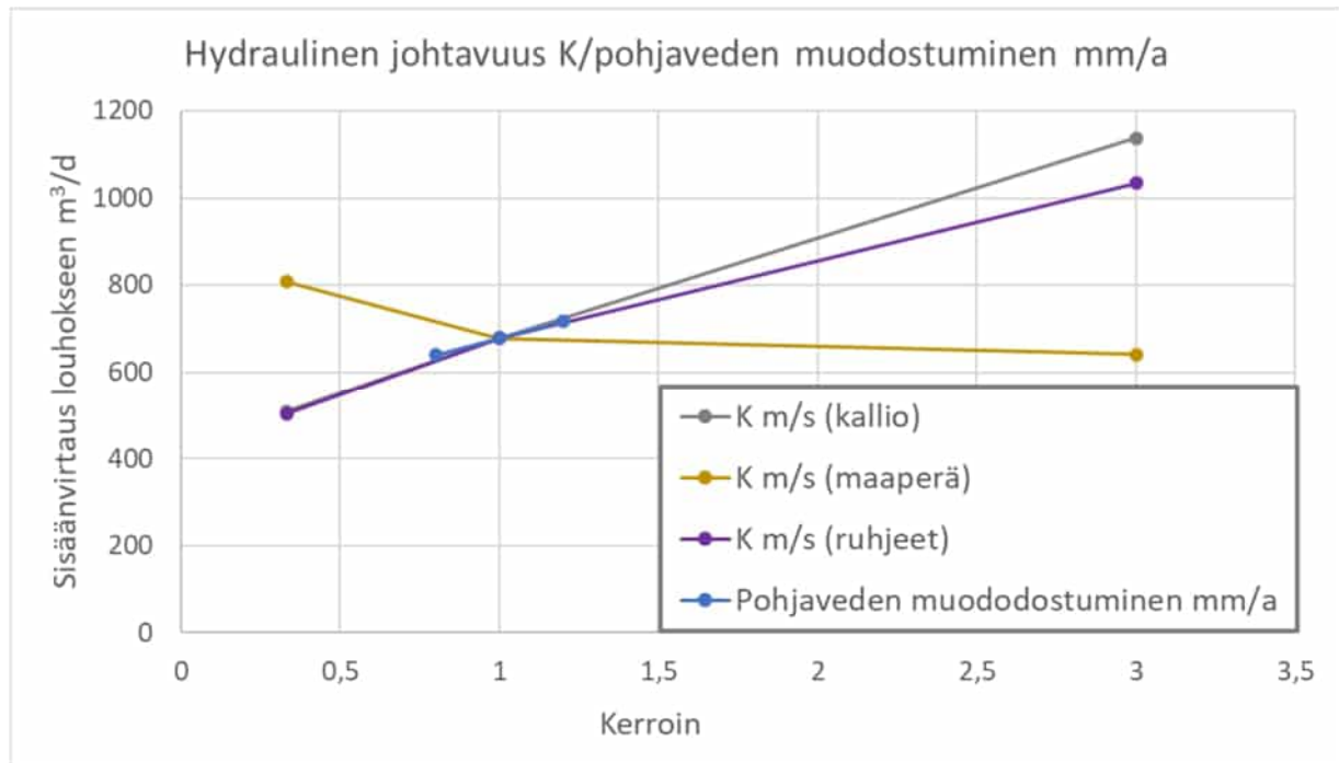
Kuva 6-14. Hydraulisen johtavuuden herkkyyssanalyysi toiminta-ajan (simulointi 1) mallissa. Kuivatettavien tunneleiden ja tilojen suotovesimäärän vaihtelu, kun ruhjeille, kalliolle ja maaperälle asetettuja hydraulisen johtavuuden arvoja suurennettiin tai pienennettiin kertoimella 3 tai pohjaveden muodostumisen määrää muutettiin kertoimella 0,8 tai 1,2 (20 %).
