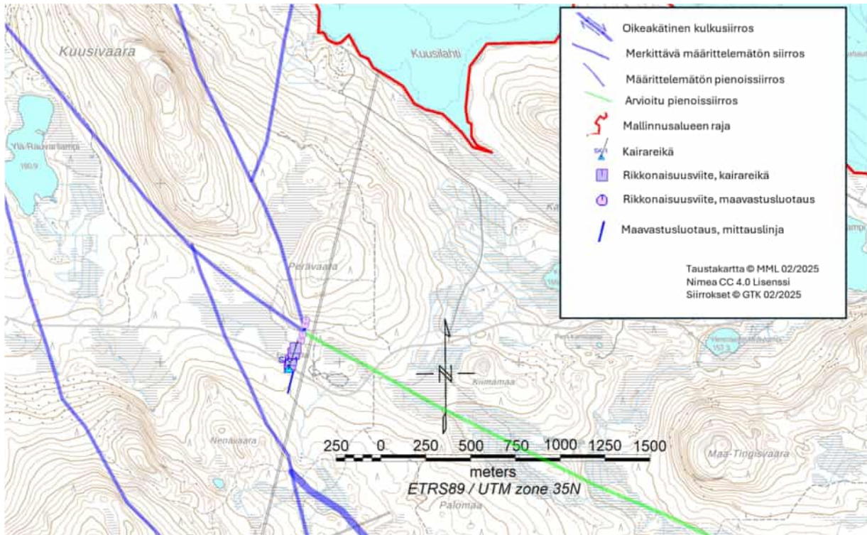
Kuva 4-8. Siirroksiin liittyvien rikkonaisuusvyöhykkeiden havaintoja kairausten ja maavastusluotausten perusteella pumppuvoimalan alavesitunnelin alueella.
