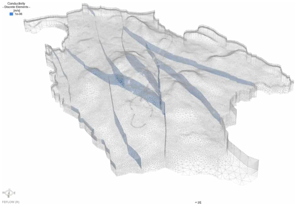
Kuva 5-5. Mallissa mukana olevat alueelliset ruhjevyöhykkeet.
