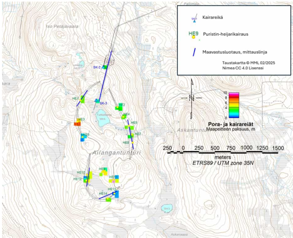
Kuva 4-13. Porauksiin ja kallionäytekairausten maaputken pituuksiin perustuvat maapeitteen paksuustiedot Ailangantunturin ylävesialtaan ja teknisten tilojen alueella. Pistemäisiä havaintoja ei ole interpoloitu.
