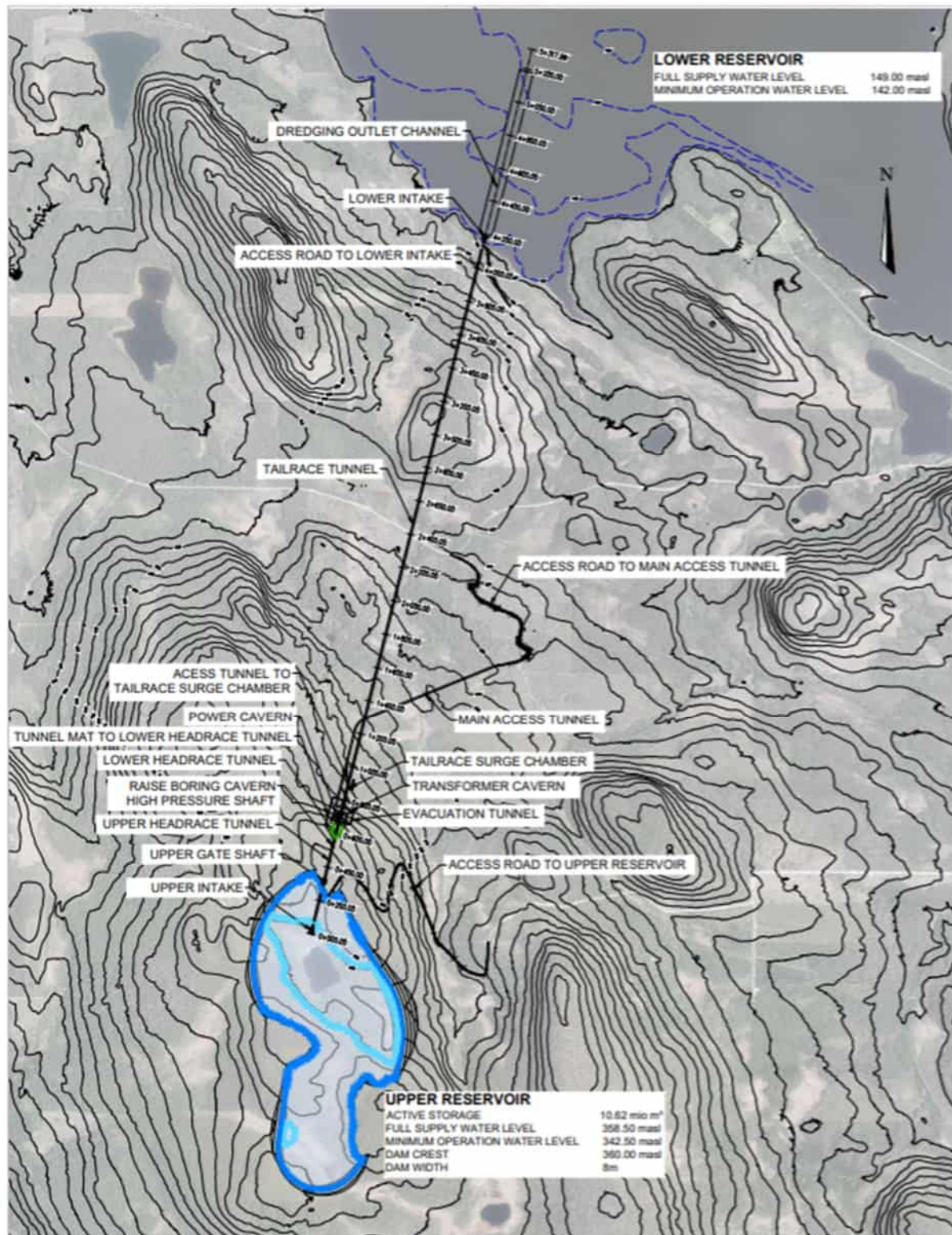
Kuva 4-25. Pumppuvoimala (KEM-AIL-CS-GE-001-002.dwg).
