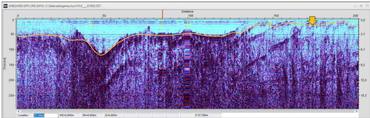
Kuva 4-17. Esimerkki maatulokaluotauksen tuloksesta, Linja 1 (paaluväli 2500–2700 m). Oranssi viiva esittää tulkitun kalliopinnan asemaa. Nuoli osoittaa porauksessa havaittua kalliota. Vasemmalla on alueella tyypillistä ohutta sedimenttikerrosta kallon päällä, paaluvälillä 50–130 m turvekerros (suo) ja sen alla mahdollisesti kalliorikkonaisuutta. Oikeassa reunassa maakerros on ohut. Loivakaateiset heijastukset ovat jatkuvia kalliorakoja.
