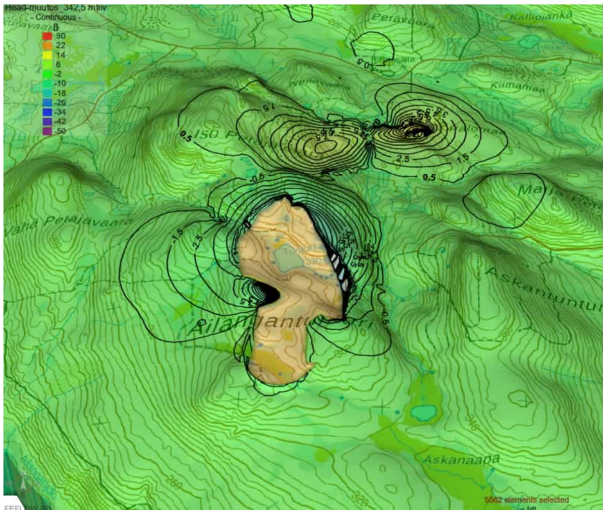
Kuva 6-11. Pohjavedenpinnan muutos pumppuvoimalaitoksen toiminnan aikana nykytilaan verrattuna, kun vesivarastoaltaan vesipinta on 342,5 m (N43), a) 2D esitys ja b) 3D esitys. Aiotunnelin ja konetilojen ympärillä pohjavesipinta laskee kuivatuspumppauksen seurauksena ja ylävesivarastoaltaan alueella pohjavesipinta nousee. +/-0,5 m tasa-arvonkäyrät rajaavat alueen, jonka ulkopuolella pohjavesipinnan muutos on pienempi kuin 0,5 m.
