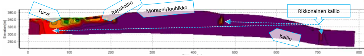
Kuva 7 Alue 5 -tulospystyleikkauskuvan X-akseli kuvaa maan päällä olevan mittauslinjan pituutta metreinä ja Y-akseli mittauksen syvyyttä metreinä. Mittauksen alkupisteen (kuvan vasen reuna) koordinaatit: 526219.0053 (X), 7380660.7697 (Y), 341,47 (Z). Mittauksen loppupisteen (kuvan oikea reuna) koordinaatit: 526398,511 (X), 7381408.065 (Y), 307,5 (Z).
