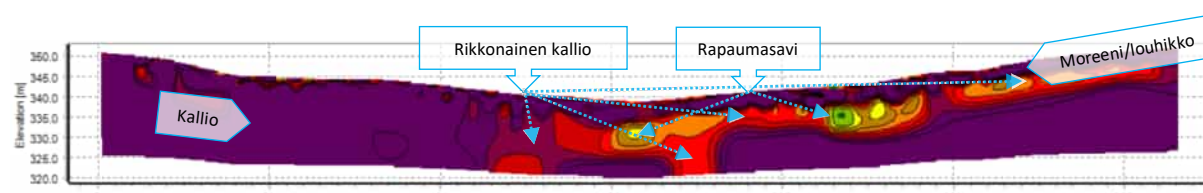
Kuva 4 Alue 2 -tulospystyleikkauksen X-akseli kuvaa maan päällä olevan mittauslinjan pituutta metreinä ja Y-akseli mittauksen syvyyttä metreinä. Mittauksen alkupisteen (kuvan vasen reuna) koordinaatit: 525849.1332 (X), 7380564.4141 (Y), 350,95 (Z). Mittauksen loppupisteen (kuvan oikea reuna) koordinaatit: 526024.1199 (X), 7380817.2725 (Y), 352,08 (Z).
