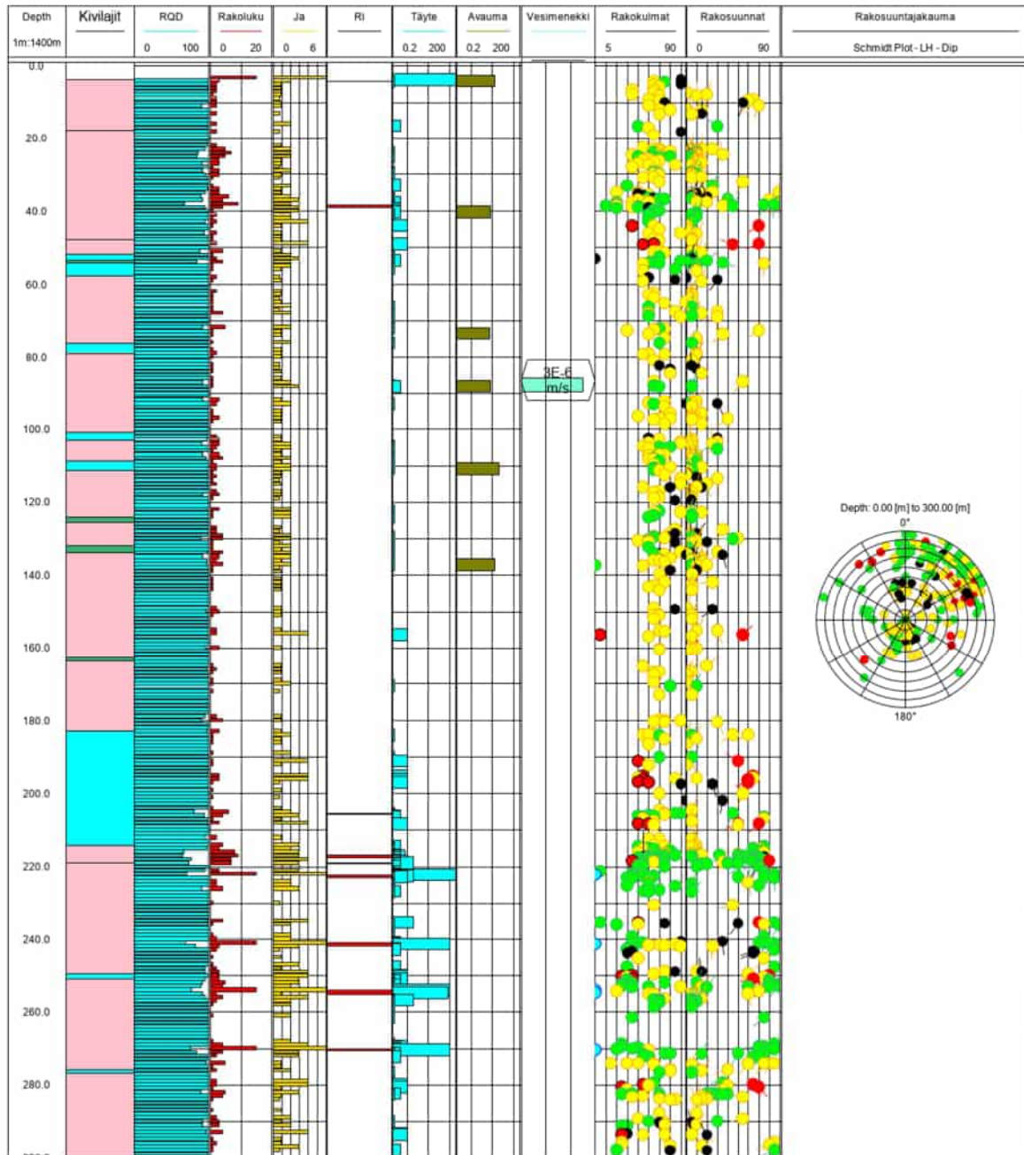
Kuva 3-4. Kairarejän SK-2 kairaustulosten yhteenveto (Mitta Oy 2025).
