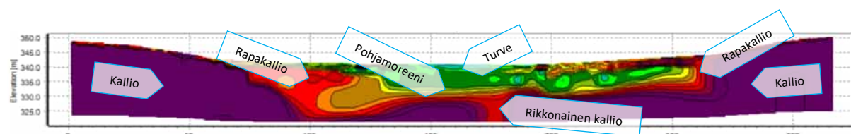
Kuva 6 Alue 4 -tulospystyleikkauksen X-akseli kuvaa maan päällä olevan mittauslinjan pituutta metreinä ja Y-akseli mittauksen syvyyttä metreinä. Mittauksen alkupisteen (kuvan vasen reuna) koordinaatit: 526026.7926 (X), 7379297.9894 (Y), 348,87 (Z). Mittauksen loppupisteen (kuvan oikea reuna) koordinaatit: 526068.5947 (X), 7379606.9562 (Y), 350,47 (Z).
