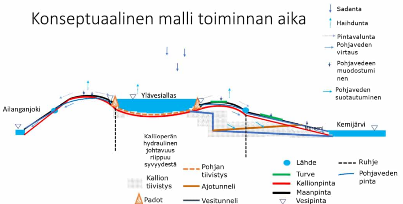
Kuva 4-29. Hydrogeologinen Ailangantunturin suunnitellun pumppuvoimalaitoksen alueen konseptualisointi numeerista mallinnusta varten esitettynä kaavamaisena poikkileikkauksena a) nykytilanteella ja b) toiminnan aikaiselle tilanteelle.
