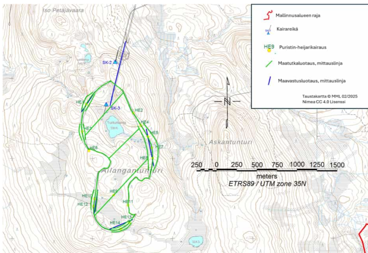
Kuva 4-10. Kalliotopografian mallin luonnissa käytetyt pohjatutkimusten sijainnit, puristin-heijarikairaukset, kallionäytekairaukset, maavastusluotaukset ja maatulkuutaukset.
