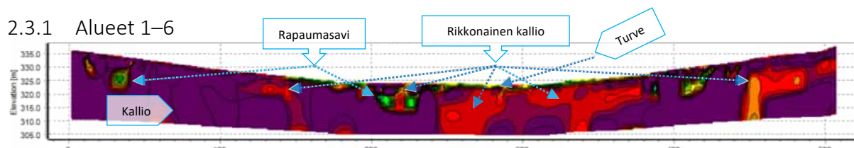
Kuva 3 Alue 1 -tulospystyleikkauskuvan X-akseli kuvaa maan päällä olevan mittauslinjan pituutta metreinä ja Y-akseli mittauksen syvyyttä metreinä. Mittauksen alkupisteen (kuvan vasen reuna) koordinaatit: 526763.1016 (X), 7379906.6713 (Y), 336,25 (Z). Mittauksen loppupisteen (kuvan oikea reuna) koordinaatit: 526666.7173 (X), 7380394.2412 (Y), 337,87 (Z).
