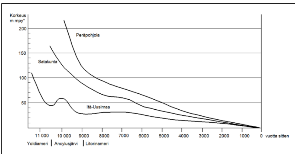
Kuva 5. Rannansiirtymiskäyriä eri puolilla Suomea. Itä-Uusimaan käyrässä näkyy selvänä kohoumana Ancylusjärven tulvavaihe noin 10 000 vuotta sitten ja matalampana Litorinameren pitkäaikaisempi, mutta vähäisempi tulvavaihe. (Kuva Åberg 2013, s. 15)
