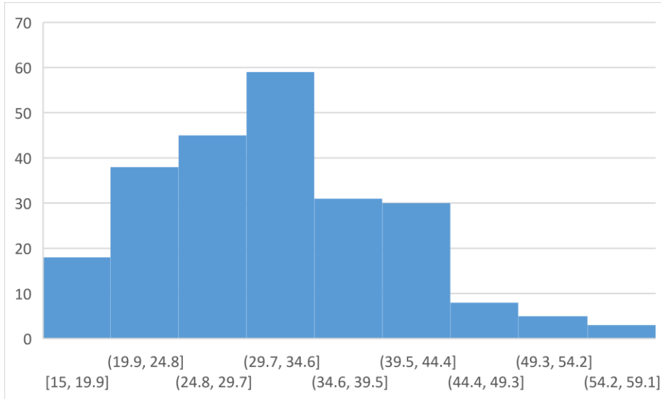
Kaavio 1. Kivikautisten asuinpaikkojen (238 kpl) sijaintikorkeuden alaraja otanta-alueella. Ainoa piikki on 29–35 metrin korkeudella mpy., mikä todennäköisesti johtuu Litorina-transgression aikaisesta pitemmästä rantavaiheesta. Kaikkiaan sijaintikorkeuden jakauma on melko tasainen korkeuksien 20–44 metrin välillä.
