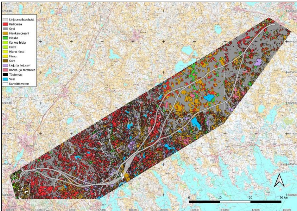
Kuva 2. Selvitysalueen maaperä. Länsiosa alueesta on pääosin savikoiden ympäröimiä kallioharjanteita ja itäosa puolestaan pääosin savea. Isompi versio kartasta karttaliitteissä. Lähde GTK:n Hakku-palvelu. (Isompi kartta, ks. karttaliite 8)
