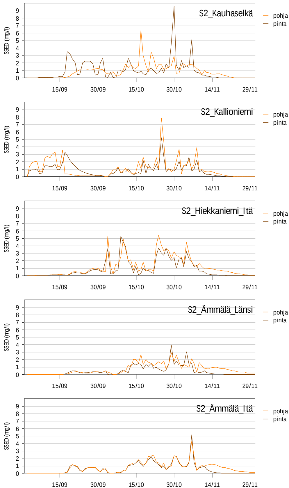
Kuva 10: Ruoppauksen aiheuttama kiintoainepitoisuuden nousu Kauhaselän eri pisteissä (vuorokauden keskipitoisuus).
