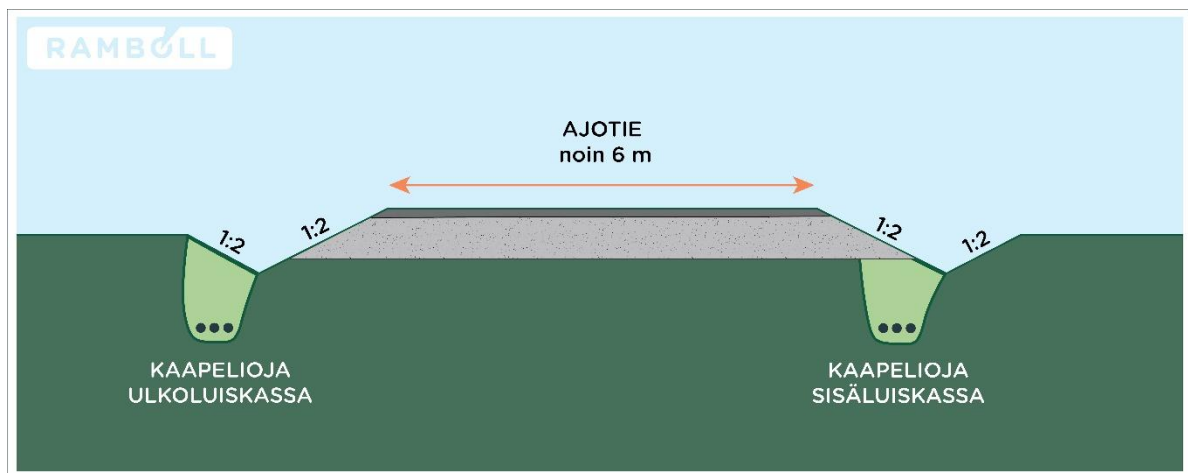
Kuva 9. Huoltotierakenteiden periaatepiirros.
