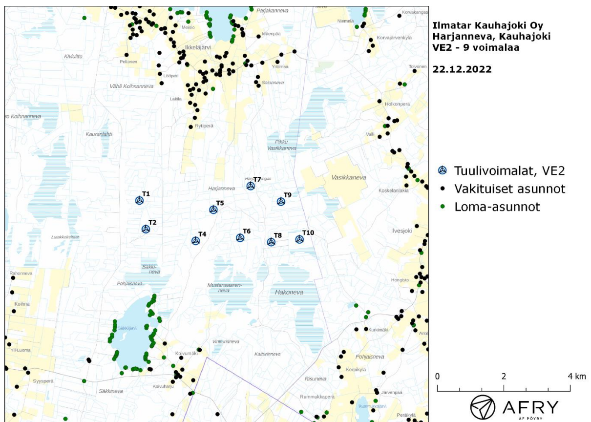
Kuva 1: Tuulivoimaloiden sijainnit Harjannevan hankealueella sijoitus suunnitelmalla VE2.
