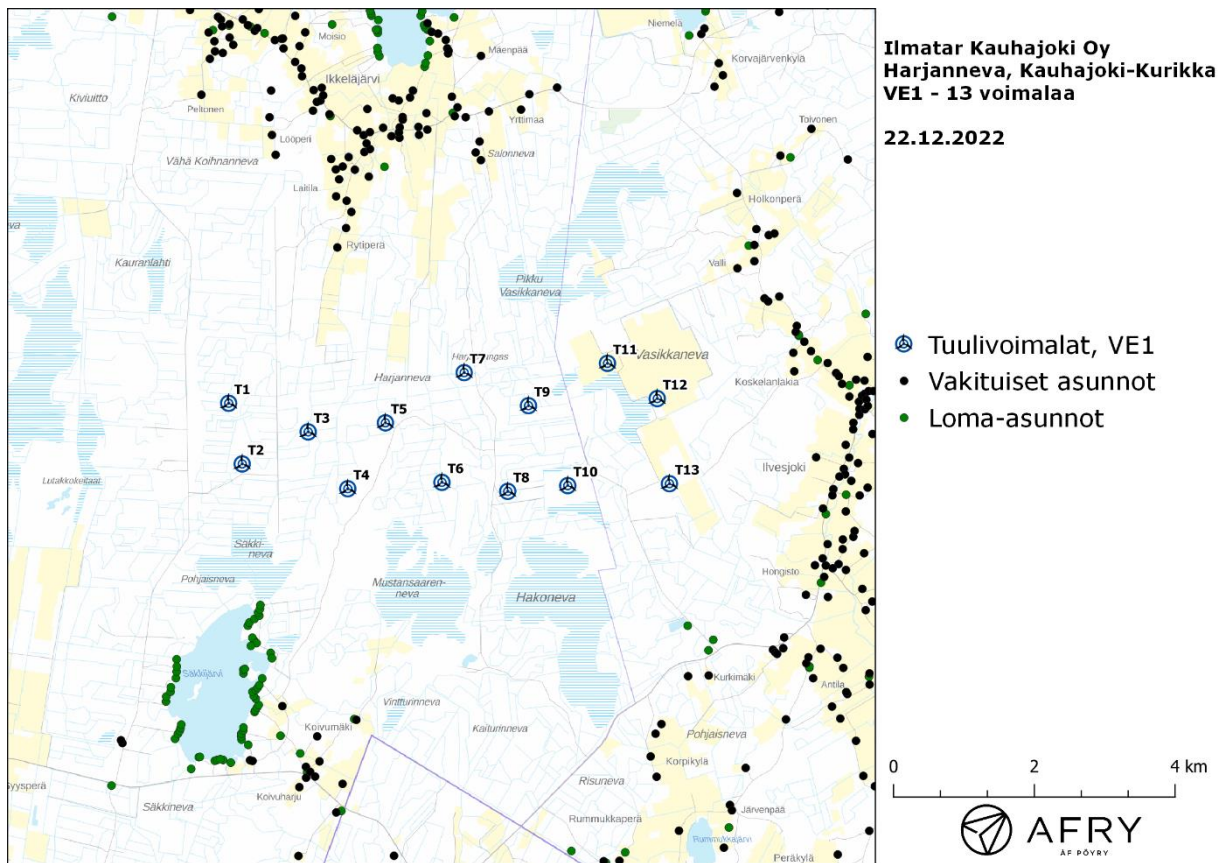
Kuva 1: Tuulivoimaloiden sijainnit Harjannevan hankealueella sijoitus suunnitelmalla VE1.
