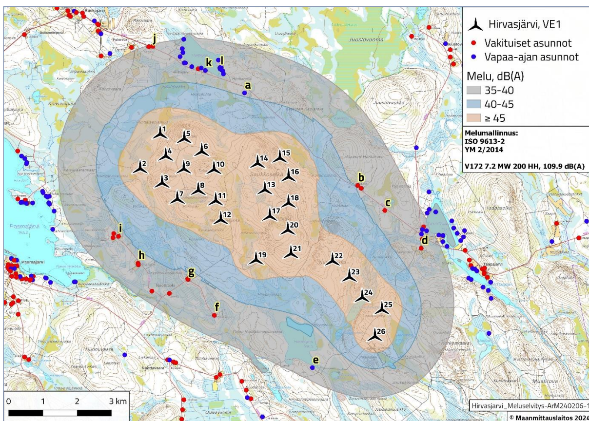
Kuva 1. Hirvasjärven tuulivoimapuiston melumallinnus (VE1). Kaksitoista havainnointipistettä on merkitty kuvaan kirjaimilla.
