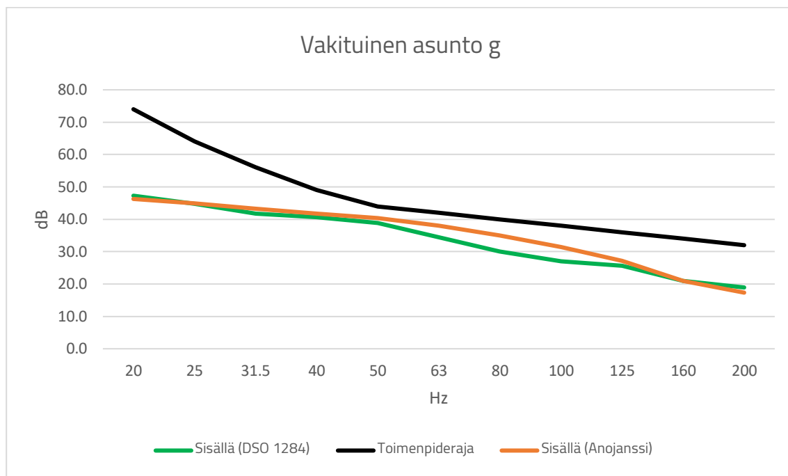
Kuva 4. Ympäristöministeriön ohjeistuksen mukainen pienitaajuisen melun laskenta sekä sosiaali- ja terveysministeriön toimenpiderajat vakituksessa asunnossa g.
