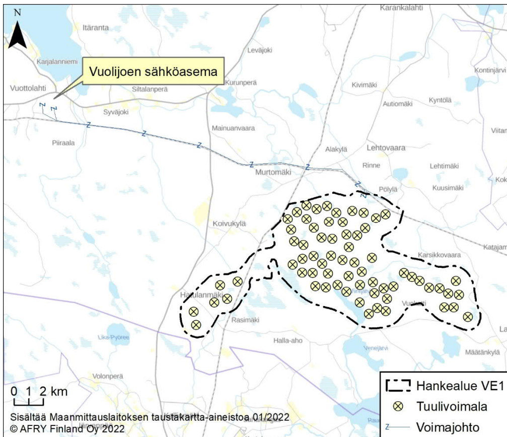
Kuva 3. Tuulipuiston sähkönsiirtoreitti.
