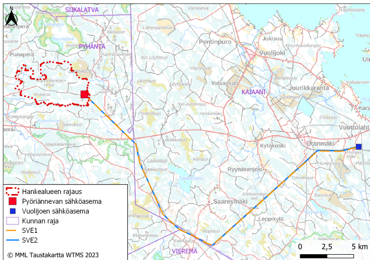
Kuva 3. Pyöriännevesin tuulivoimahankkeen suunniteltu sähkönsiirto
