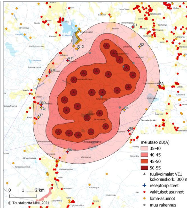
Kuva 1. Keskiäänitasot ( L_{Aeq} ) sijoitussuunnitelmassa VE1. Voimalan napakorkeus on joko 225 m, 190 m tai 165 m.
