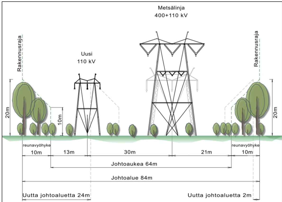
Kuva 5. Johtoalueen poikkileikkaus. Sähkösiihtoreitin SVEA ilmajohto sijoittuu Fingridin Metsälinja 400+110 kV voimajohdon pohjoispuolelle Hirsinevan Natura-alueen ja Metsälinjan väliin. Johtoaukean leveydeksi tulee yhteensä noin 64 metriä ja johtoalueen leveydeksi noin 84 metriä.
