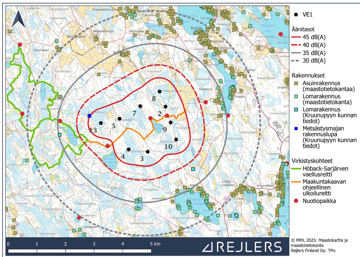
Kuva 2. Äänitasot hankealueella ja sen ympäristössä hankevaihtoehdossa VE1.
