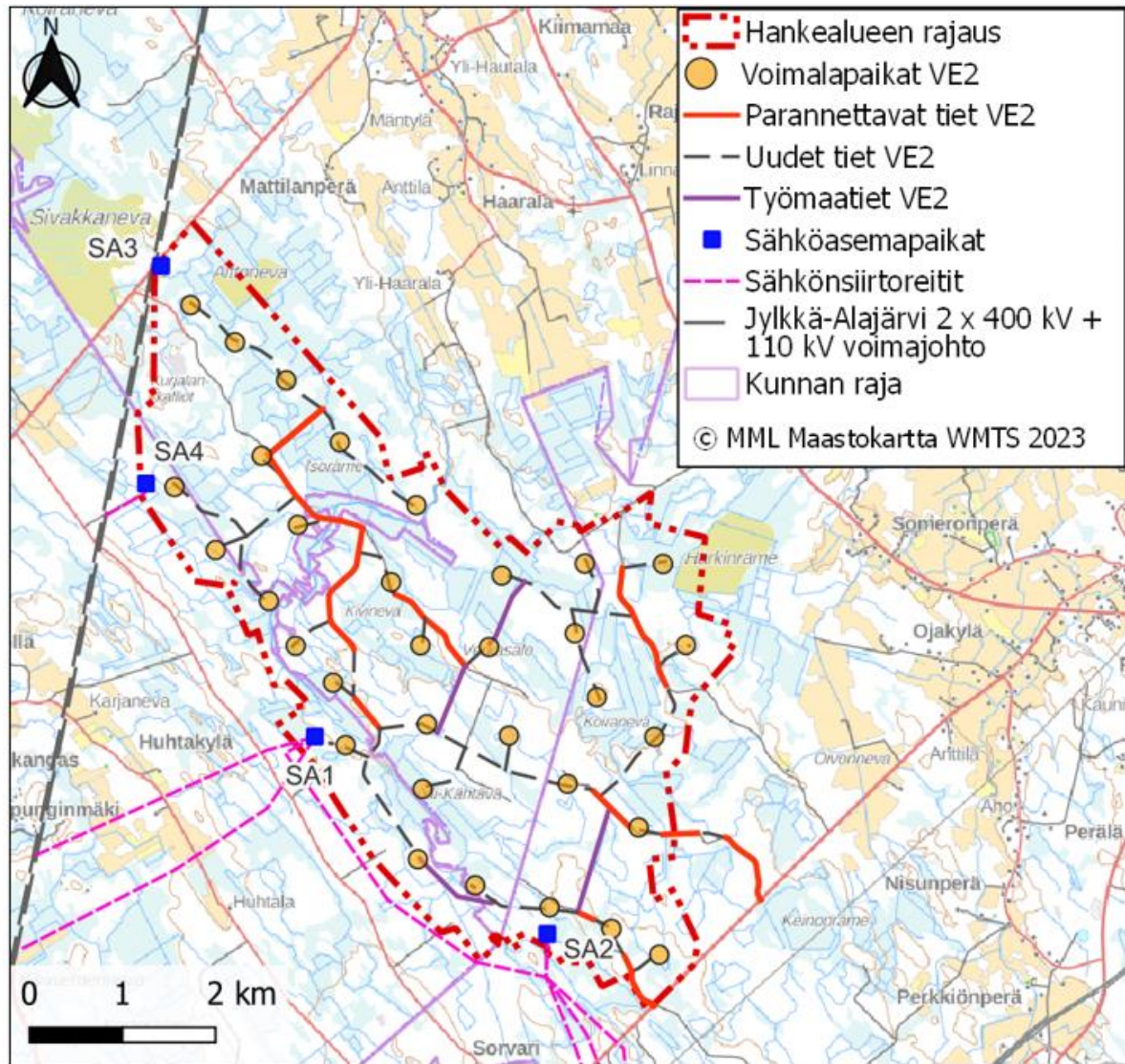
Kuva 3. Hankealueen raja ja tuulivoimaloiden sijainnit hankevaihtoehdossa VE2 (33 voimalaa). Suunnitelluista voimaloista sijaitsee 18 Alavieskan alueella, 9 Ylivieskan alueella ja 6 Kalajoen alueella.
