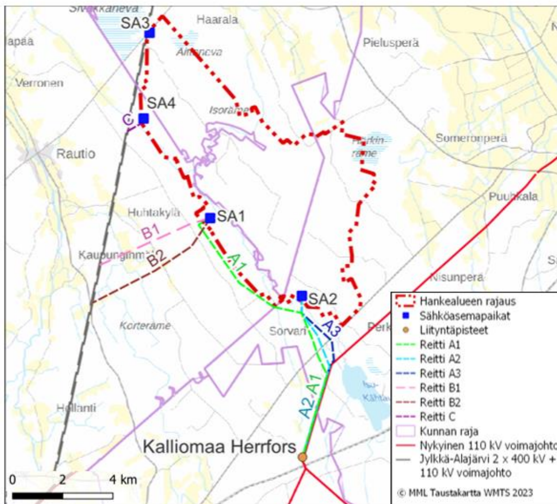
Kuva 4. Suunnitellut voimajohtoreittivaihtoehdot (SVEA, SVEB ja SVEC) alavaihtoehtoineen. Reittivaihtoehdossa SVED liitytään suoraan tuulivoimapaiston sähköasemalta SA3 Jylkkä-Alajärvi voimajohtoon.
