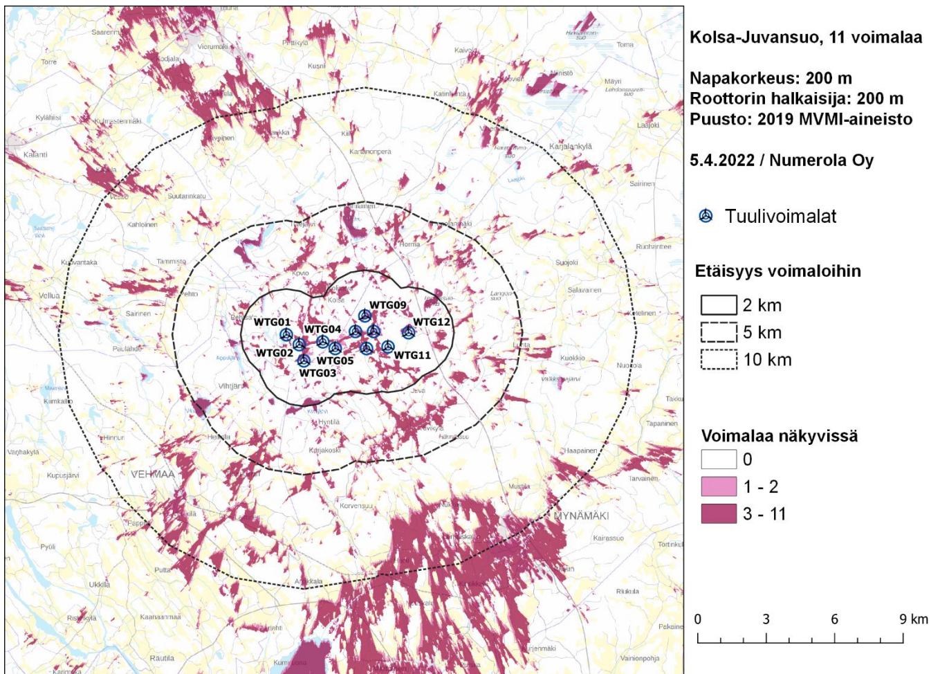
Kuva 3: Tuulivoimaloiden näkyminen 11 voimalan sijoitussuunnitelmalla.
