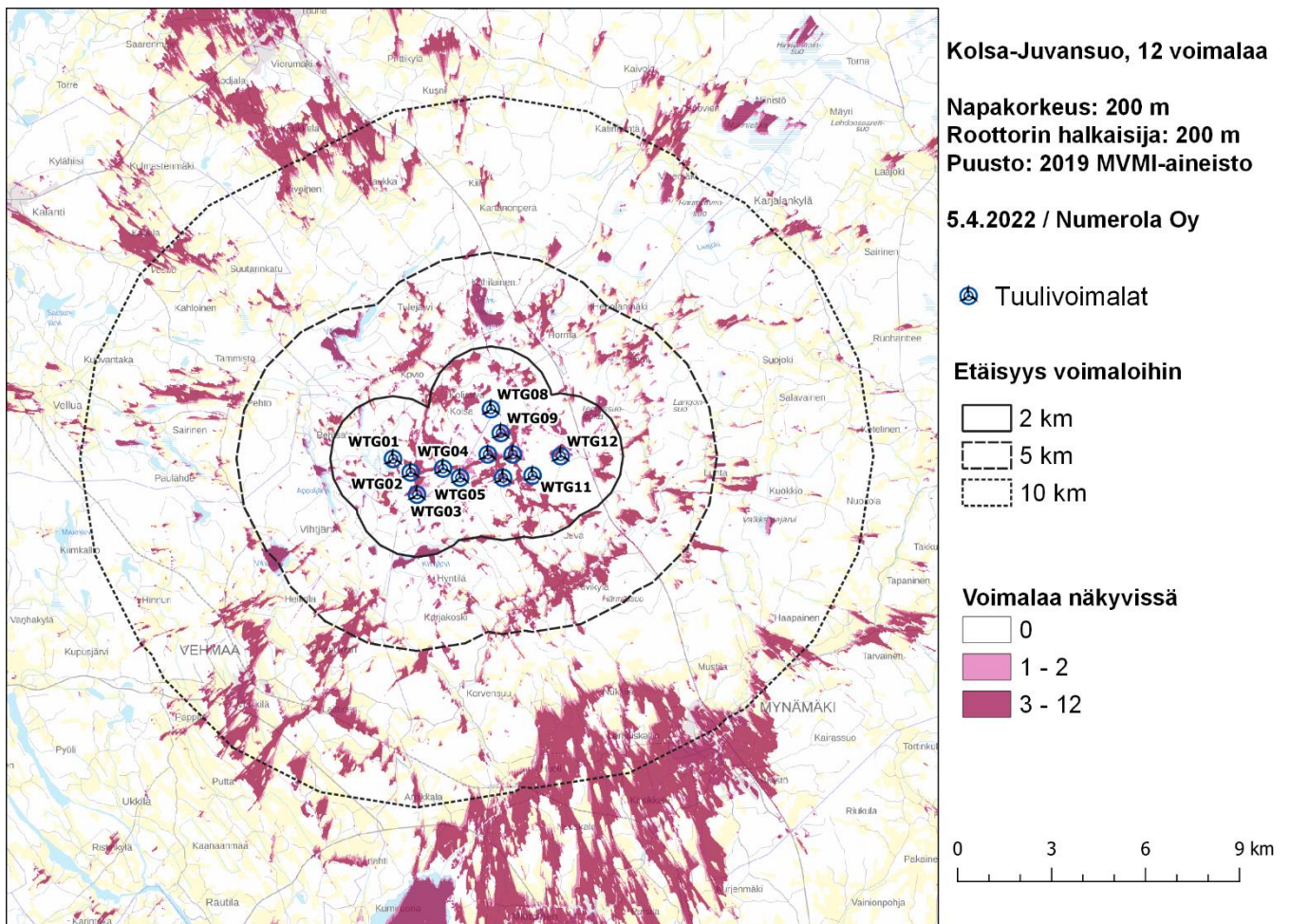
Kuva 2: Tuulivoimaloiden näkyminen 12 voimalan sijoitussuunnitelmalla.
