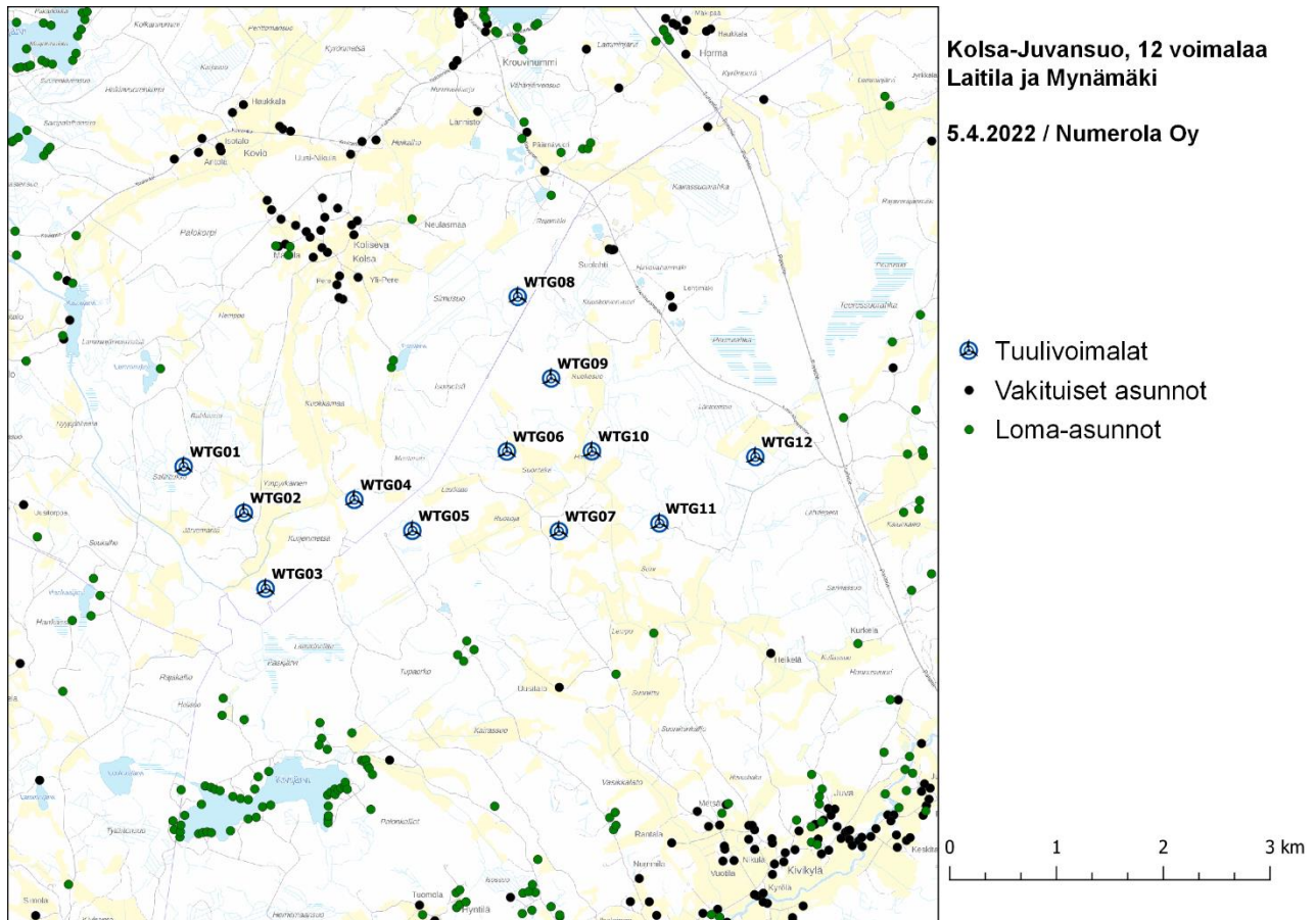
Kuva 1: Tuulivoimaloiden sijainnit Kolsa-Juvansuon tuulivoimapuiston 12 voimalan sijoitus suunnitelmalla. 11 voimalan sijoitus suunnitelmasta puuttuu voimala WTG08 ja muiden voimaloiden koordinaatit ovat samat molemmissa suunnitelmissa.
