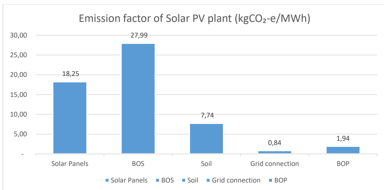
Kuvio 3 Aurinkovoimalan elinkaaren aikaiset päästökertoimet (kgCO 2 -e/MWh)
